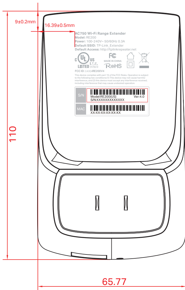
尺寸图
