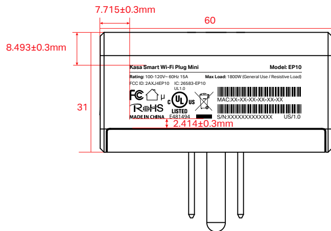
尺寸图
