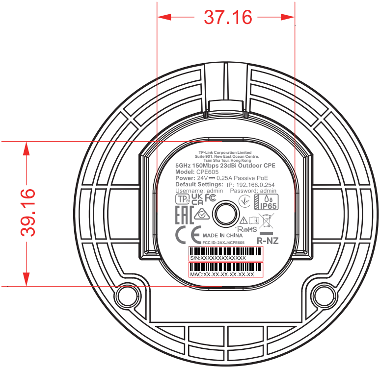
尺寸圖
