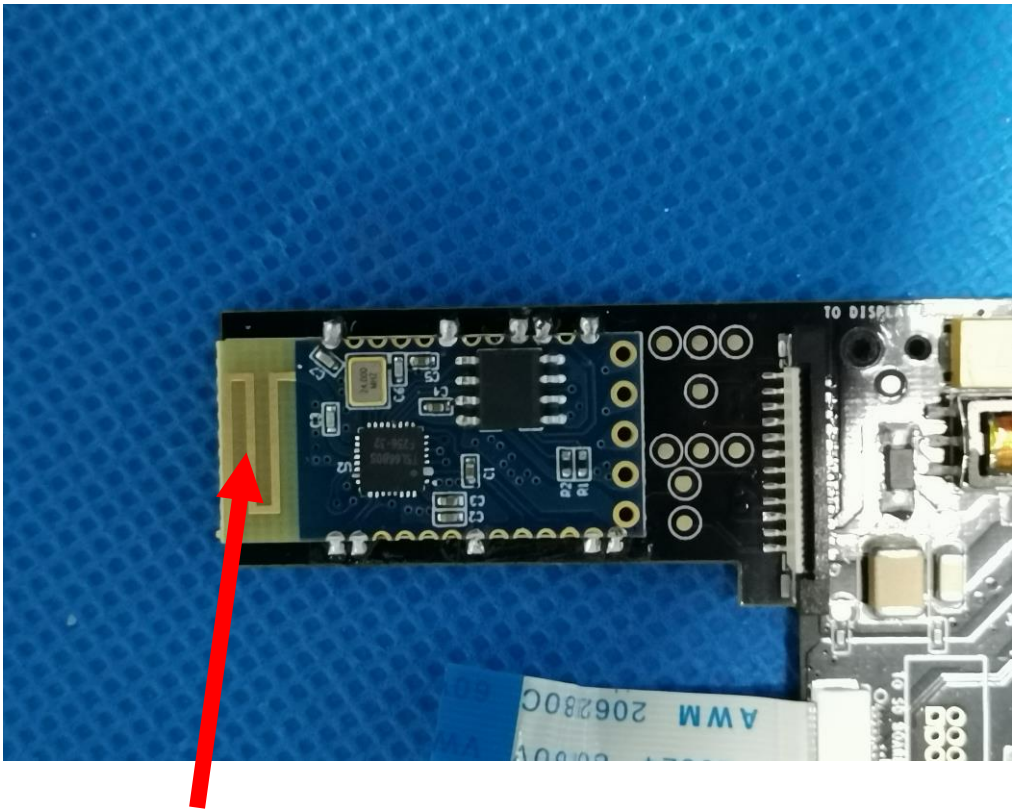
BT ANT
