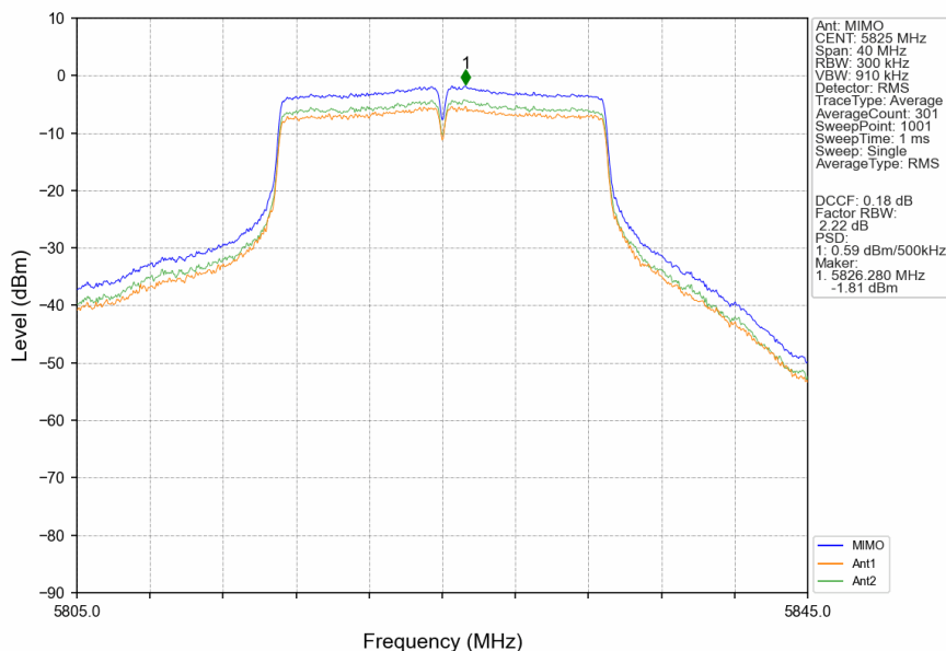
802.11n(HT20)_HCH_5825MHz_MIMO_NTNV
