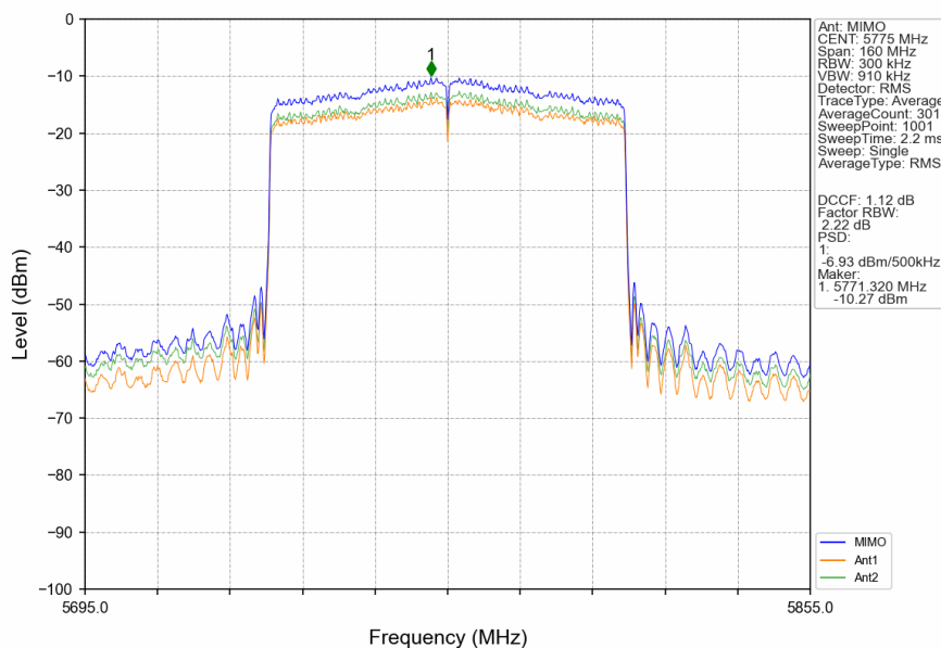
802.11ax(HEW80)_MCH_5775MHz_SU_ / _MIMO_NTNV
