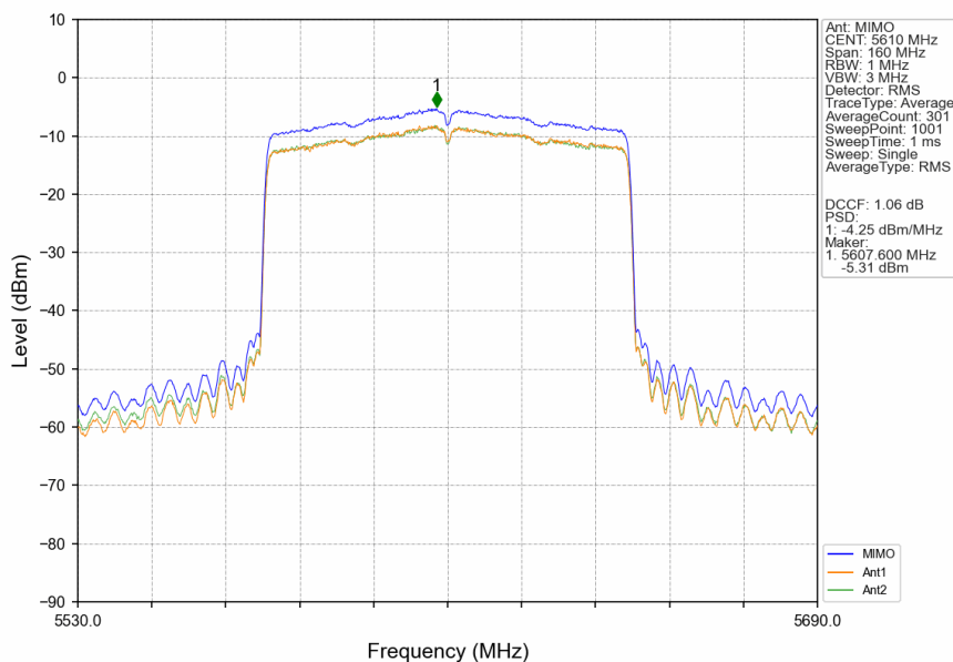
802.11ax(HEW80)_HCH_5610MHz_SU_ / _MIMO_NTNV
