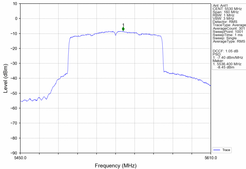
802.11ax(HEW80)_LCH_5530MHz_SU_ / _Ant1_NTNV
