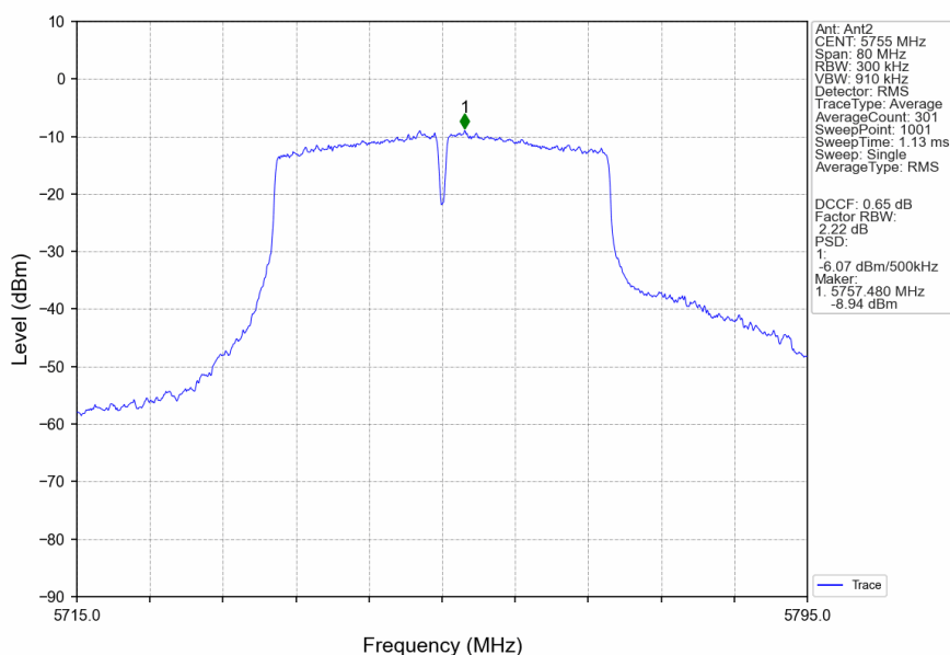
802.11n(HT40)_LCH_5755MHz_Ant2_NTNV
