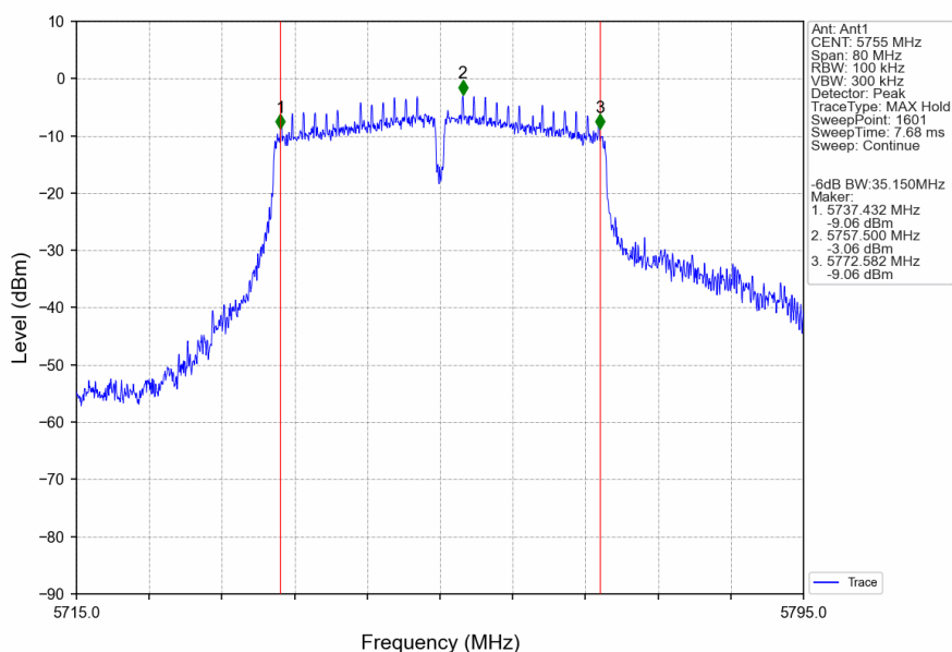
802.11n(HT40)_LCH_5755MHz_Ant1_NTNV
