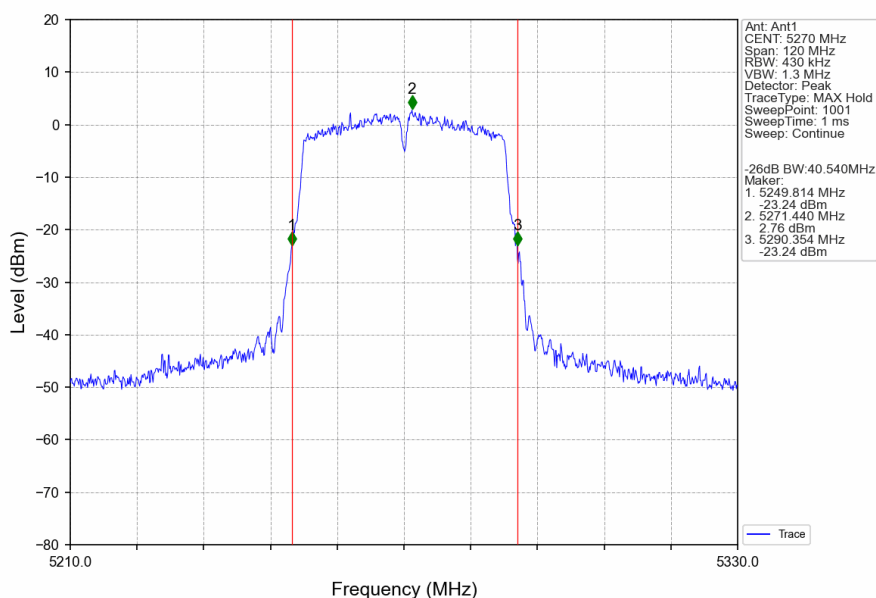
802.11n(HT40)_LCH_5270MHz_Ant1_NTNV
