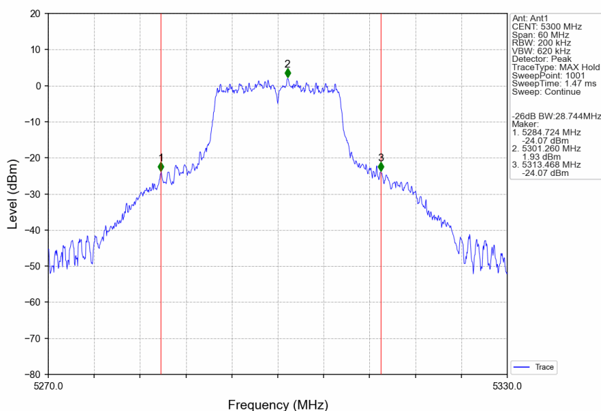
802.11a_MCH_5300MHz_Ant1_NTNV
