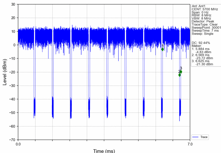
802.11ac(VHT20)_HCH_5700MHz_Ant1_NTNV
