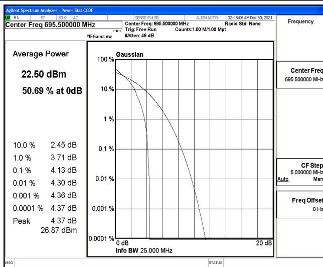
Band71-5MHz-QPSK-133447-25RB#0
