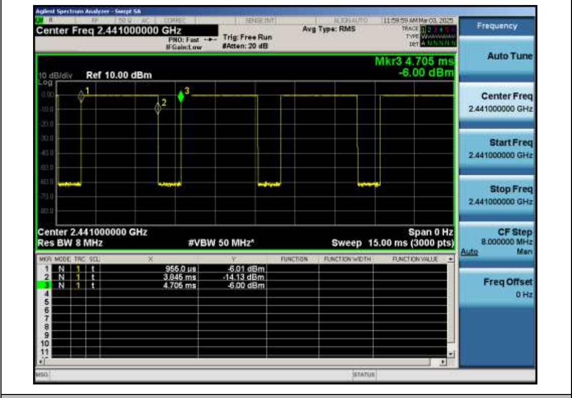
BR-GFSK-Ant1-2441
