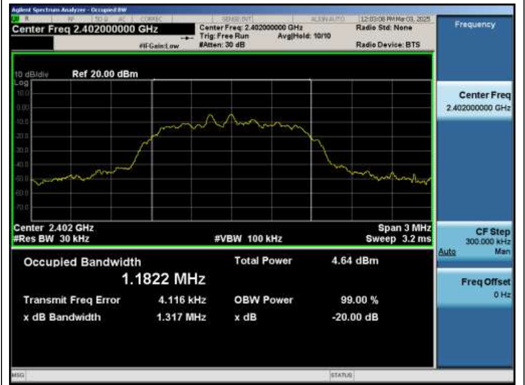
Test_Graph_EDR_ANT1_2402_2Mbps_OBW
