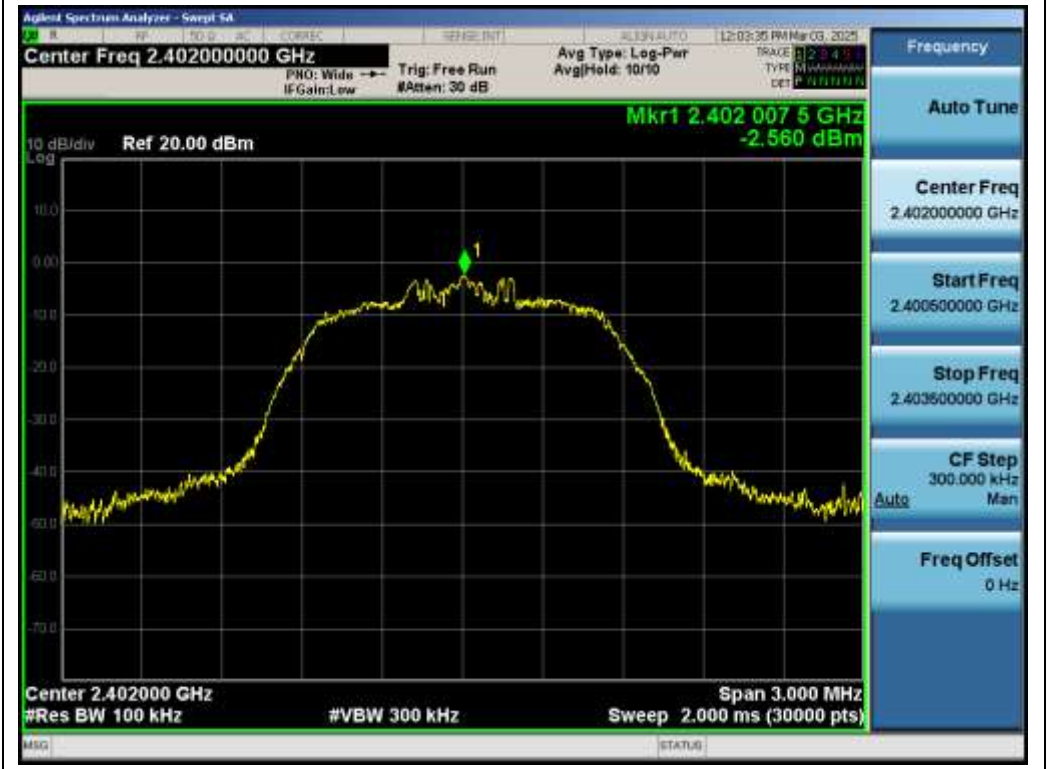
Test_Graph_EDR_ANT1_2402_2Mbps_Reference Level
