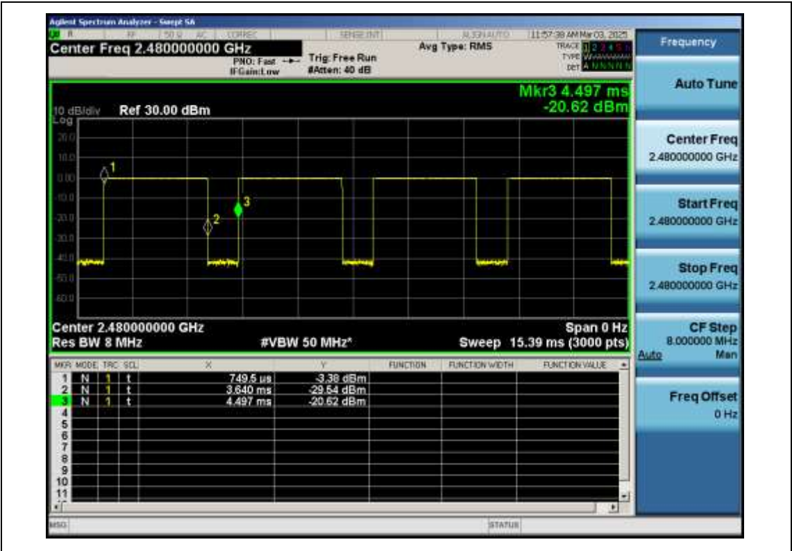
BR-GFSK-Ant1-2480
