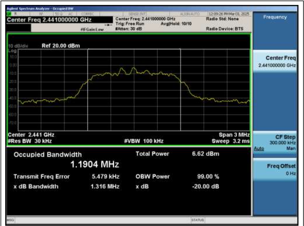
Test_Graph_EDR_ANT1_2441_2Mbps_OBW
