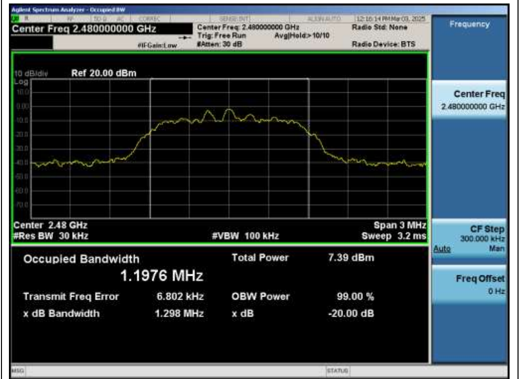
Test_Graph_EDR_ANT1_2480_2Mbps_OBW
