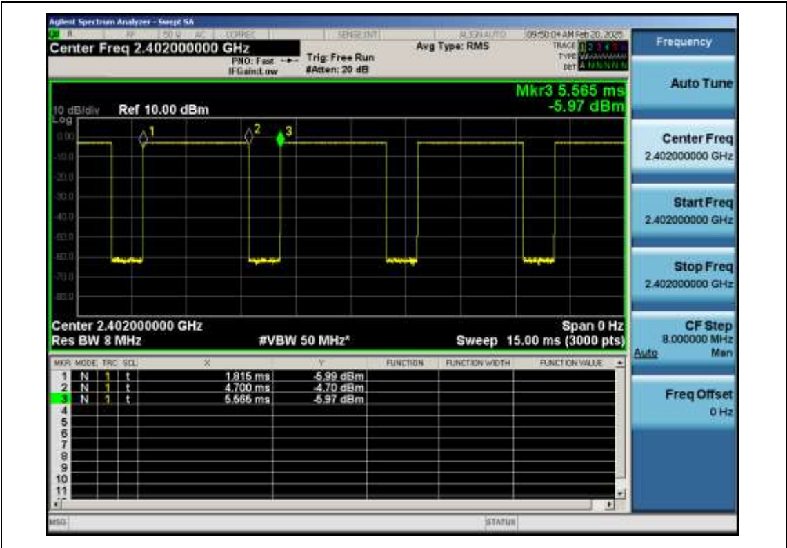
BR-GFSK-Ant1-2402
