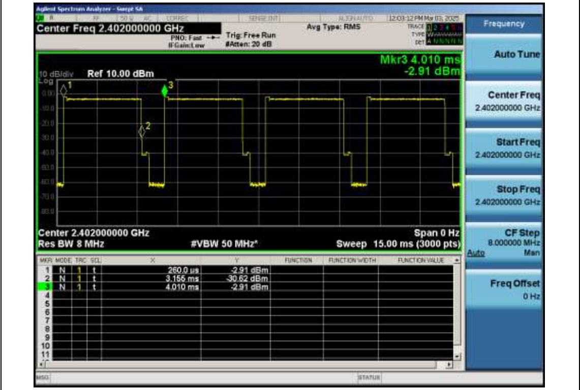
EDR- \pi/4 -DQPSK-Ant1-2402
