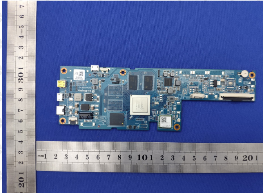
EUT Photo 3
