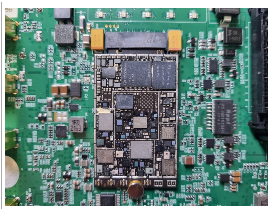
< 5G NR, LTE Module >
