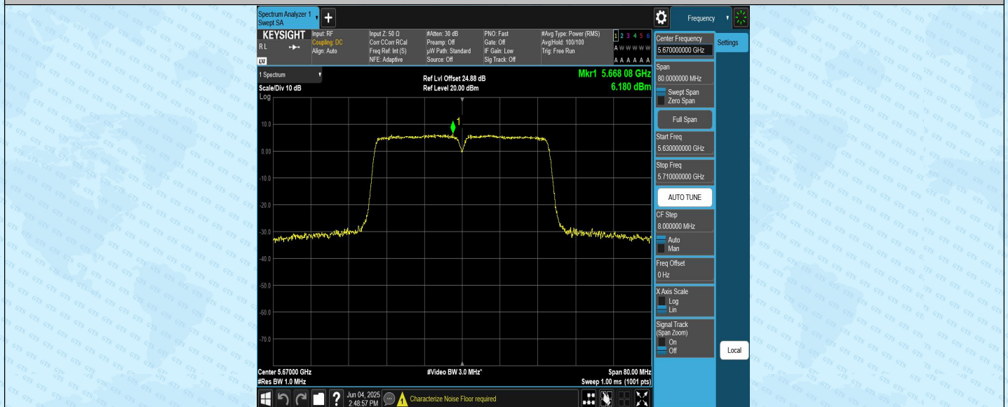
11N40CDD_Ant2_5670
