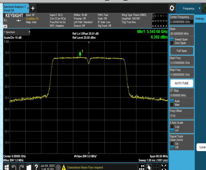
11N40CDD_Ant2_5550
