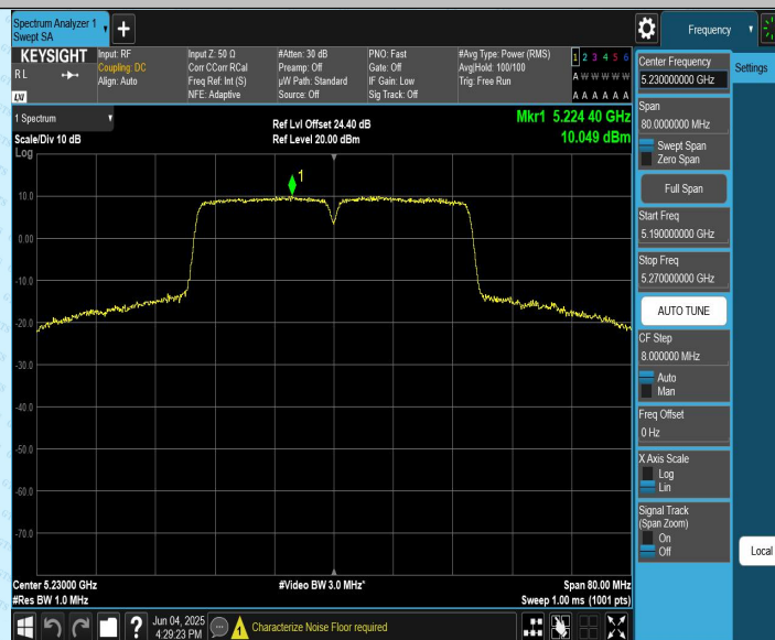
11AC40CDD_Ant2_5230
