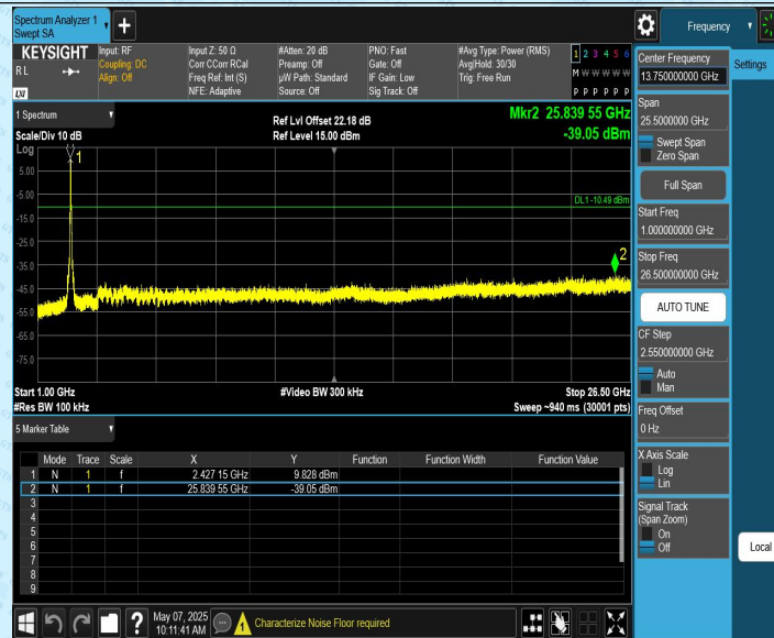
11N40CDD_Ant2_2422_0~Reference
