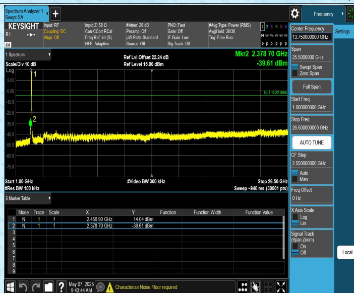
11N20CDD_Ant2_2462_0~Reference
