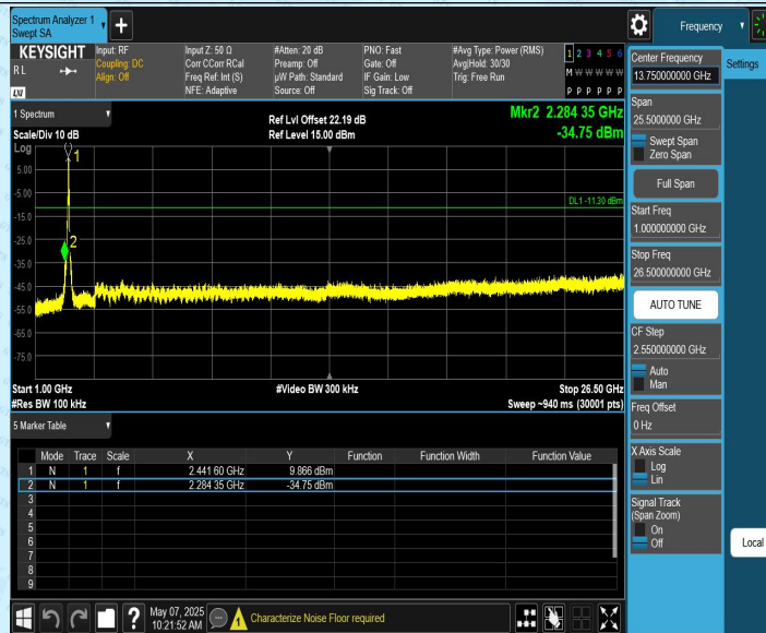
11N40CDD_Ant2_2437_0~Reference
