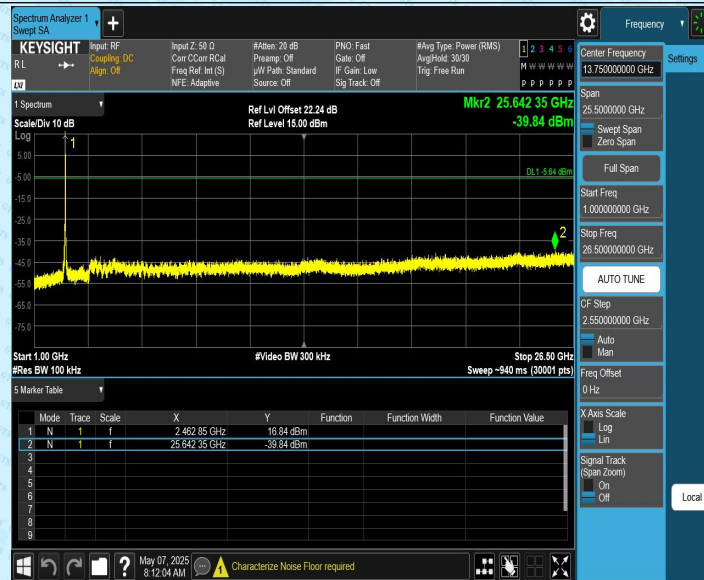
11B-CDD_Ant2_2462_0~Reference
