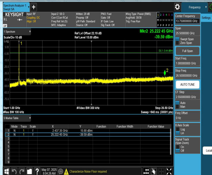
11B-CDD_Ant2_2437_0~Reference
