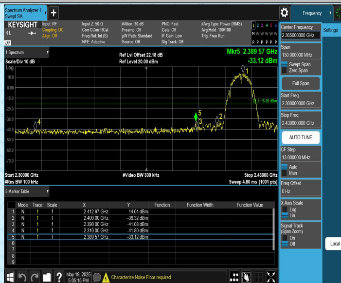
11B-CDD_Ant2_Low_2412
