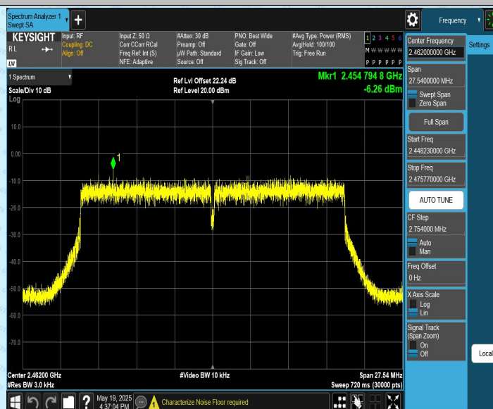
11AX20CDD_Ant2_2462
