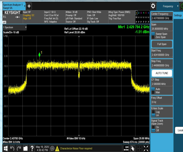
11AX20CDD_Ant2_2437
