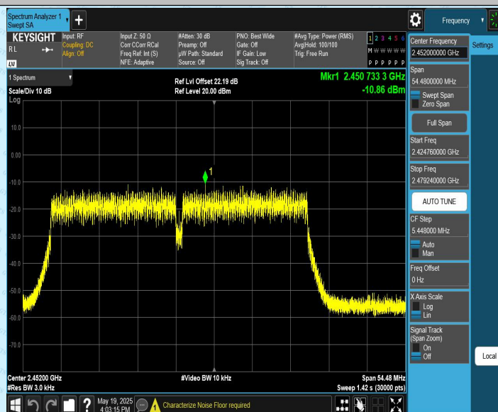
11N40CDD_Ant2_2452
