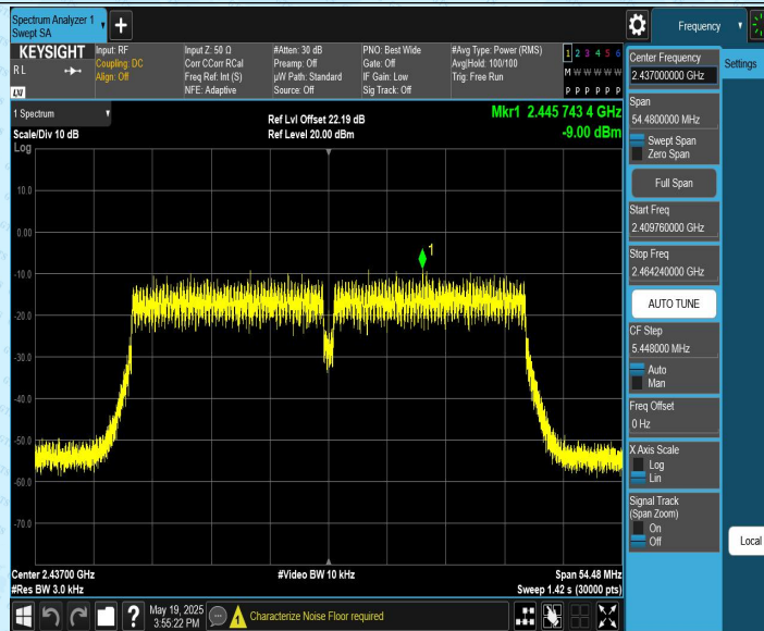
11N40CDD_Ant2_2437
