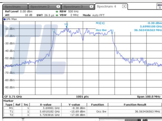
802.11n(HT40) - 5 710 MHz
