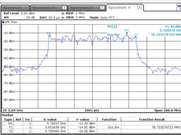
802.11ac(VHT80) - 5 690 MHz
