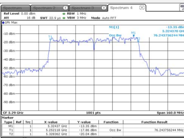
802.11ac(VHT80) - 5 290 MHz
