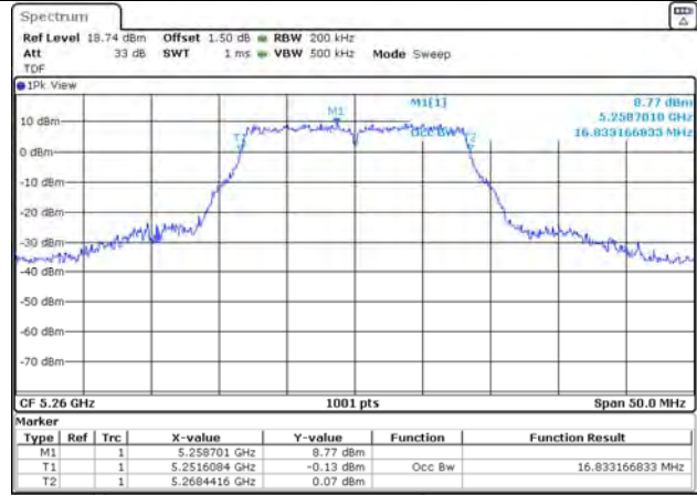
UNII-2A / 802.11a / 5 260 MHz
