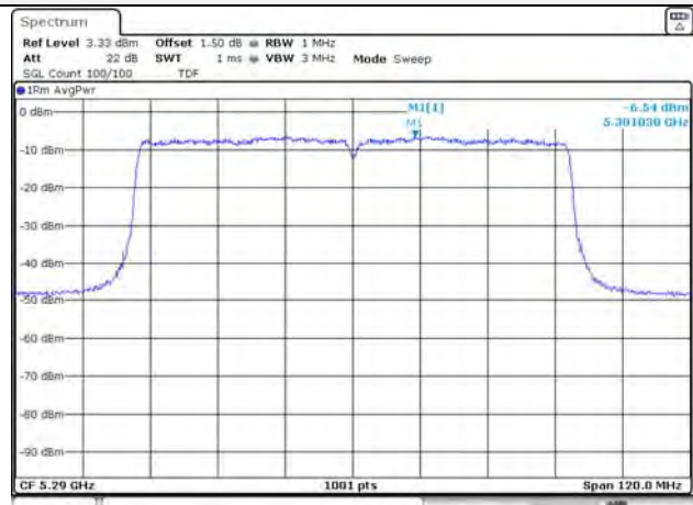
UNII-2A / 802.11ac VHT80 / 5 290 MHz
