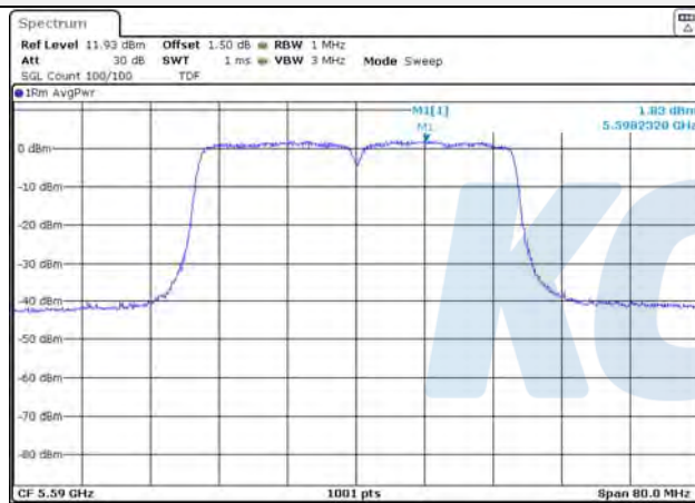
UNII-2C / 802.11ac VHT40 / 5 590 MHz
