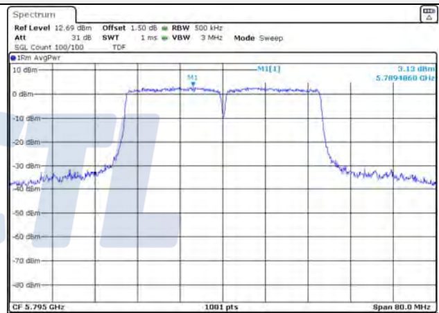
UNII-3 / 802.11ac VHT40 / 5 795 MHz
