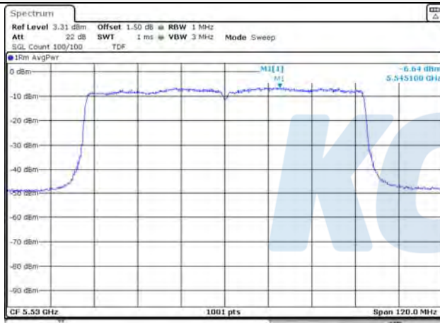
UNII-2C / 802.11ac VHT80 / 5 530 MHz
