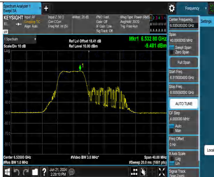
11BE20MIMO Ant4 6535 52+26 OFDMA 1
