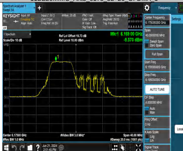
11BE20MIMO Ant4 6175 52+26 OFDMA 1
