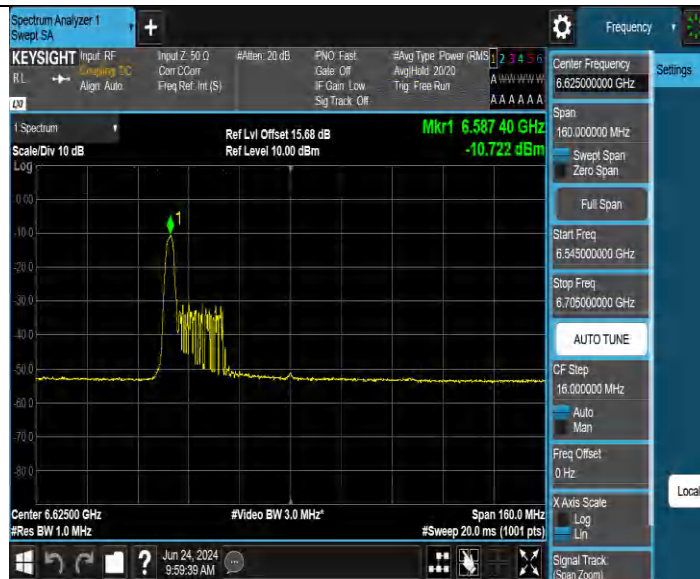
11BE80MIMO_Ant3 6625 26Tone RU0
