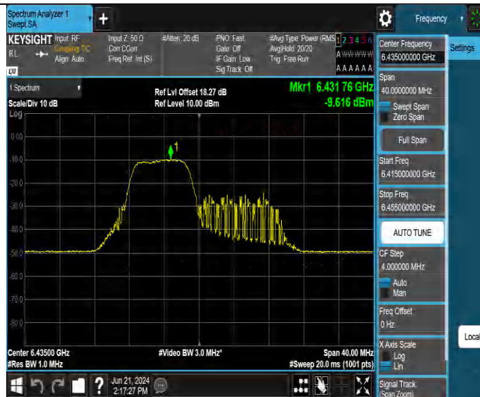
11BE20MIMO Ant4 6435 52+26 OFDMA 1
