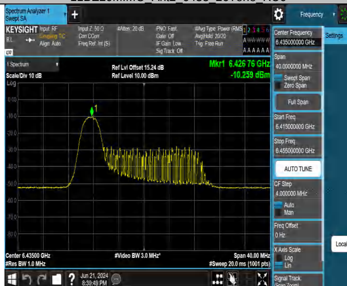
11BE20MIMO_Ant3_6435_26Tone_RU0
