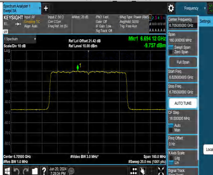
11BE80MIMO_Ant4_6705
