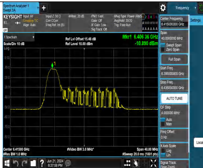
11BE20MIMO_Ant2 6415 26Tone RU0
