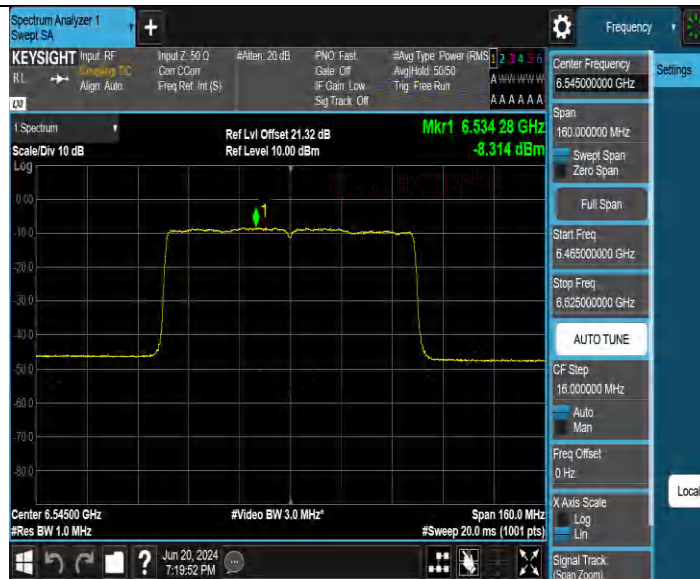
11BE80MIMO_Ant2 6545
