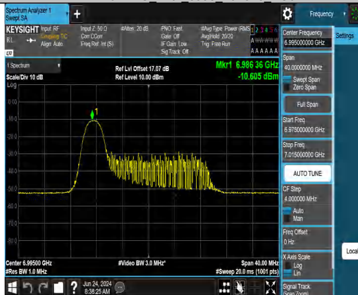
11BE20MIMO_Ant3_6995_26Tone_RU0
