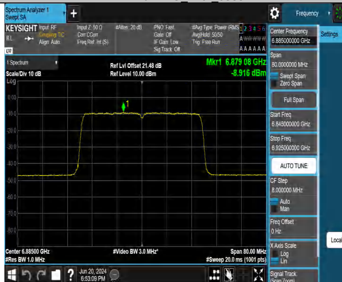
11BE40MIMO_Ant2 6885
