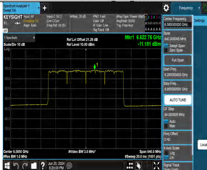
11BE320MIMO Ant3 6585
