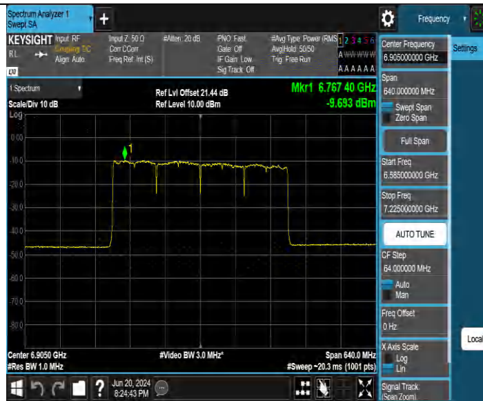
11BE320MIMO Ant4 6905
