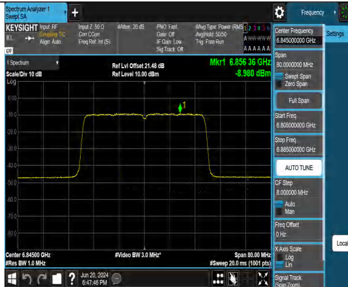
11BE40MIMO_Ant2 6845
