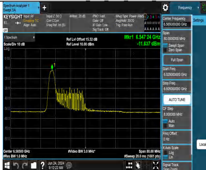
11BE40MIMO_Ant2 6565 26Tone RU0
