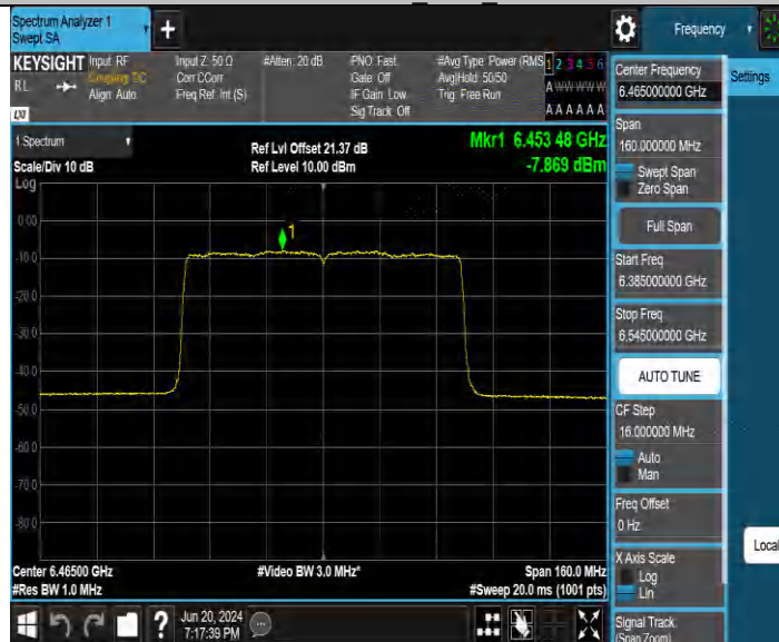
11BE80MIMO_Ant2 6465
