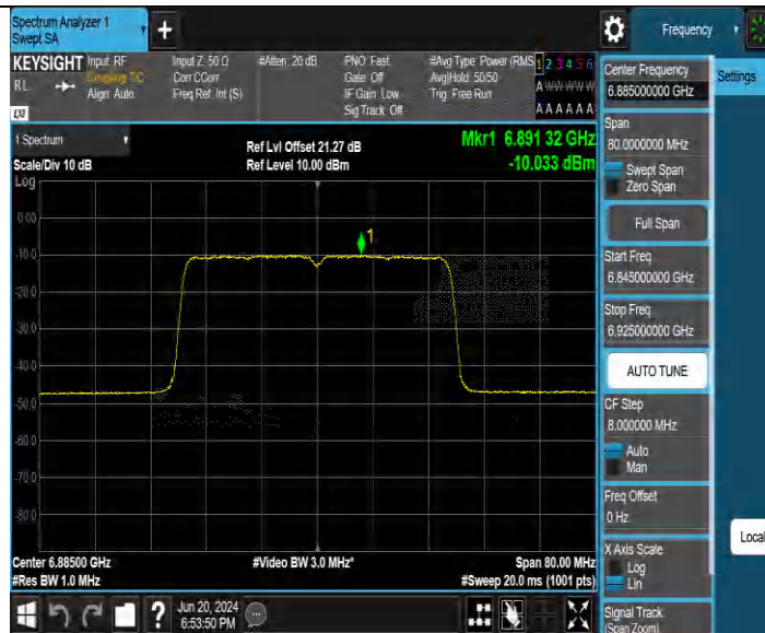
11BE40MIMO_Ant4 6885
