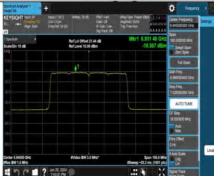
11BE80MIMO_Ant4_6945
