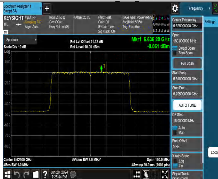
11BE80MIMO_Ant2_6625
