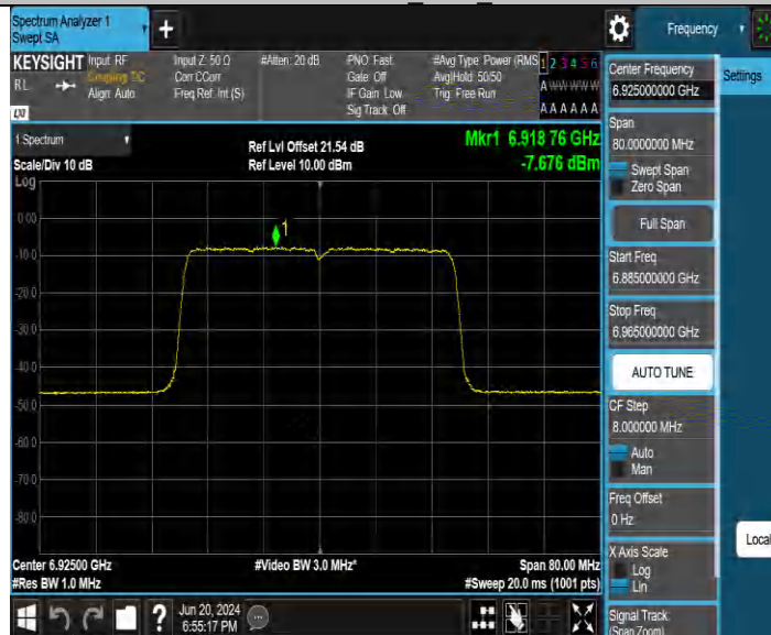
11BE40MIMO_Ant2 6925
