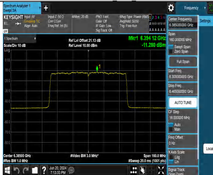
11BE80MIMO_Ant3_6385
