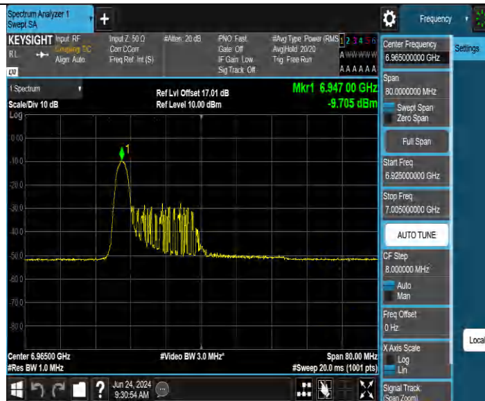
11BE40MIMO_Ant4 6965 26Tone RU0
