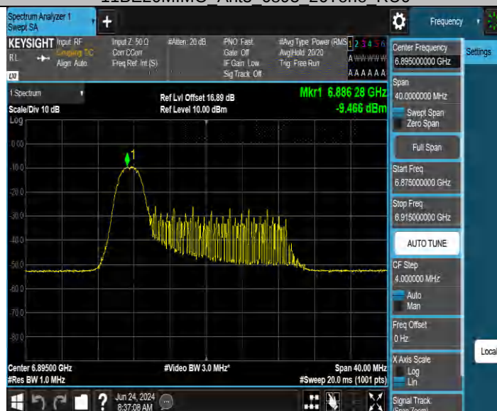
11BE20MIMO_Ant4 6895 26Tone RU0
