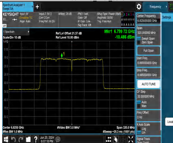
11BE160MIMO Ant3 6825
