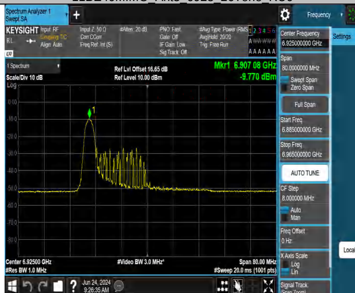
11BE40MIMO_Ant4 6925 26Tone RU0
