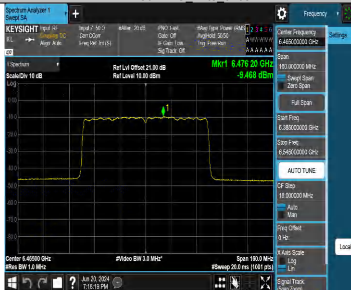
11BE80MIMO_Ant4_6465
