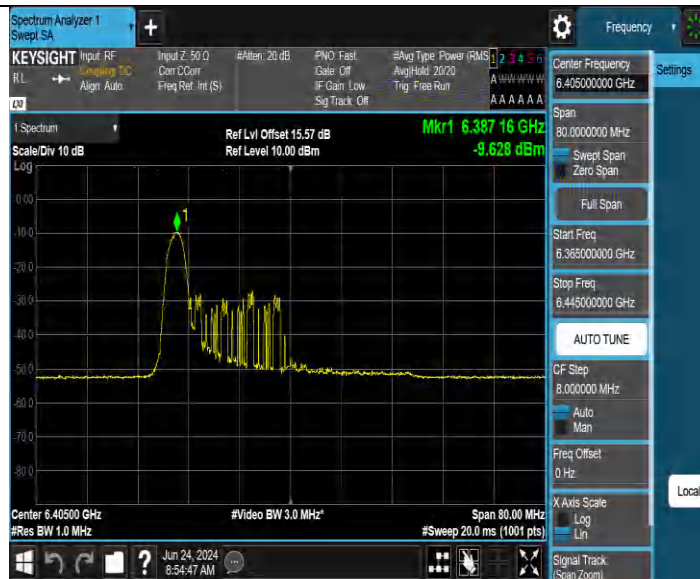
11BE40MIMO_Ant4 6405 26Tone RU0
