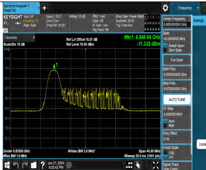
11BE20MIMO_Ant2_6855_26Tone_RU0
