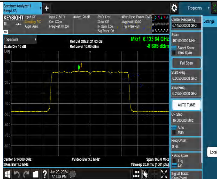
11BE80MIMO_Ant4 6145
