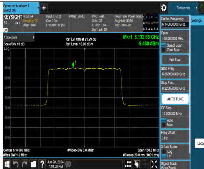
11BE80MIMO_Ant2 6145
