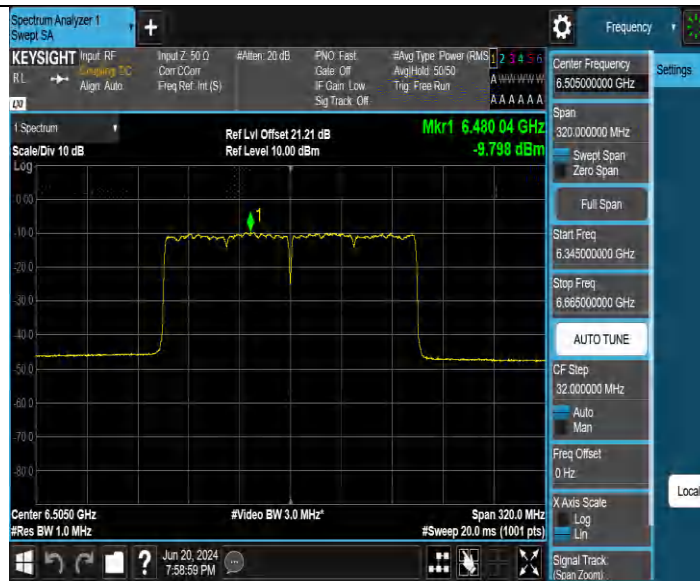
11BE160MIMO Ant4 6505
