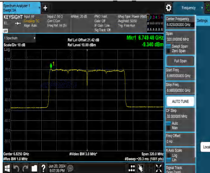
11BE160MIMO Ant4 6825
