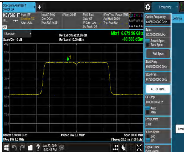
11BE40MIMO_Ant3_6685
