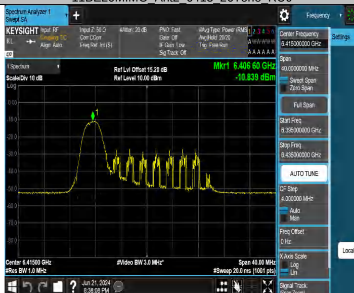
11BE20MIMO_Ant3 6415 26Tone RU0
