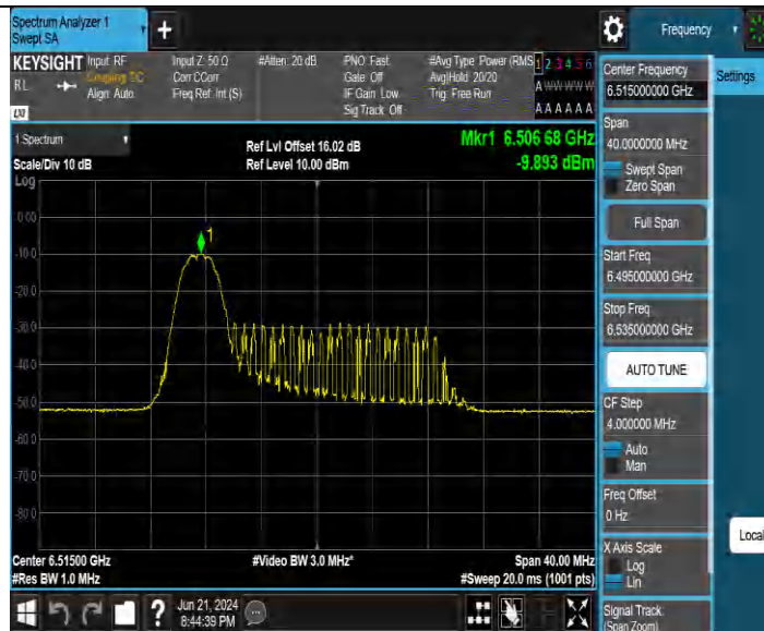
11BE20MIMO_Ant2_6515_26Tone_RU0
