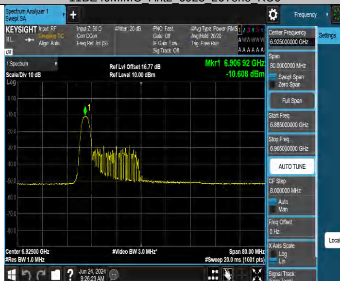
11BE40MIMO_Ant3 6925 26Tone RU0
