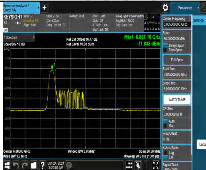
11BE40MIMO_Ant2 6885 26Tone RU0
