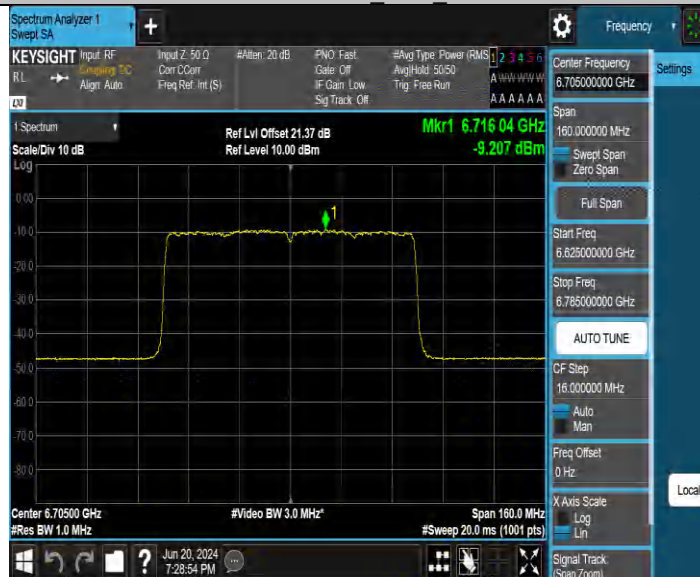
11BE80MIMO_Ant2 6705
