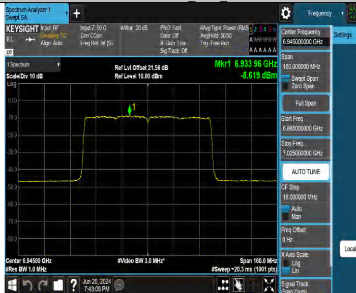
11BE80MIMO_Ant2_6945
