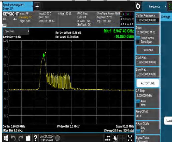
11BE40MIMO_Ant2 5965 26Tone RU0
