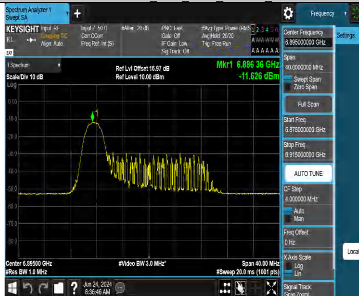
11BE20MIMO_Ant2 6895 26Tone RU0
