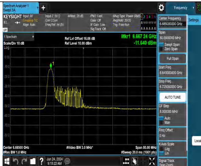
11BE40MIMO_Ant2_6685_26Tone_RU0
