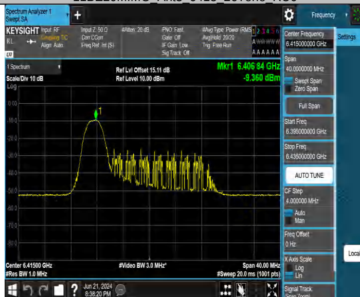
11BE20MIMO_Ant4 6415 26Tone RU0
