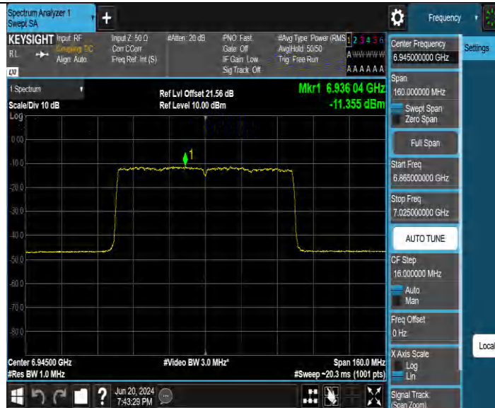
11BE80MIMO_Ant3_6945
