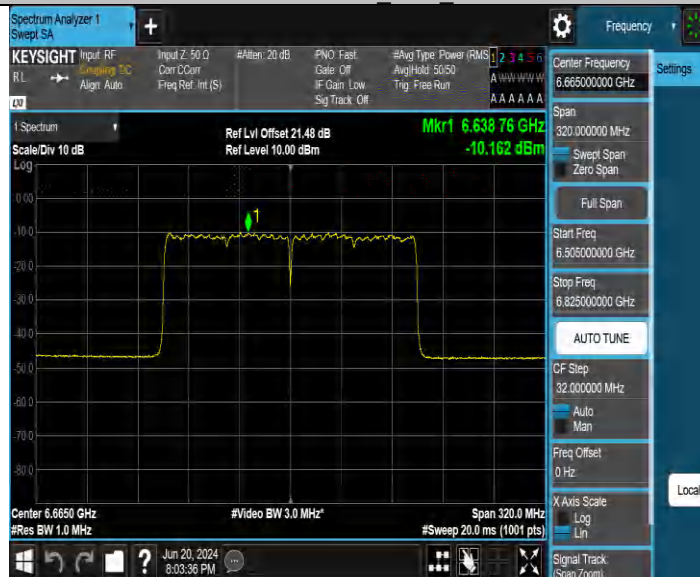
11BE160MIMO Ant1 6825
