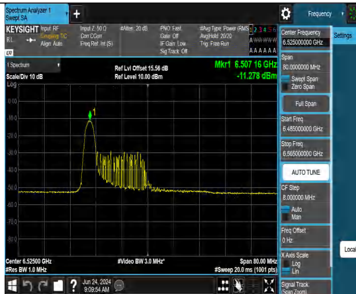
11BE40MIMO_Ant4 6525 26Tone RU0
