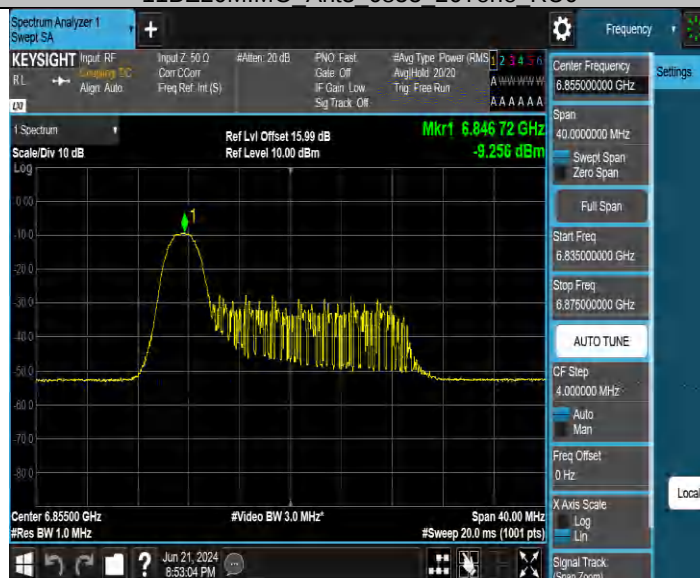
11BE20MIMO_Ant4_6855_26Tone_RU0
