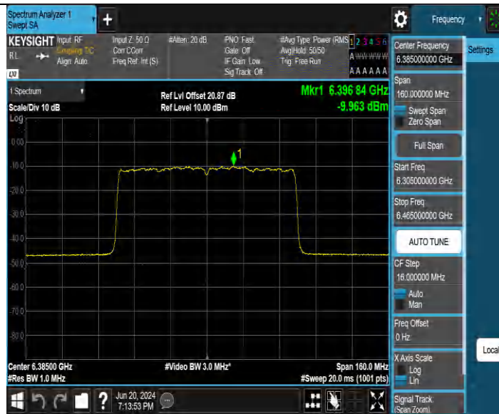
11BE80MIMO_Ant4 6385
