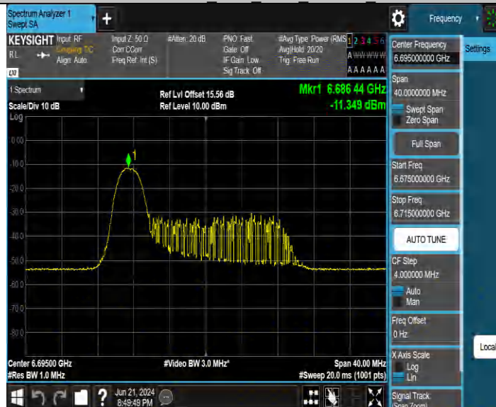
11BE20MIMO_Ant2 6695 26Tone RU0
