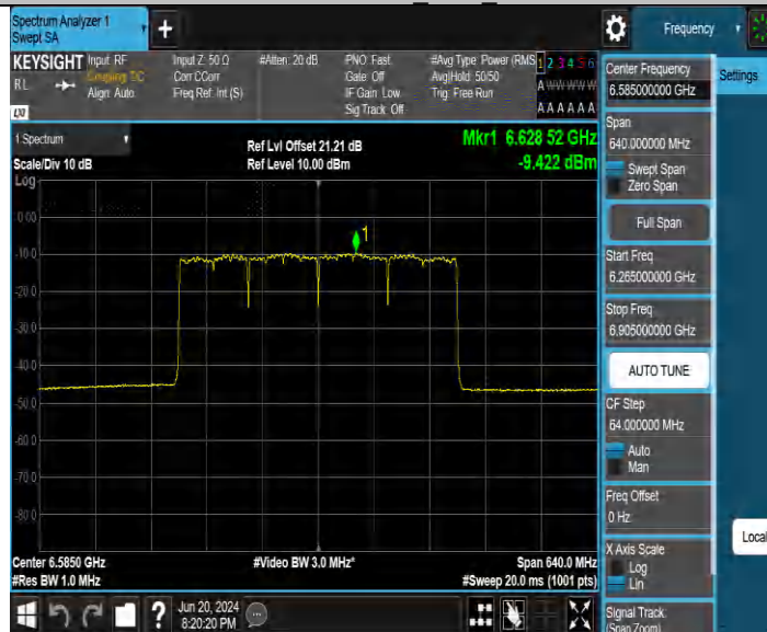
11BE320MIMO Ant4 6585
