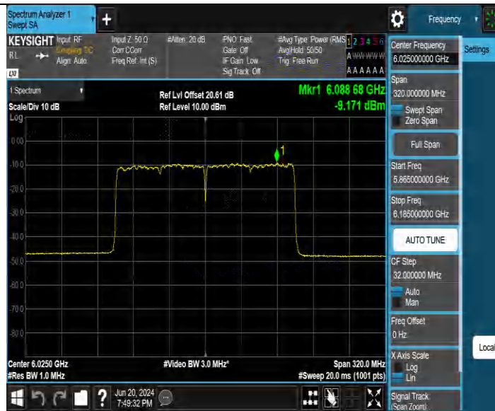
11BE160MIMO Ant4 6025
