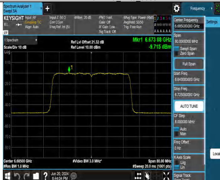
11BE40MIMO_Ant4_6685
