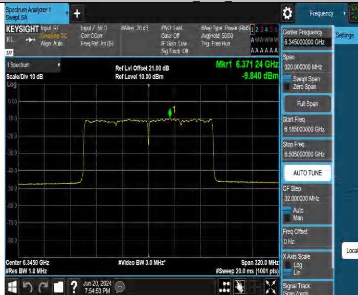
11BE160MIMO Ant4 6345
