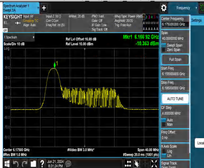
11BE20MIMO_Ant4 6175 26Tone RU0
