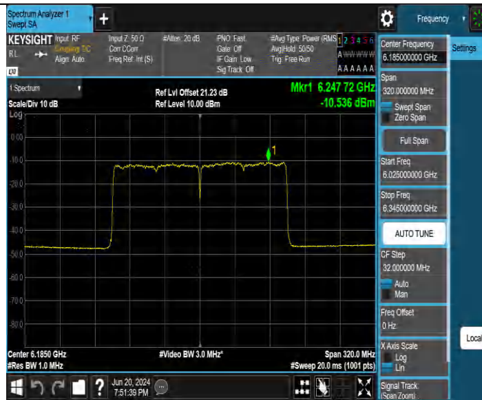
11BE160MIMO Ant3 6185
