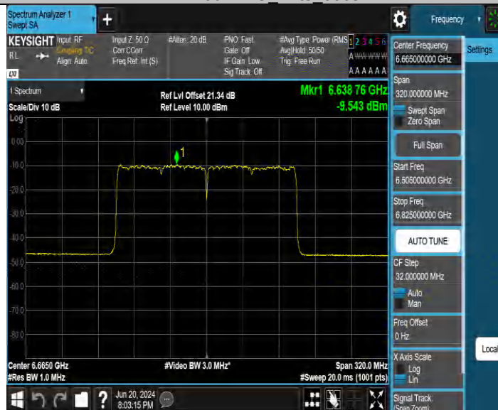
11BE160MIMO Ant4 6665
