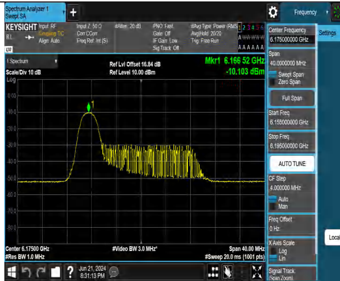
11BE20MIMO_Ant3 6175 26Tone RU0
