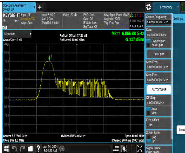
11BE20MIMO_Ant4 6875 26Tone RU0
