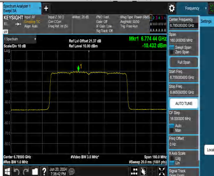
11BE80MIMO_Ant3 6785
