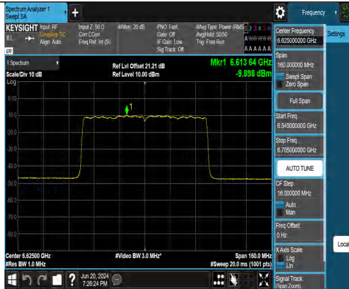
11BE80MIMO_Ant4 6625
