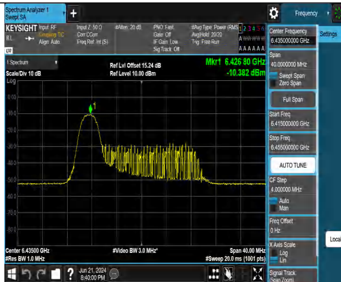
11BE20MIMO Ant4 6435 26Tone RU0
