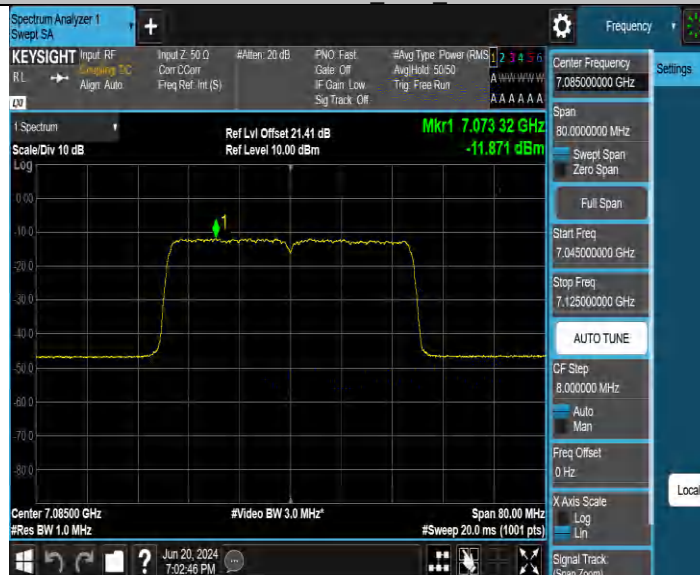
11BE40MIMO_Ant3_7085
