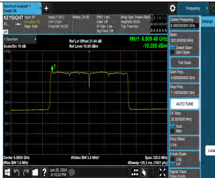
11BE160MIMO Ant4 6985
