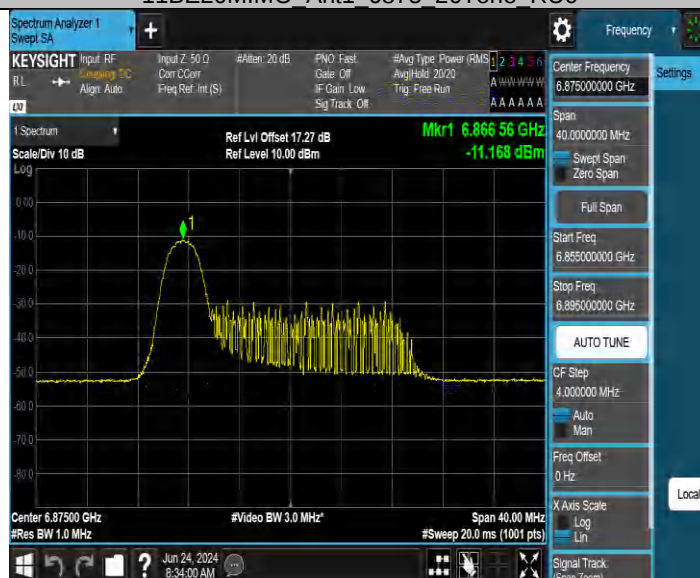
11BE20MIMO_Ant2_6875_26Tone_RU0
