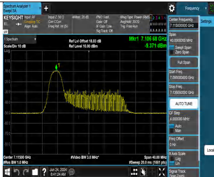
11BE20MIMO_Ant4 7115 26Tone RU0
