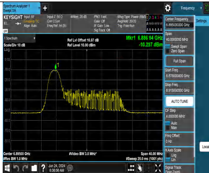
11BE20MIMO_Ant3 6895 26Tone RU0
