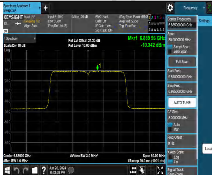
11BE40MIMO_Ant3 6885
