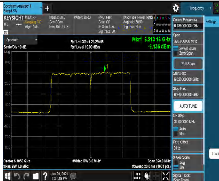
11BE160MIMO Ant2 6185
