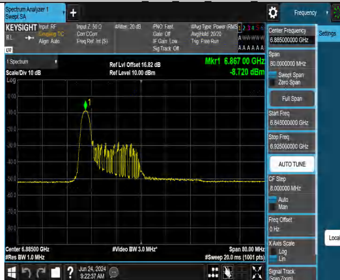
11BE40MIMO_Ant1 6925 26Tone RU0
