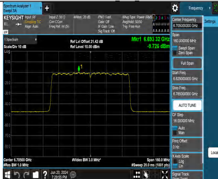
11BE80MIMO_Ant1_6785
