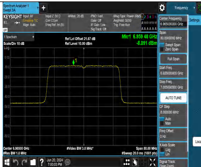
11BE40MIMO_Ant2_6965
