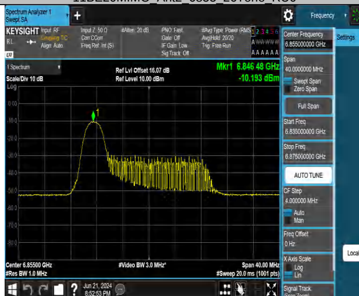
11BE20MIMO_Ant3_6855_26Tone_RU0
