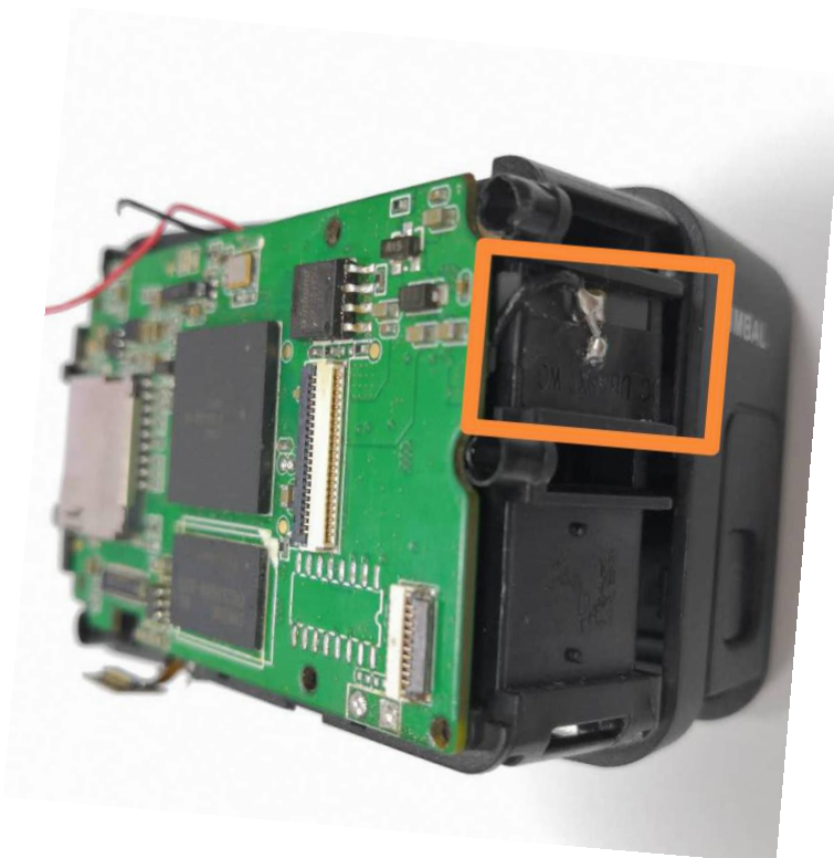
ANTENNA
