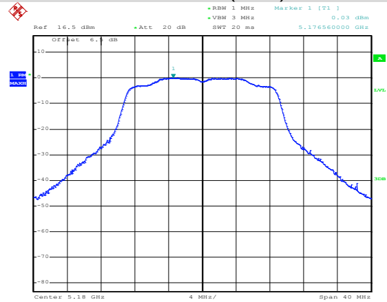
ANT2 802.11n(HT20)
