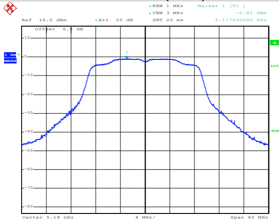
ANT1 802.11n(HT20)
