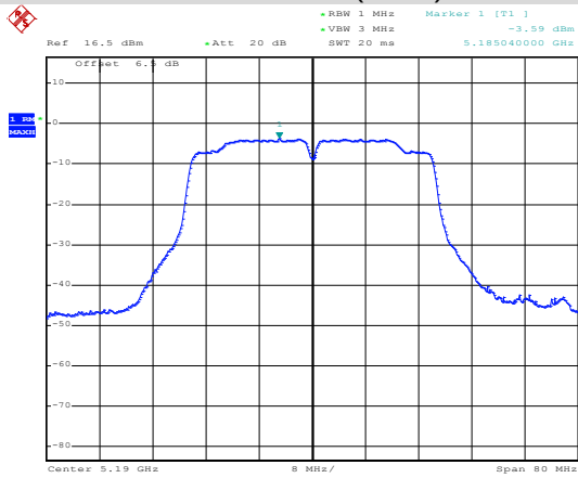
ANT1 802.11n(HT40)
