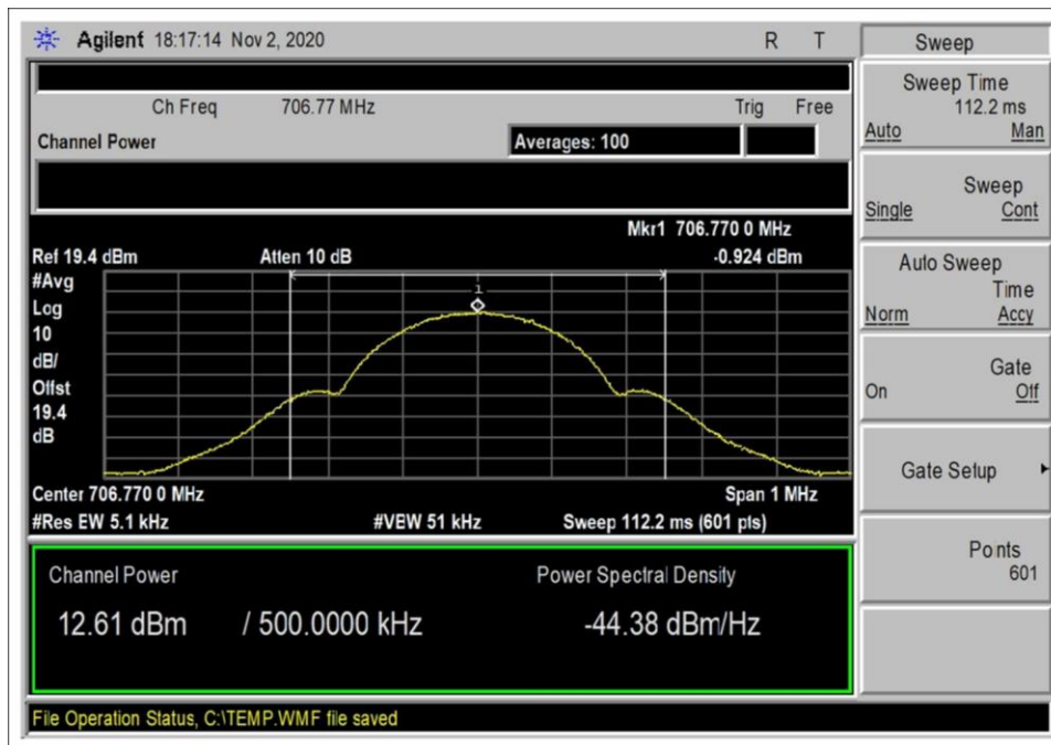
UL 698-716 AGC+3dB
