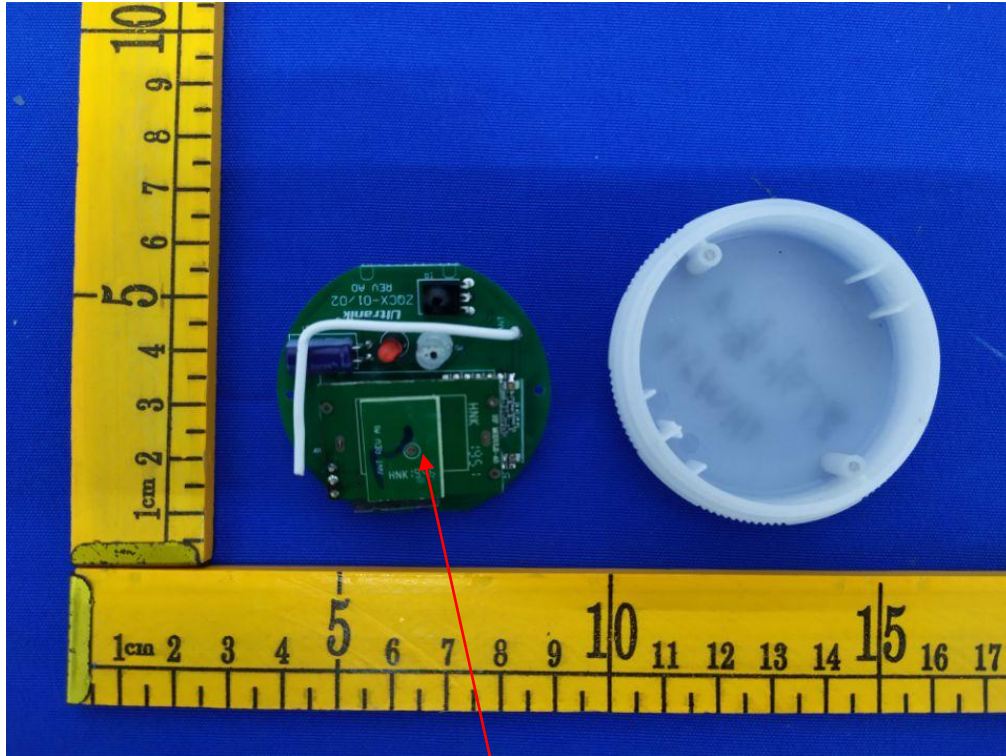
5.8GHz Antenna
