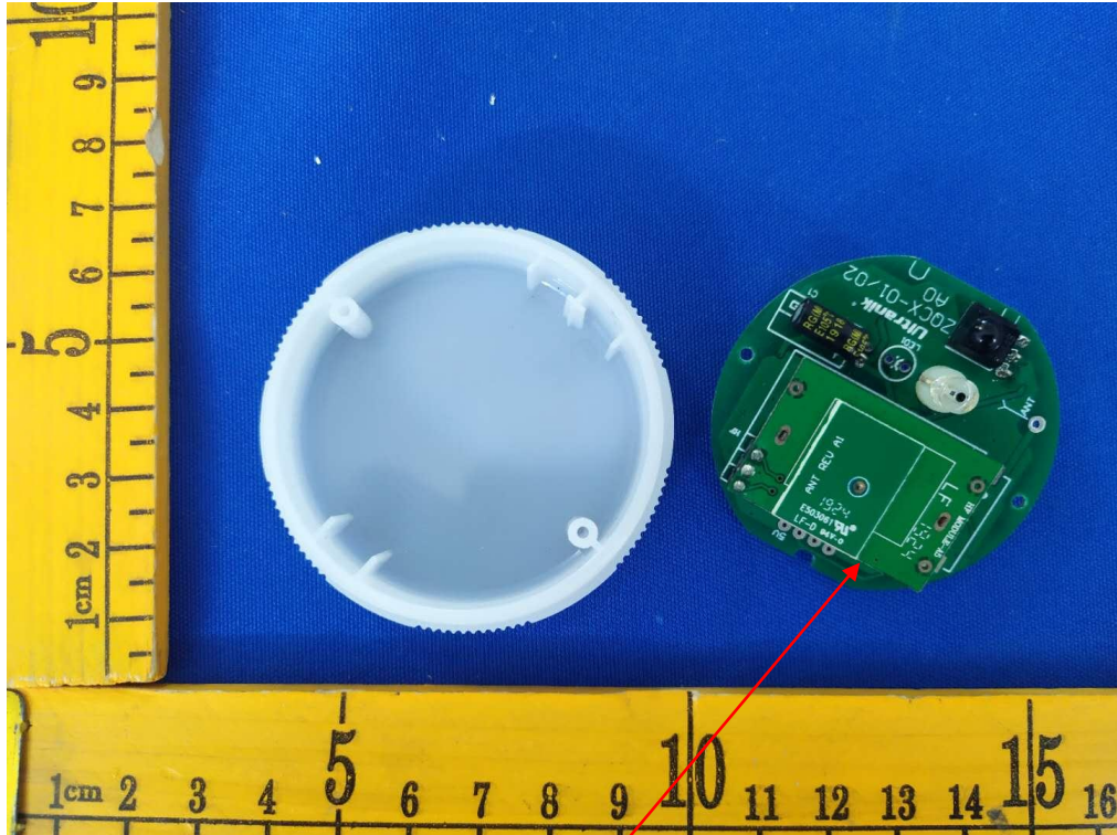
5.8GHz Antenna
