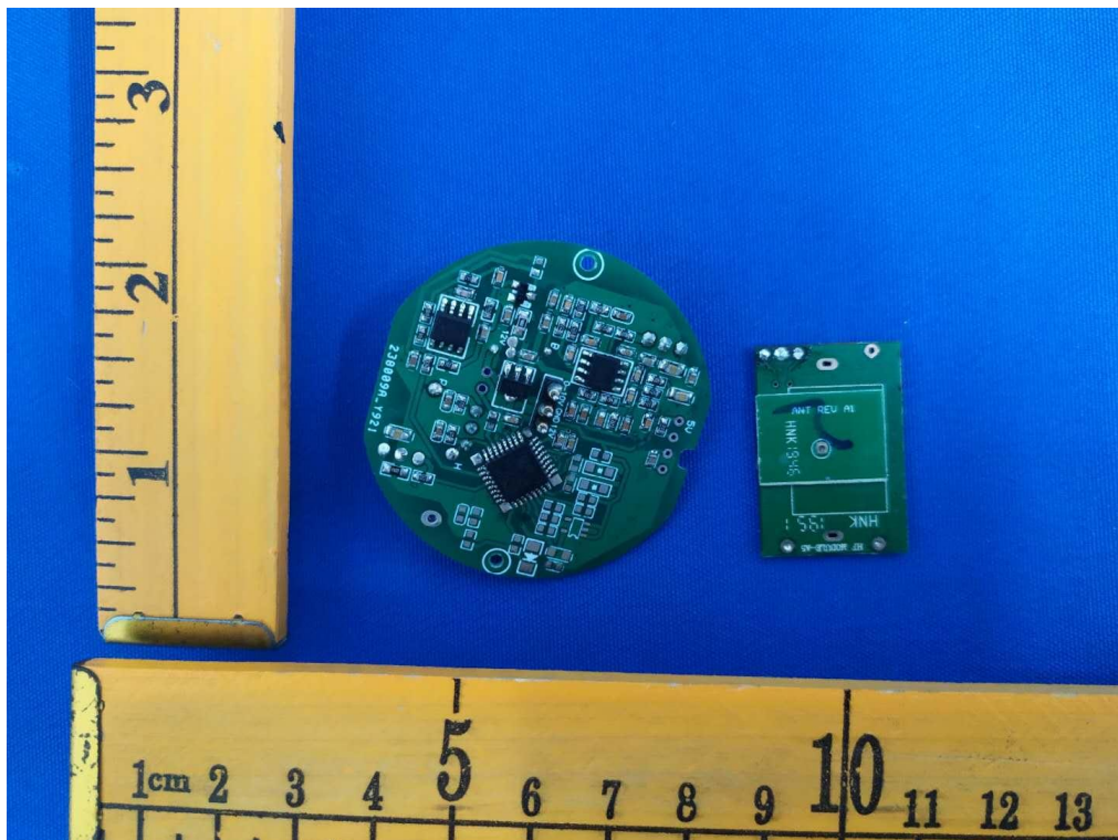
5.8GHz Antenna
