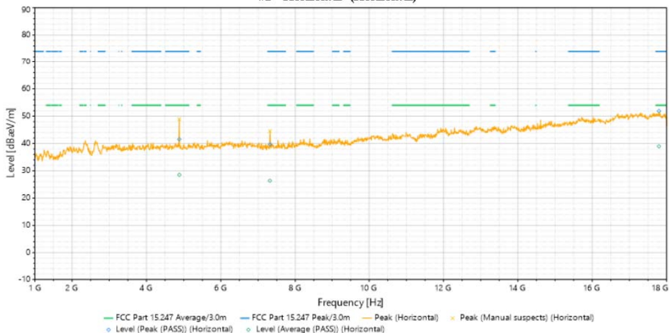
#2 - Horizontal (Horizontal)
