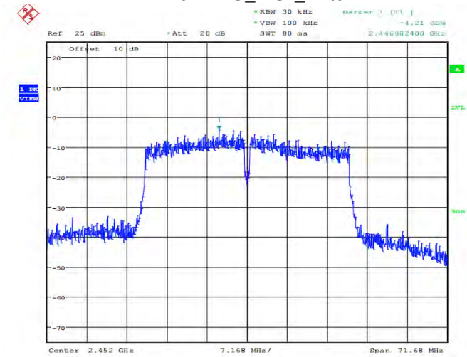
11N40MIMO_2452_Ant0
