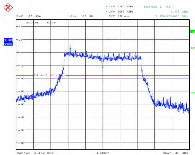
11N20MIMO_2462_Ant0
