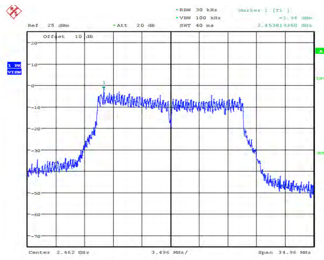
11N20MIMO_2462_Ant0
