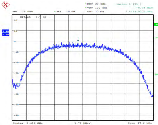
11BMIMO_2412_Ant0
