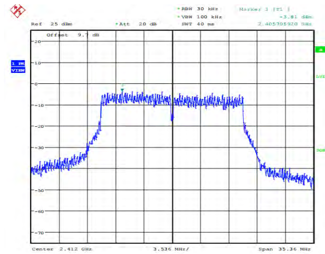
11N20MIMO_2412_Ant1
