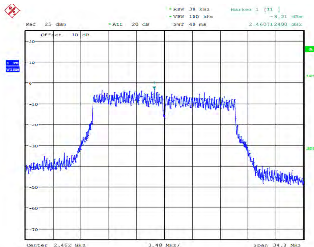
11N20MIMO_2462_Ant1
