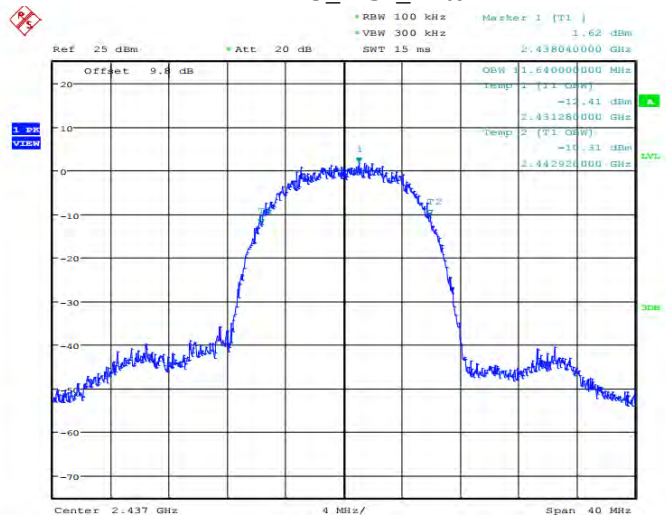
11BMIMO_2437_Ant0
