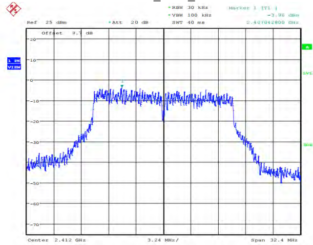
11GMIMO_2412_Ant0
