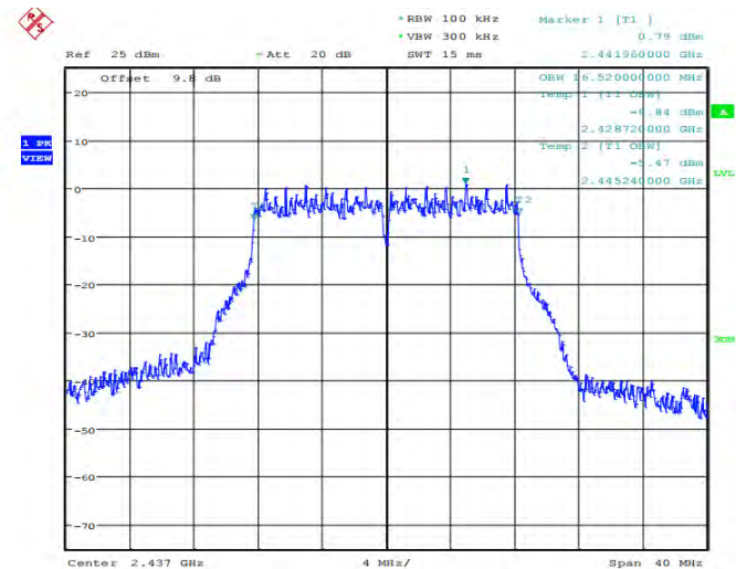
11GMIMO_2437_Ant1
