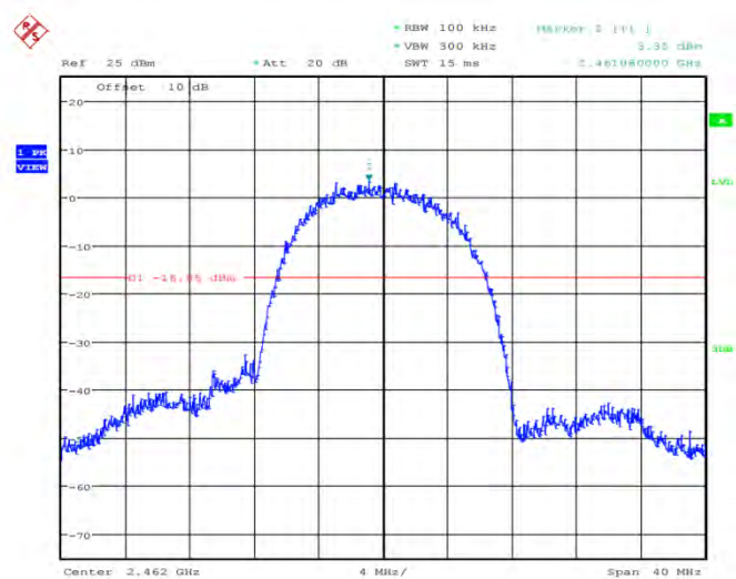
11BMIMO_2462_Ant1
