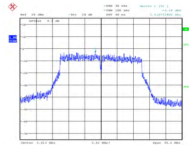
11N20MIMO_2412_Ant1
