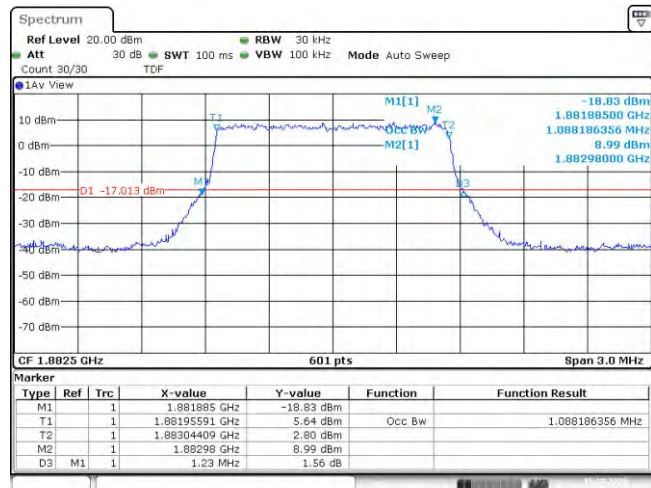
Band25-1.4MHz-QPSK-26365-6RB#0-1.088
