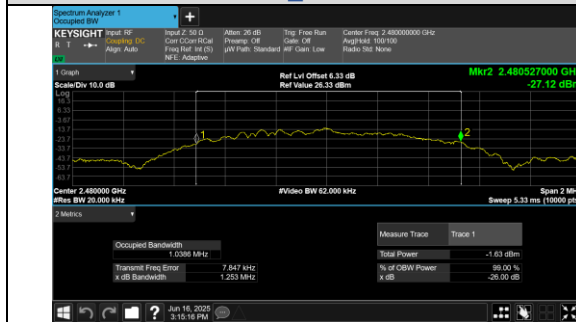
BLE 1M Channel 39
