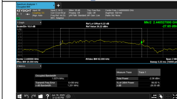
BLE 1M Channel 19
