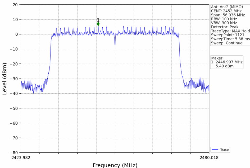
802.11ax(HEW40)_HCH_2452MHz_RU484_Left_Ant2 (MIMO)_NTNV
