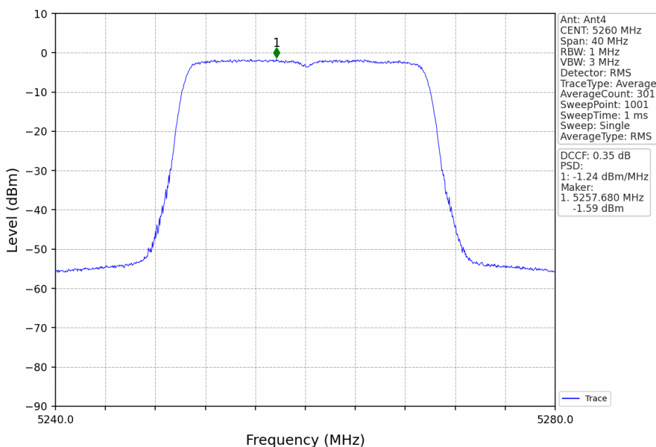
802.11ax(HEW20)_LCH_5260MHz_RU242_Left_Ant4_NTNV
