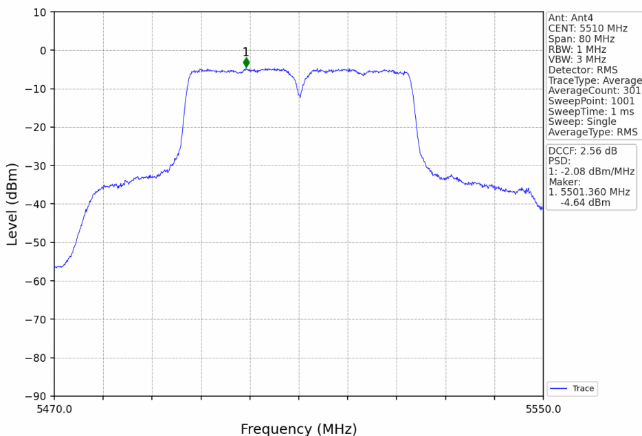
802.11n(HT40)_LCH_5510MHz_Ant4_NTNV
