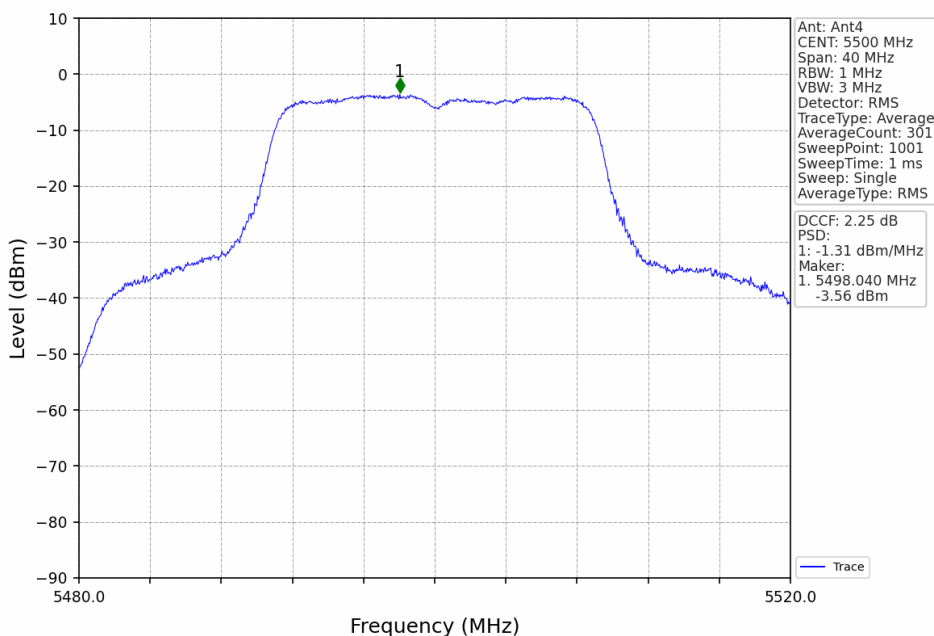
802.11n(HT20)_LCH_5500MHz_MIMO_NTNV
