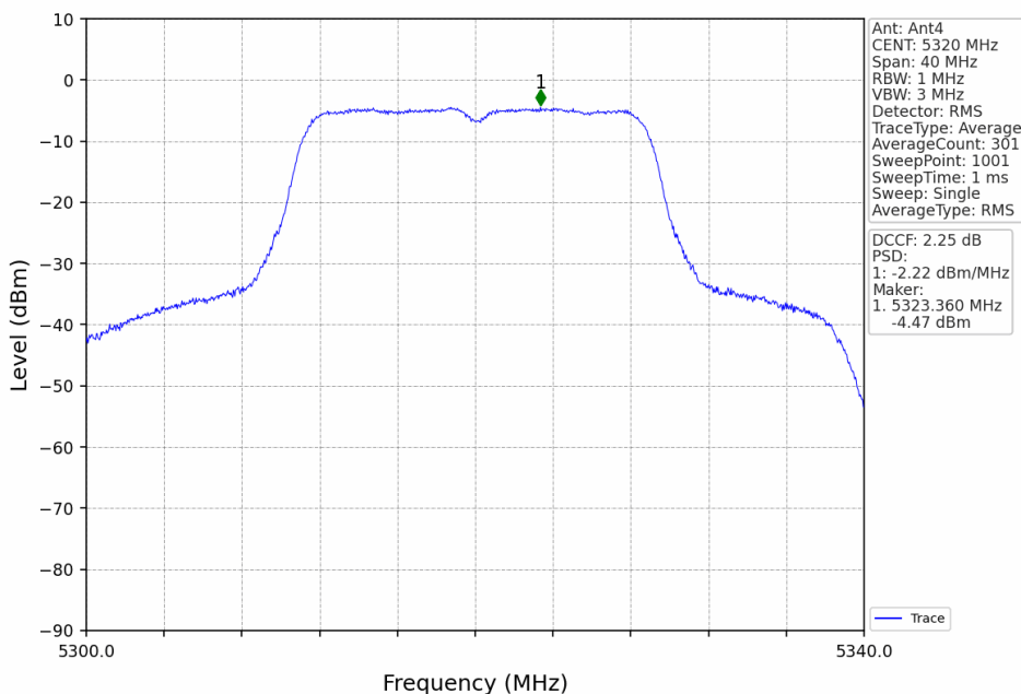
802.11n(HT20)_HCH_5320MHz_Ant4_NTNV
