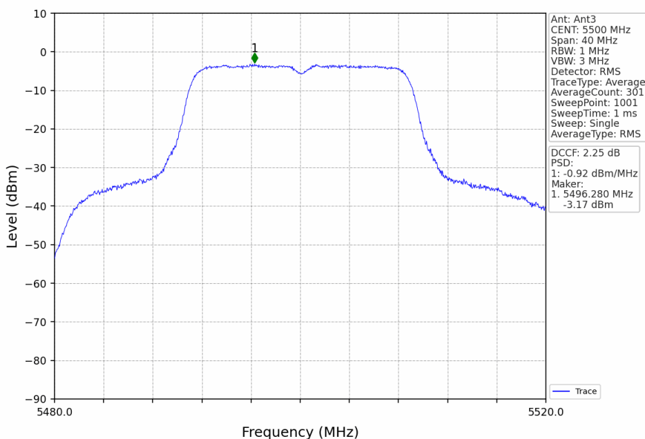
802.11n(HT20)_LCH_5500MHz_Ant3_NTNV
