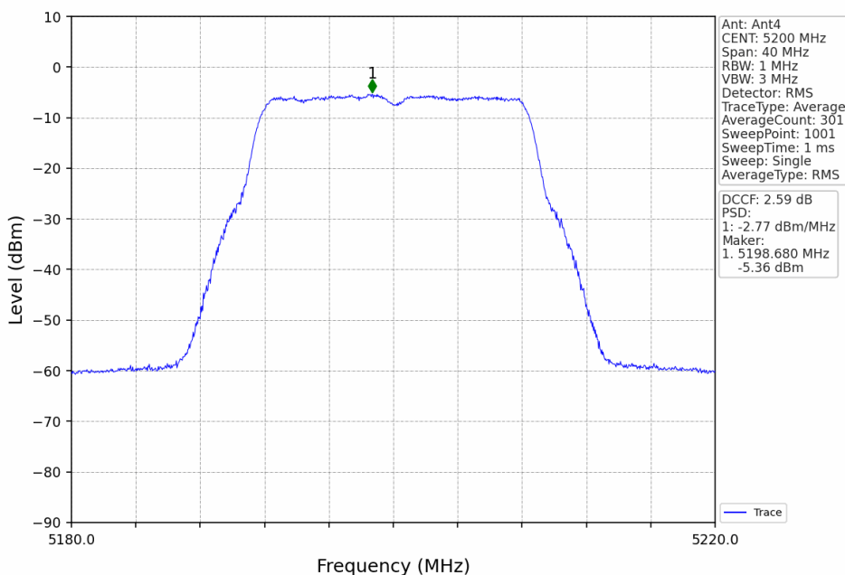
802.11a_MCH_5200MHz_MIMO_NTNV
