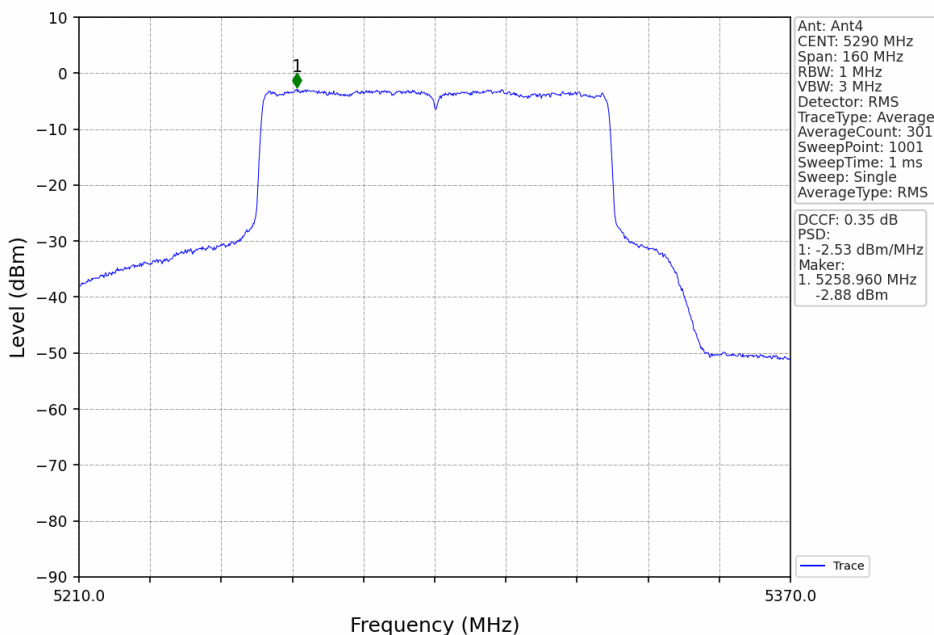
802.11ax(HEW80)_MCH_5290MHz_RU996_Left_Ant4_NTNV
