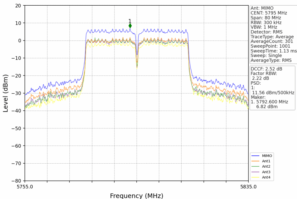
802.11n(HT40)_HCH_5795MHz_MIMO_NTNV
