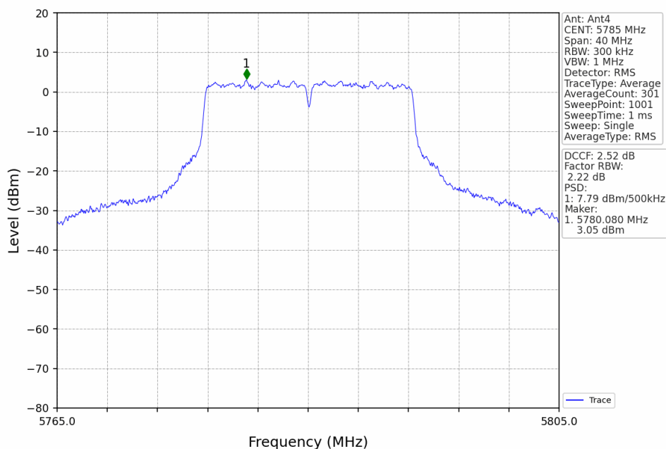
802.11a_MCH_5785MHz_MIMO_NTNV
