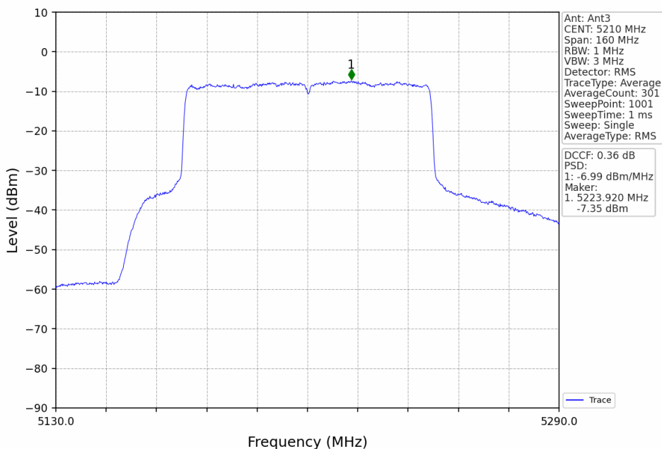
802.11ax(HEW80)_MCH_5210MHz_RU996_Left_Ant3_NTNV
