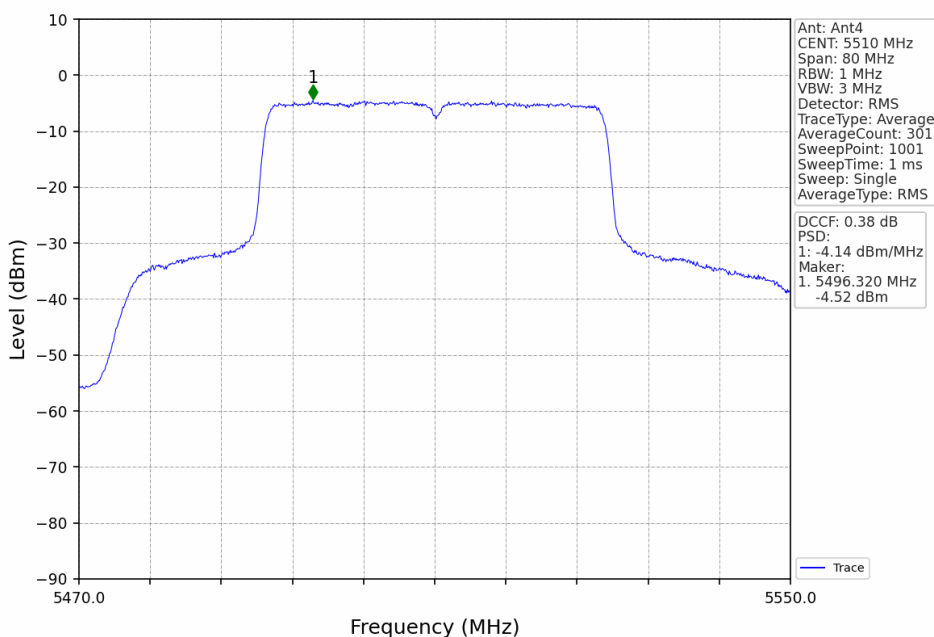
802.11ax(HEW40)_LCH_5510MHz_RU484_Left_Ant4_NTNV
