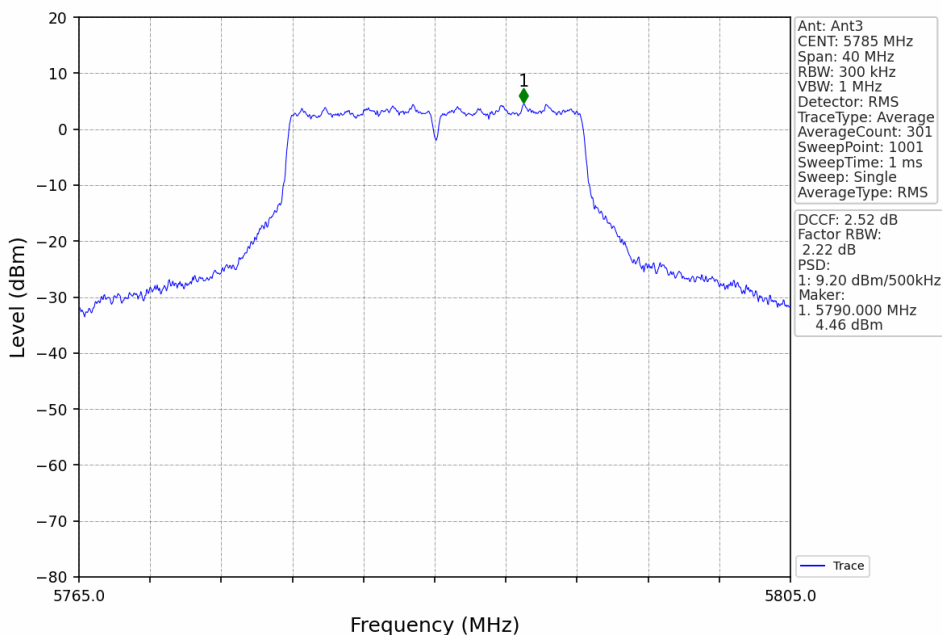
802.11a_MCH_5785MHz_Ant3_NTNV
