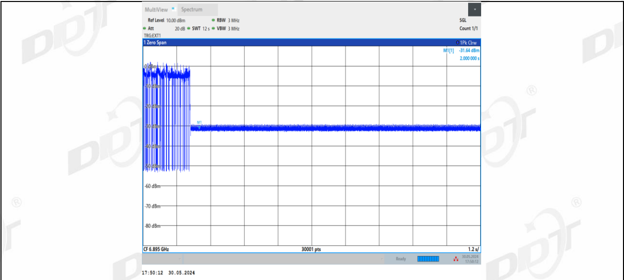
11BE20MIMO_Ant1_6895_Center_6895_7
