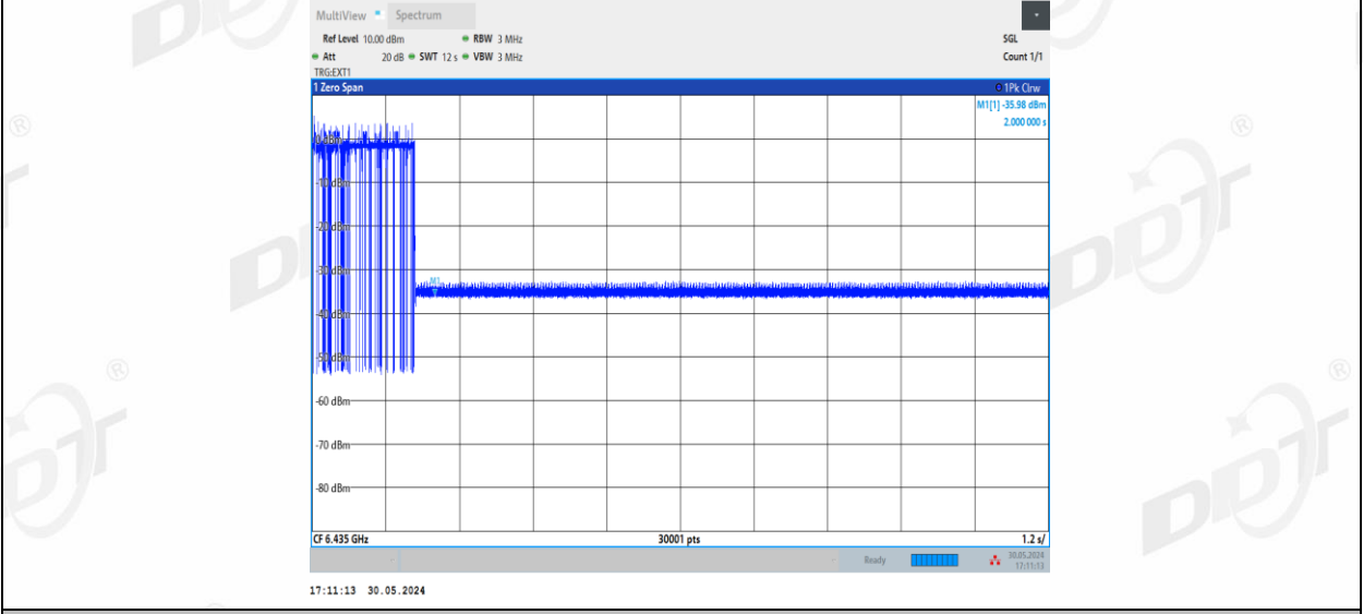
11BE20MIMO_Ant1_6435_Center_6435_2
