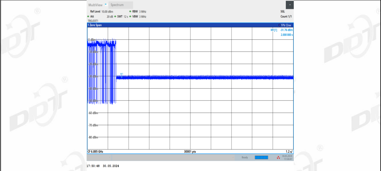
11BE20MIMO_Ant1_6895_Center_6895_8
