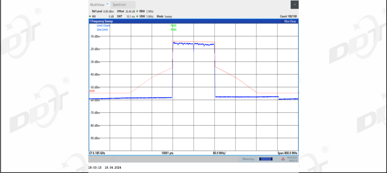
11BE160MIMO_Ant3_6185
