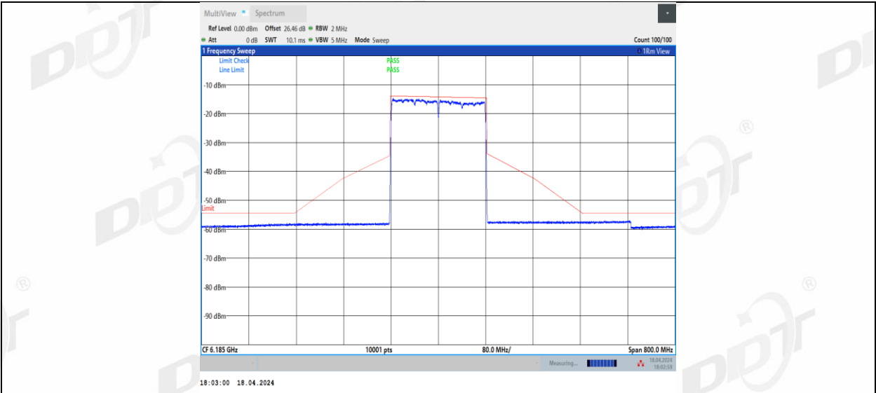
11BE160MIMO_Ant2_6185
