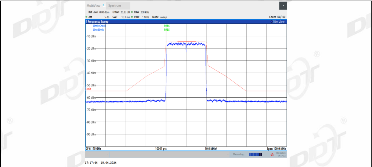
11BE20MIMO_Ant2_6175
