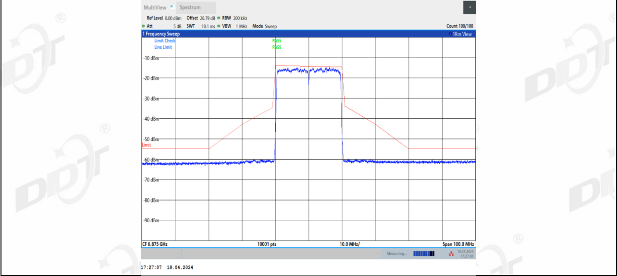
11BE20MIMO_Ant3_6875
