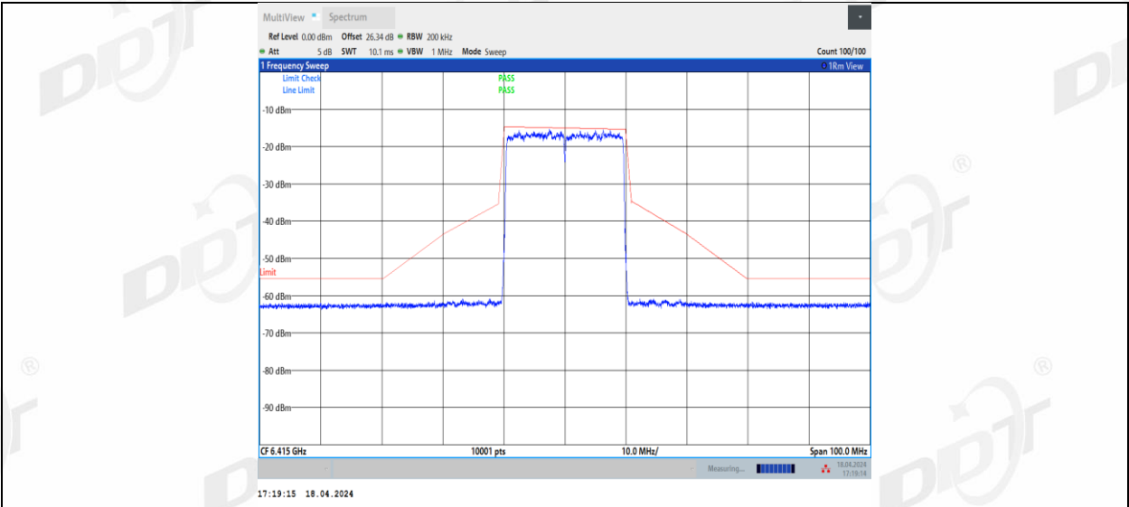
11BE20MIMO_Ant2_6415
