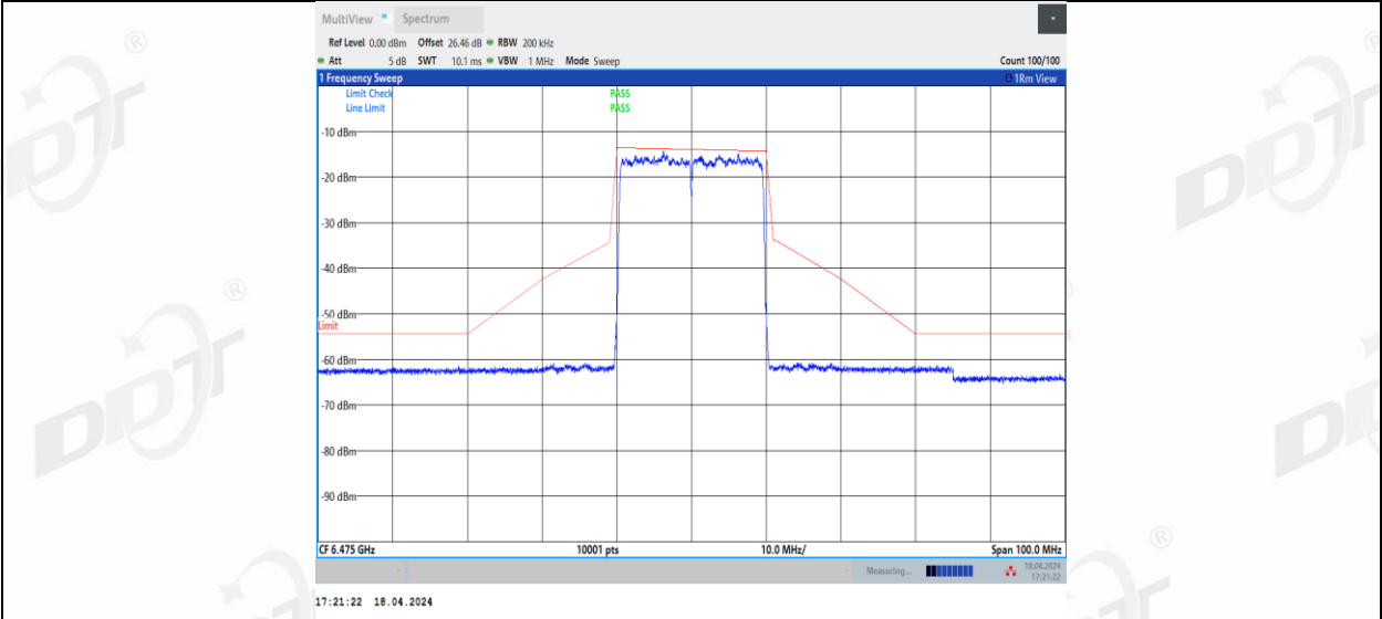
11BE20MIMO_Ant3_6475
