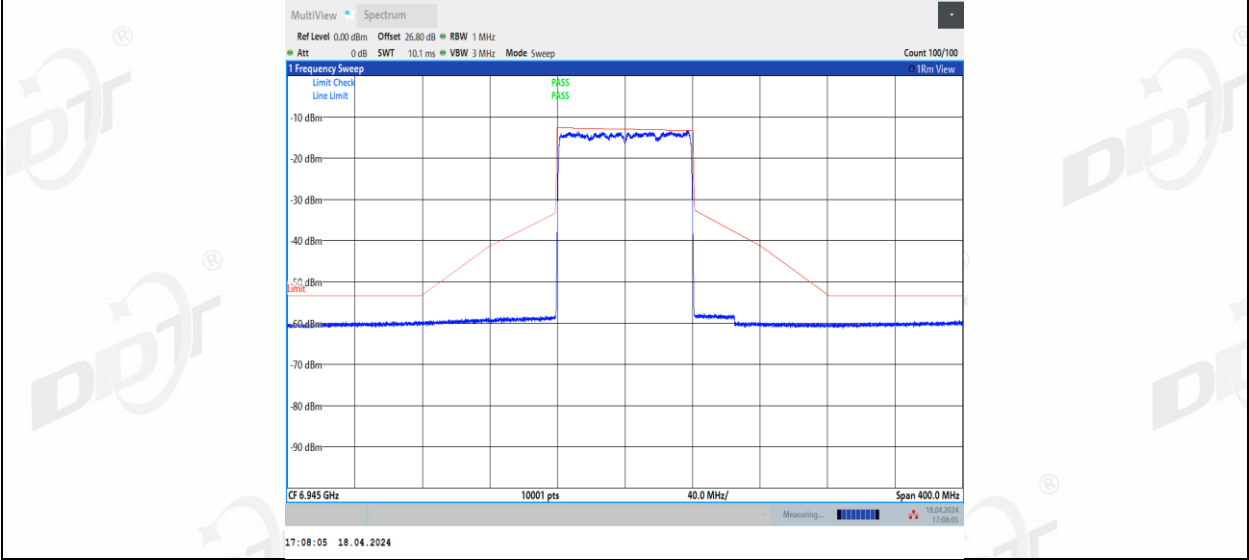
11AX80MIMO_Ant3_6945
