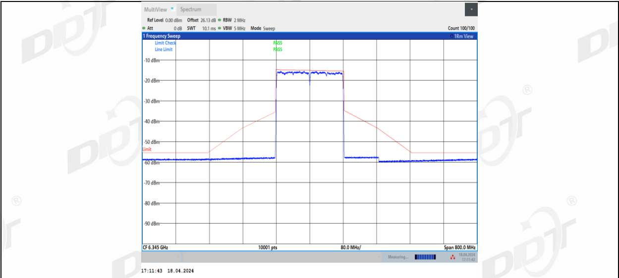
11AX160MIMO_Ant2_6345
