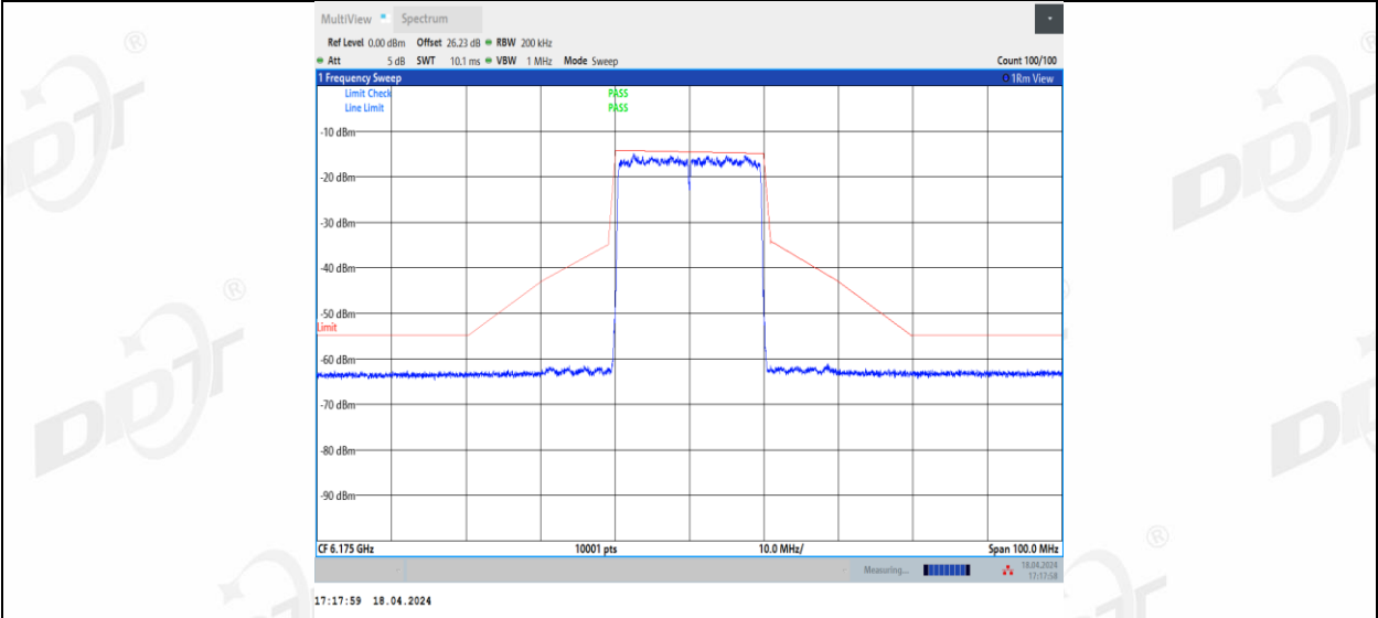
11BE20MIMO_Ant3_6175
