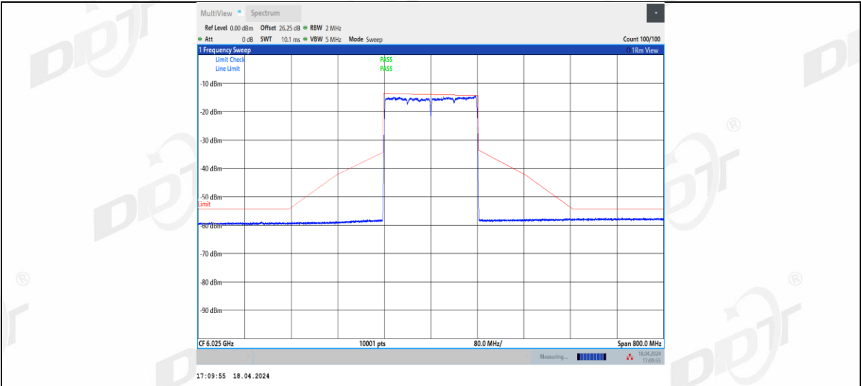
11AX160MIMO_Ant2_6025
