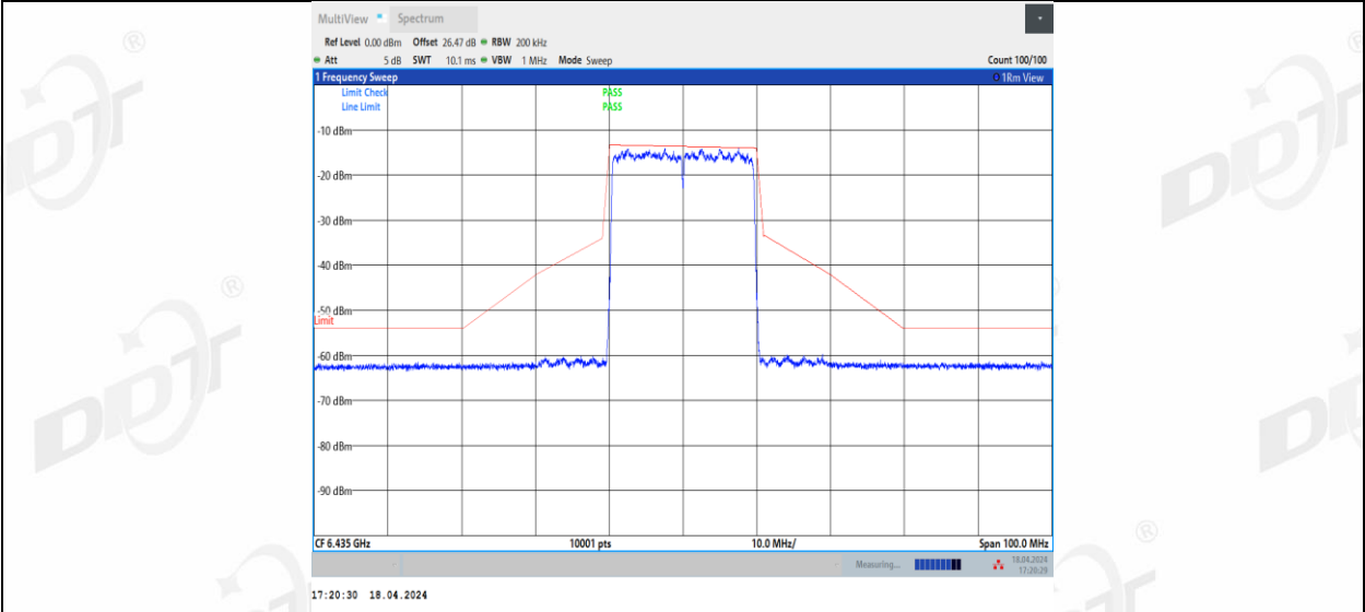
11BE20MIMO_Ant3_6435
