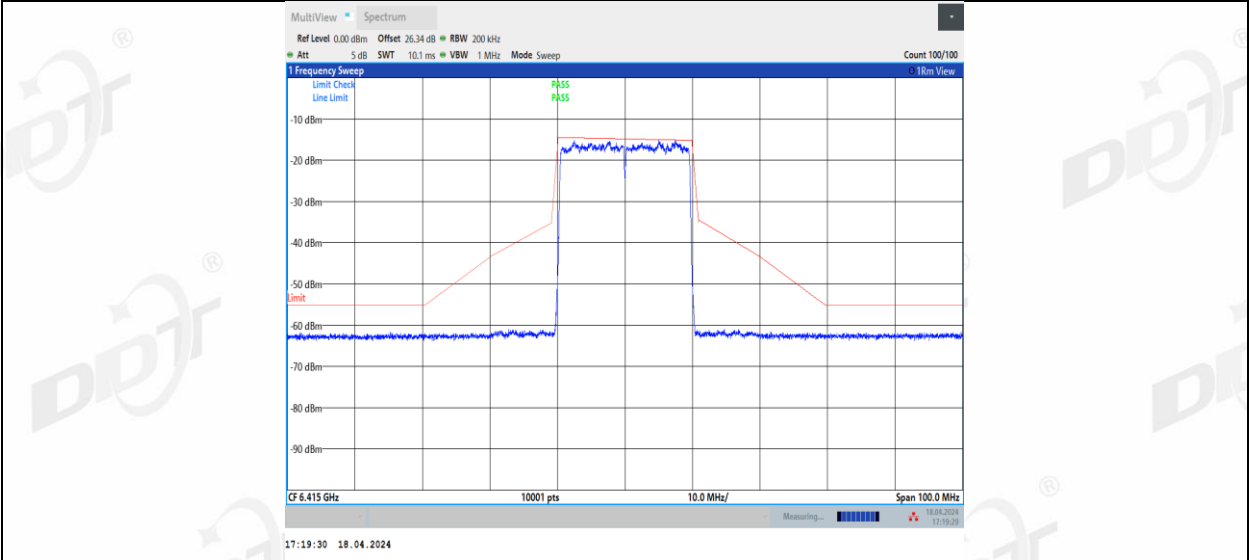
11BE20MIMO_Ant3_6415
