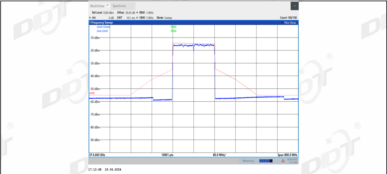
11AX160MIMO_Ant2_6665
