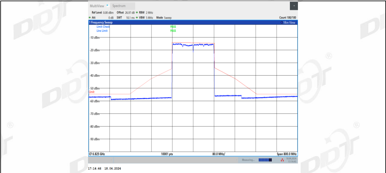
11AX160MIMO_Ant2_6825
