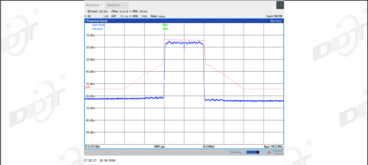
11BE20MIMO_Ant3_6515
