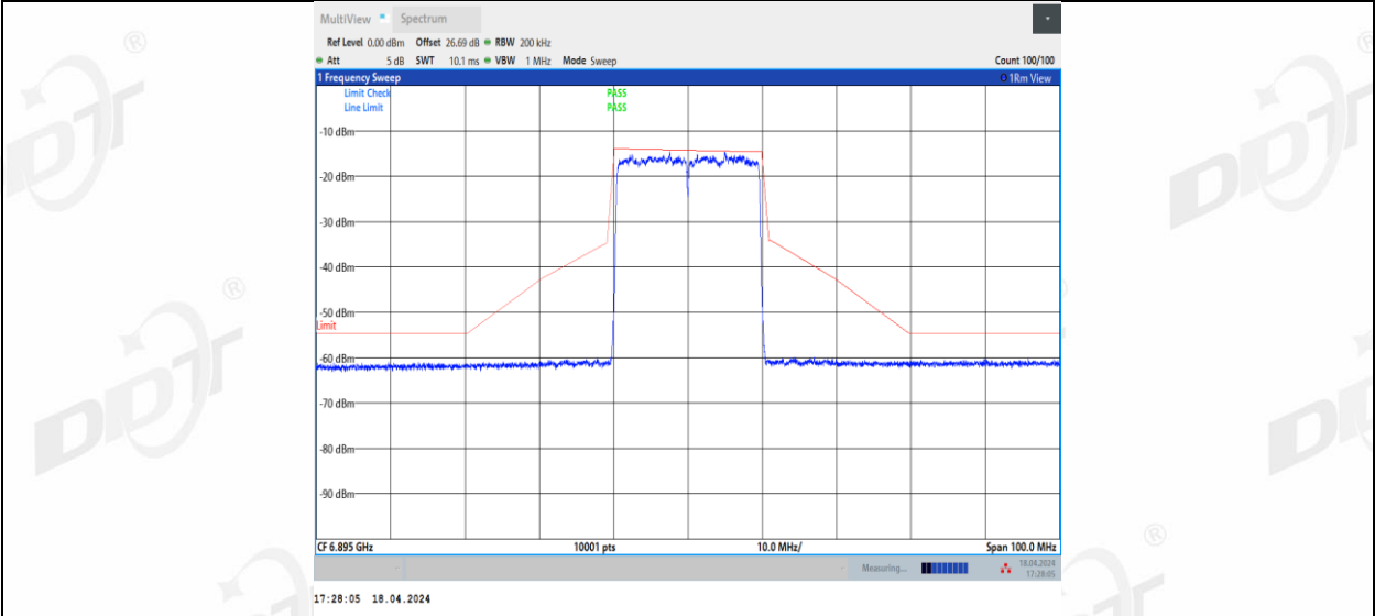
11BE20MIMO_Ant3_6895
