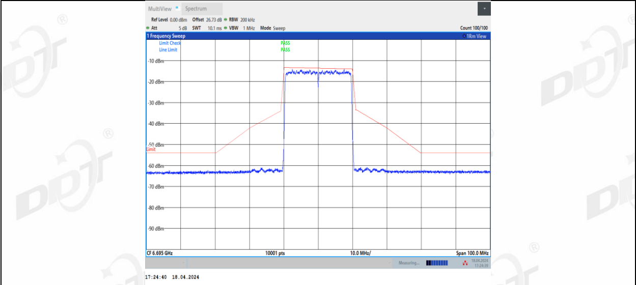
11BE20MIMO_Ant3_6695
