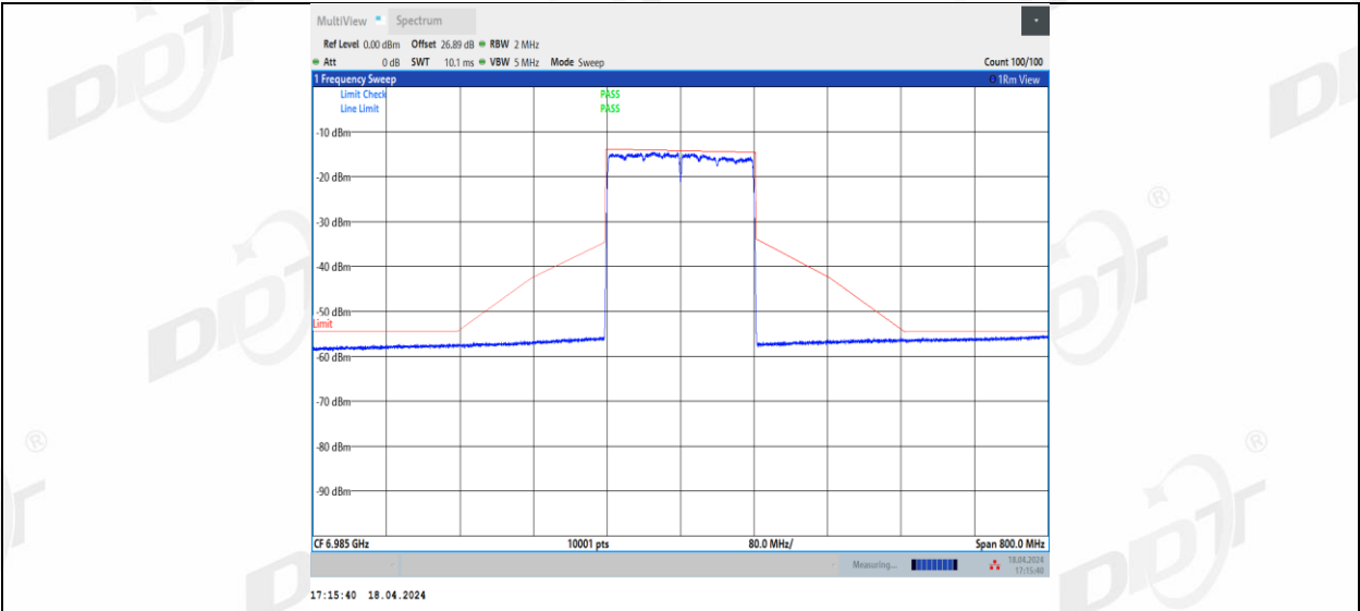
11AX160MIMO_Ant2_6985
