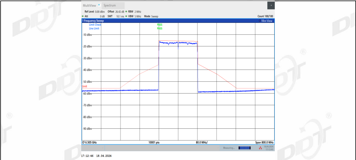
11AX160MIMO_Ant2_6505
