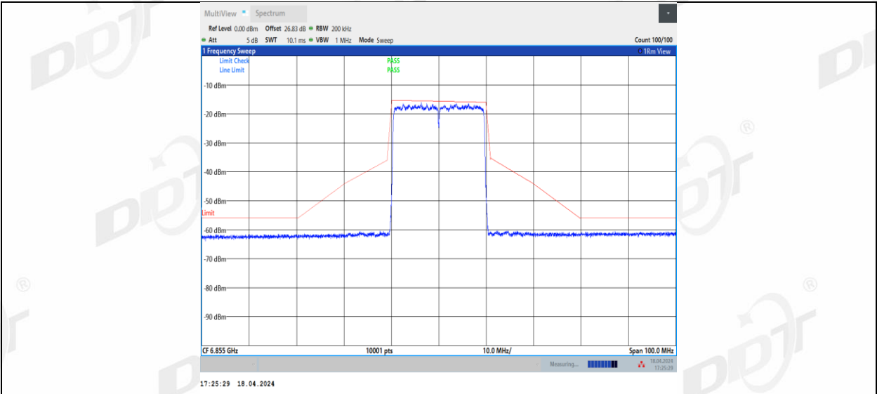
11BE20MIMO_Ant2_6855
