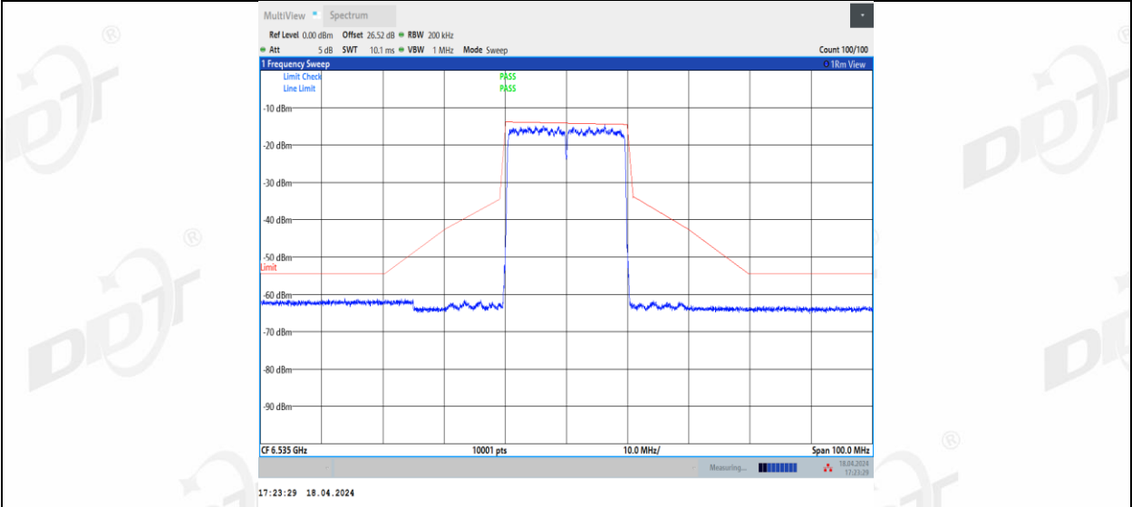
11BE20MIMO_Ant3_6535
