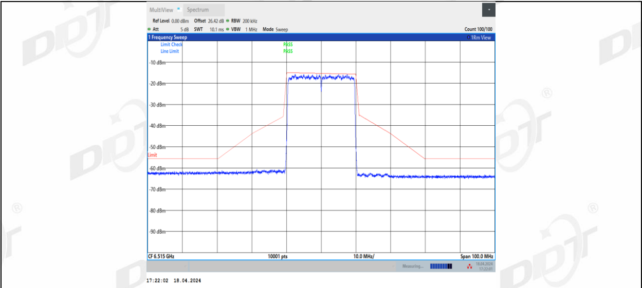
11BE20MIMO_Ant2_6515
