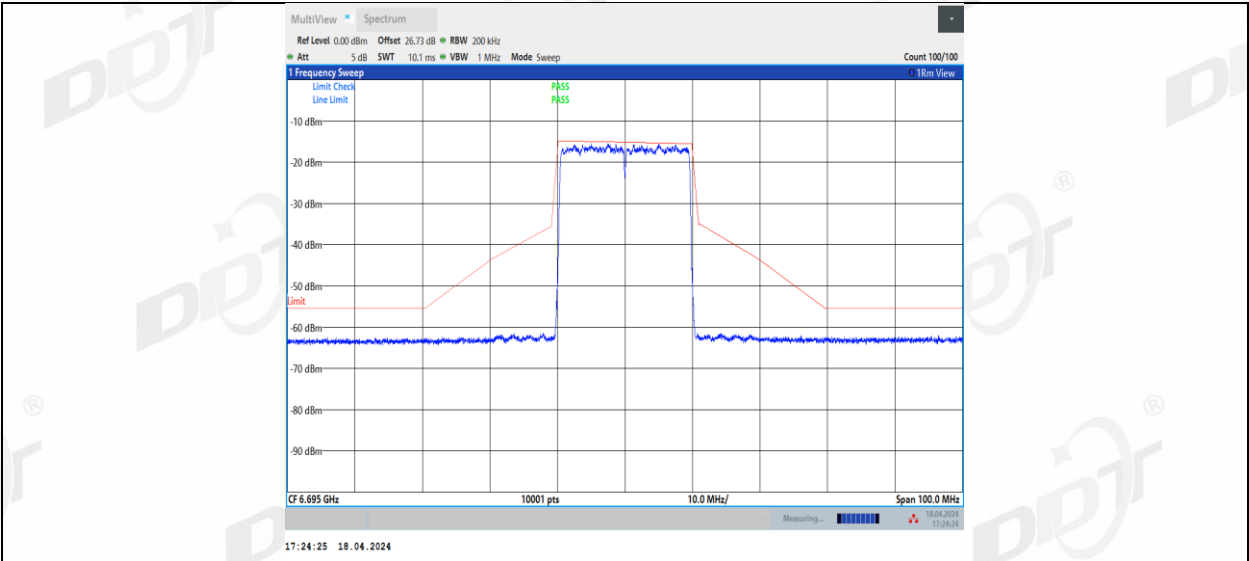
11BE20MIMO_Ant2_6695
