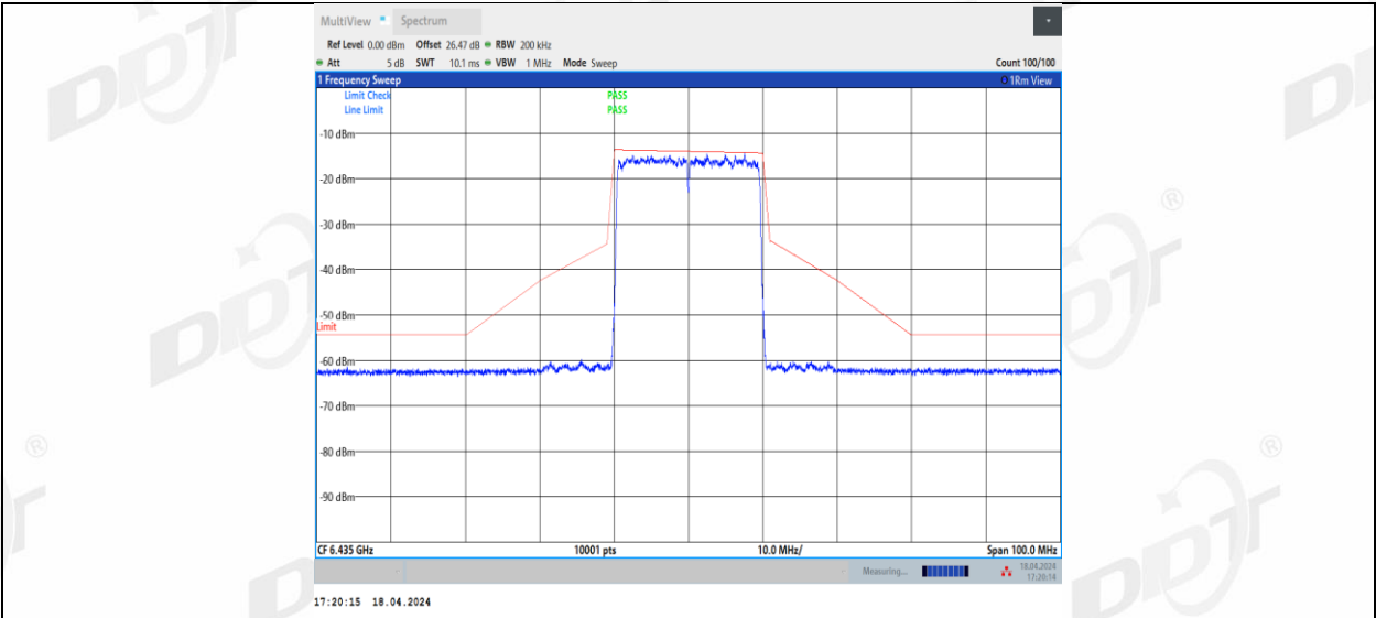
11BE20MIMO_Ant2_6435
