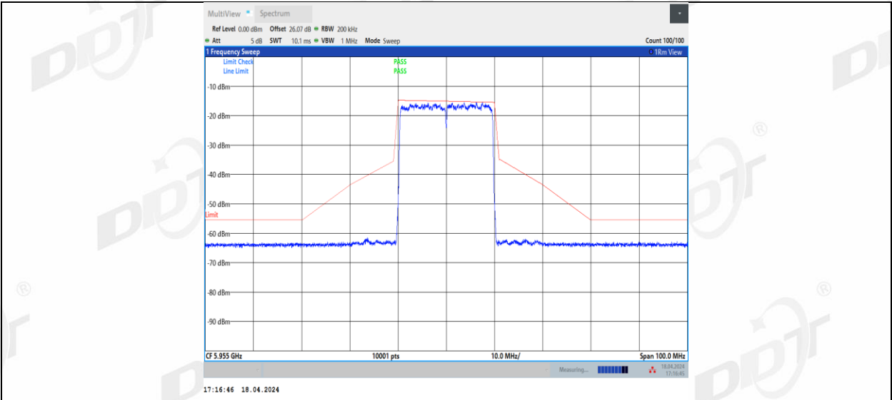
11BE20MIMO_Ant2_5955
