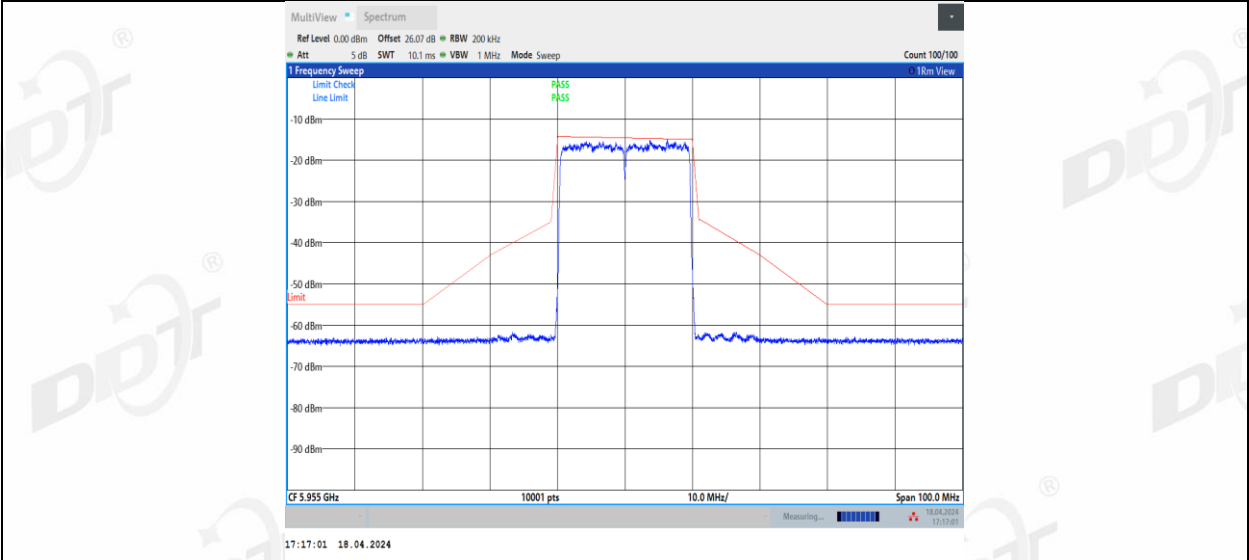
11BE20MIMO_Ant3_5955
