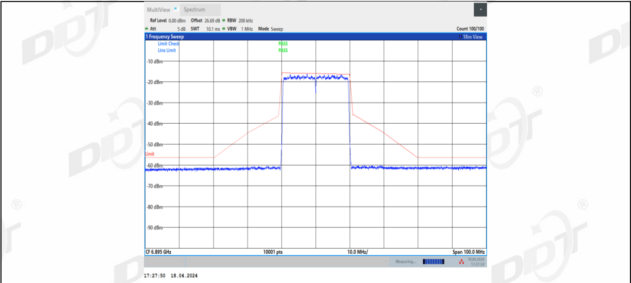
11BE20MIMO_Ant2_6895
