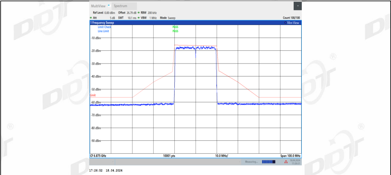
11BE20MIMO_Ant2_6875
