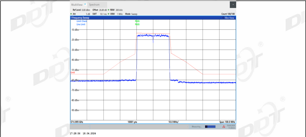
11BE20MIMO_Ant2_6995
