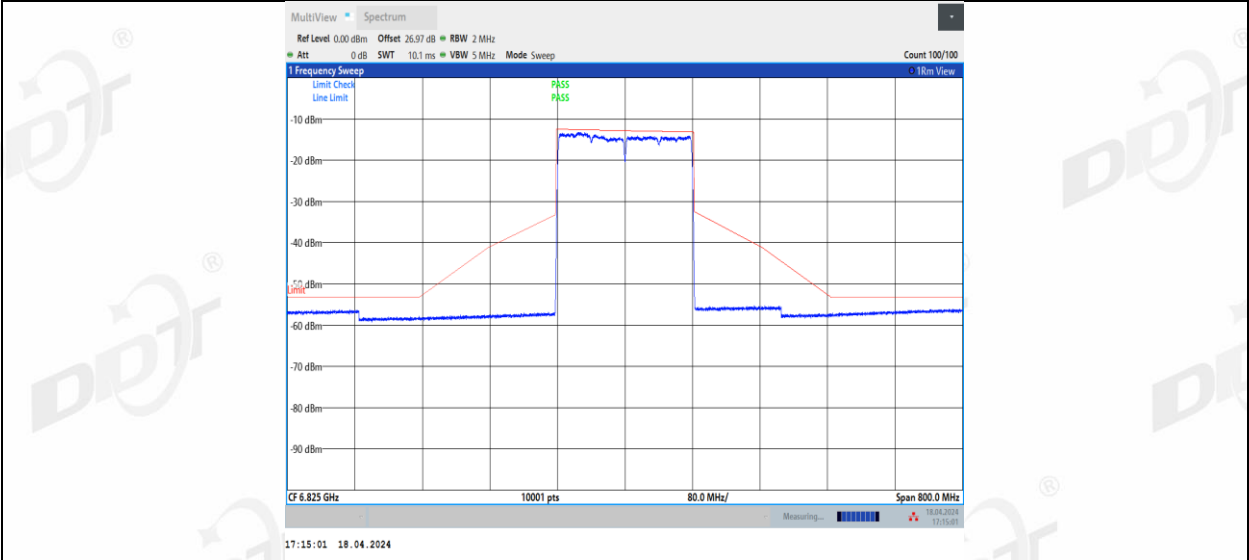
11AX160MIMO_Ant3_6825
