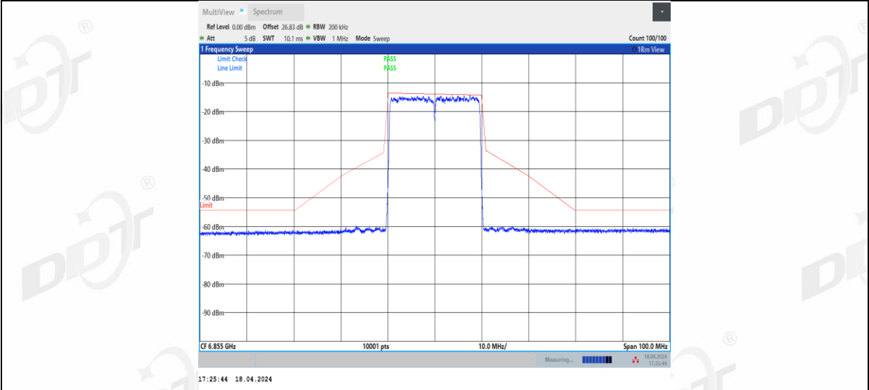
11BE20MIMO_Ant3_6855
