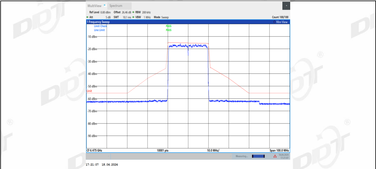
11BE20MIMO_Ant2_6475
