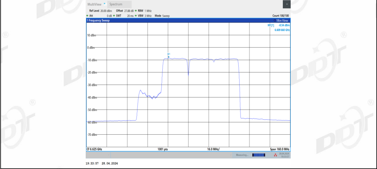
11BE80MIMO_Ant3_6625_484+242_2
