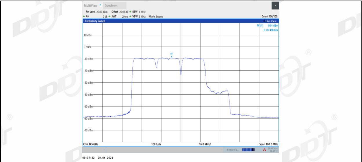
11BE80MIMO_Ant2_6145_484+242_1
