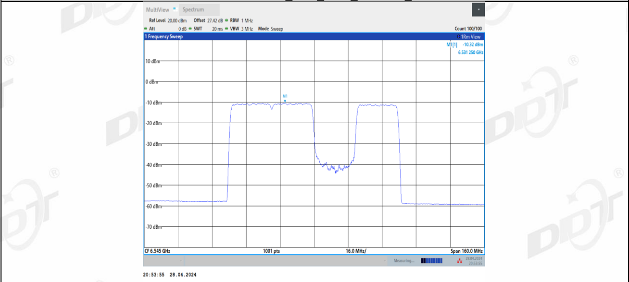
11BE80MIMO_Ant1_6545_484+242_4
