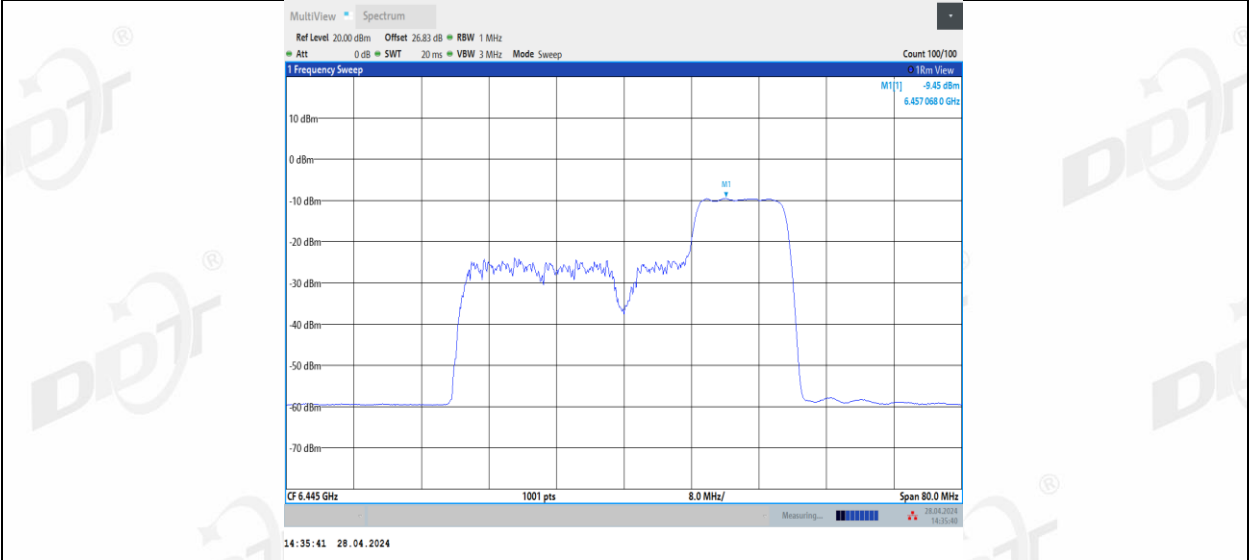
11BE40MIMO_Ant2_6445_106+26_3
