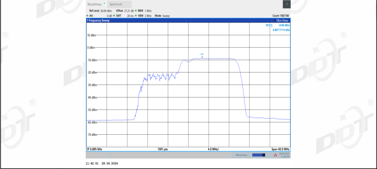
11BE20MIMO_Ant1_6995_52+26_1
