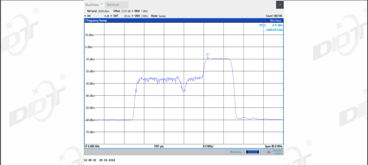
11BE40MIMO_Ant2_6685_106+26_3
