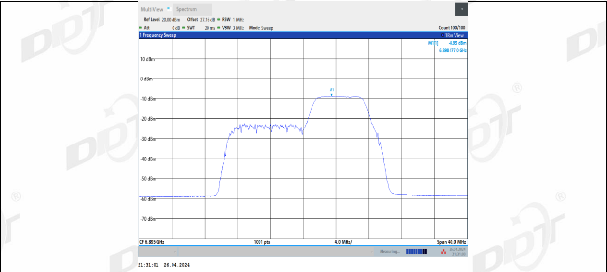
11BE20MIMO_Ant3_6895_106+26_1
