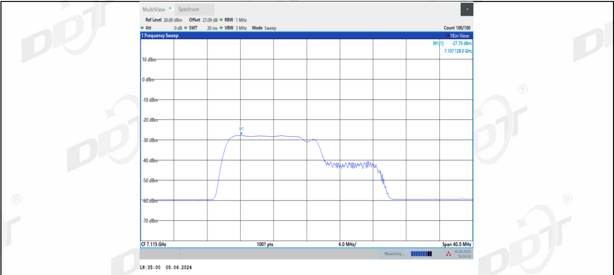
11BE20MIMO_Ant1_7115_106+26_2
