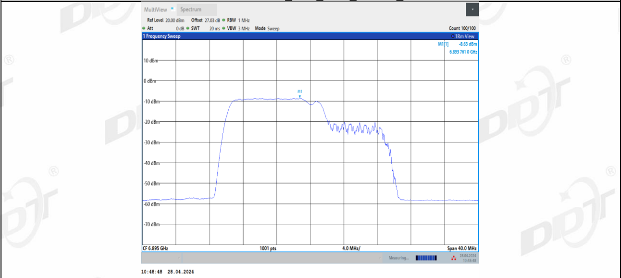
11BE20MIMO_Ant2_6895_106+26_2
