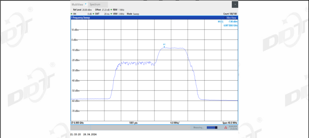
11BE20MIMO_Ant2_6995_106+26_1
