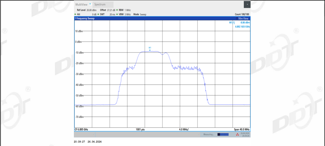
11BE20MIMO_Ant3_6895_52+26_3
