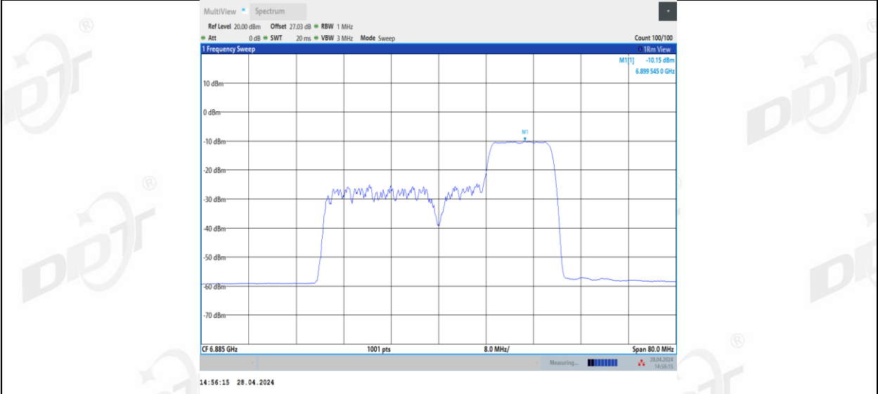
11BE40MIMO_Ant2_6885_106+26_3
