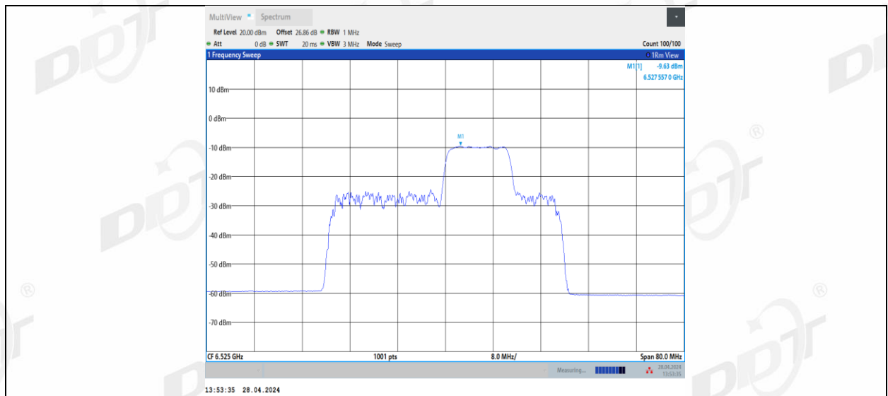
11BE40MIMO_Ant1_6525_106+26_4
