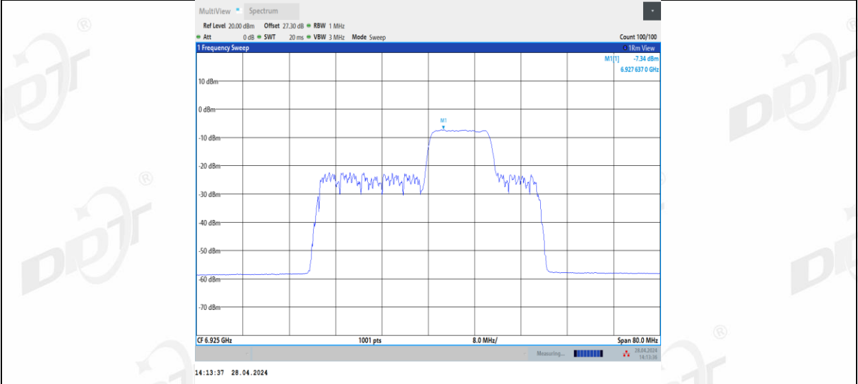
11BE40MIMO_Ant3_6925_106+26_4
