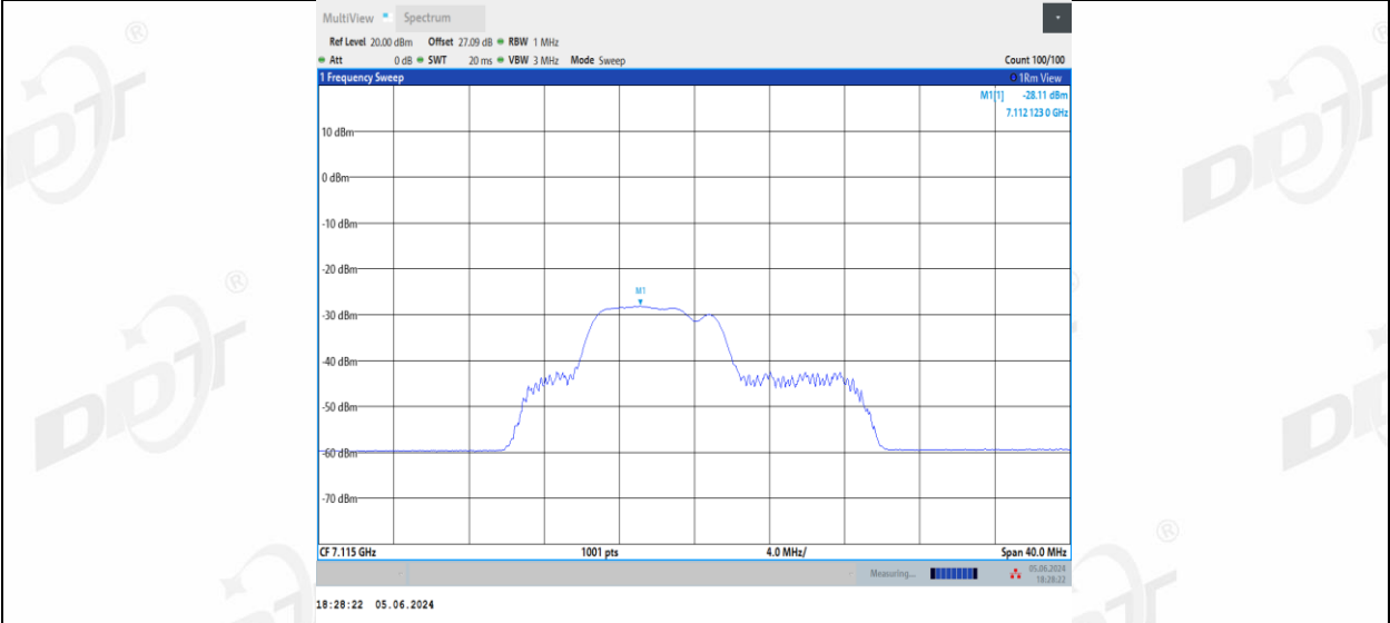
11BE20MIMO_Ant1_7115_52+26_3
