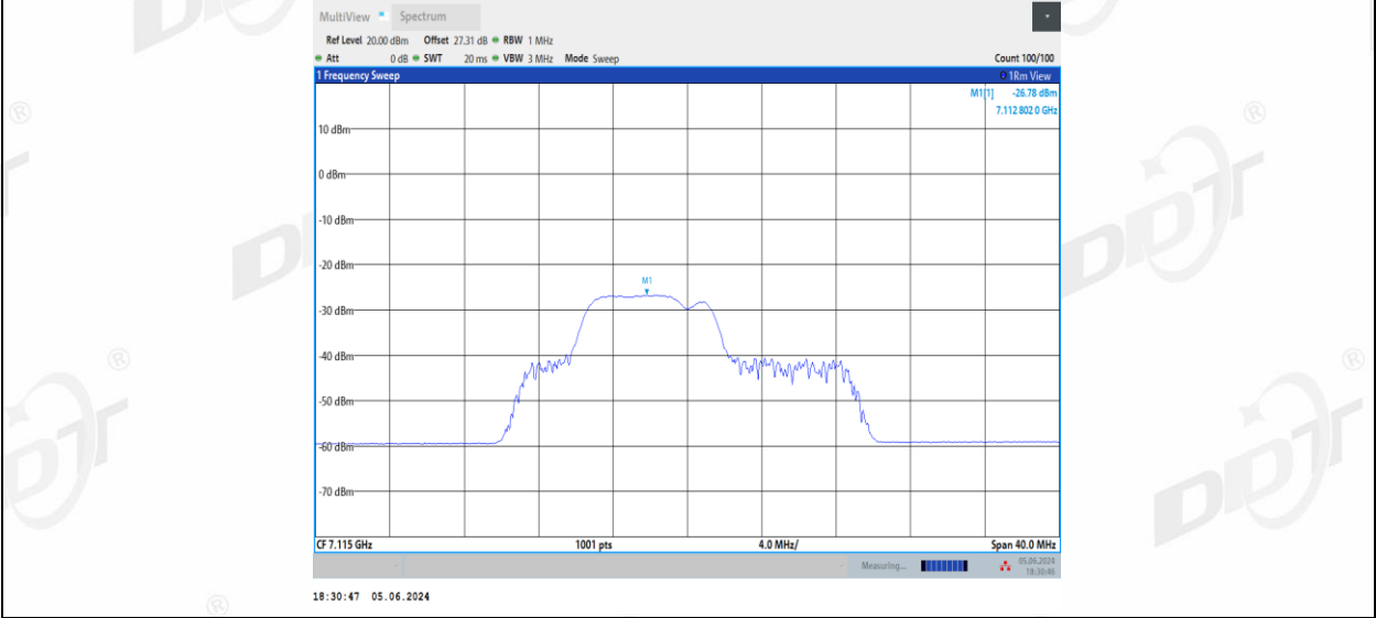
11BE20MIMO_Ant3_7115_52+26_3
