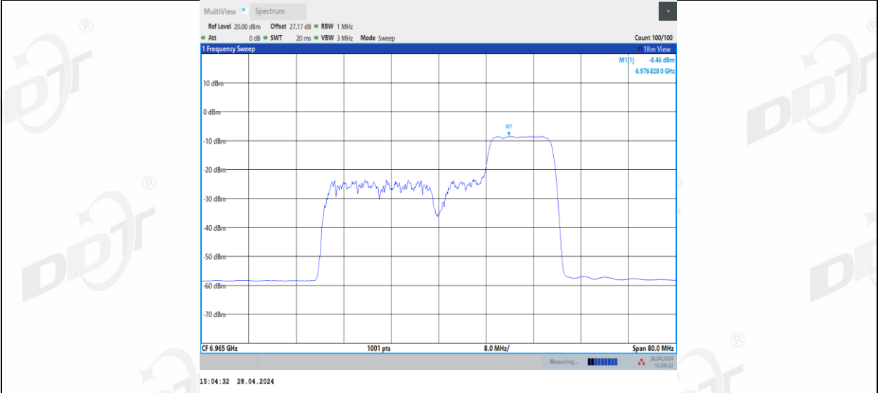
11BE40MIMO_Ant2_6965_106+26_3
