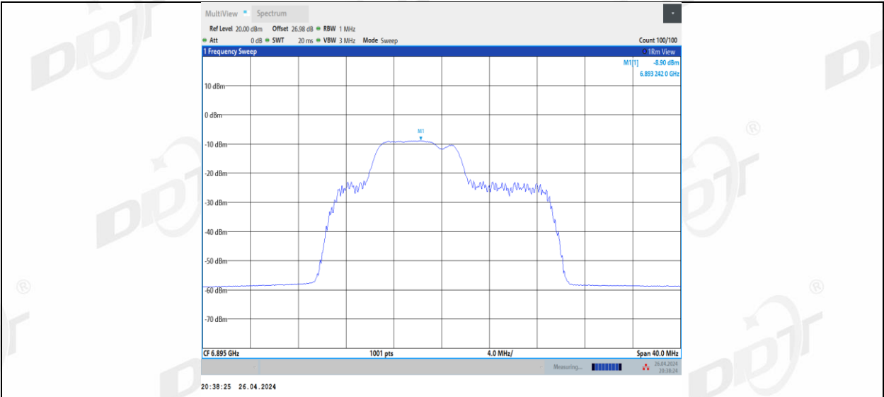
11BE20MIMO_Ant2_6895_52+26_3
