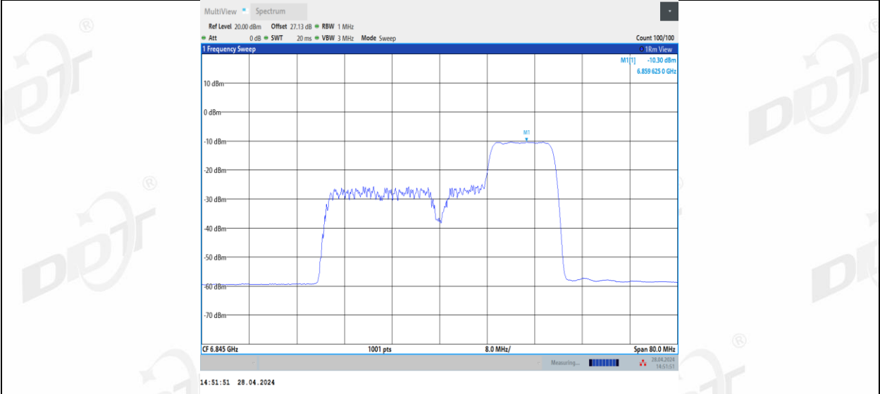
11BE40MIMO_Ant2_6845_106+26_3
