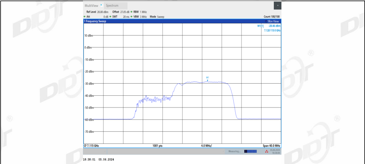
11BE20MIMO_Ant3_7115_52+26_1
