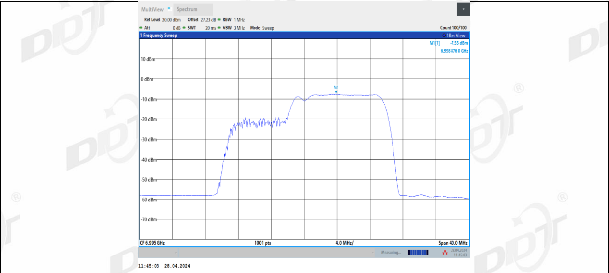
11BE20MIMO_Ant3_6995_52+26_1
