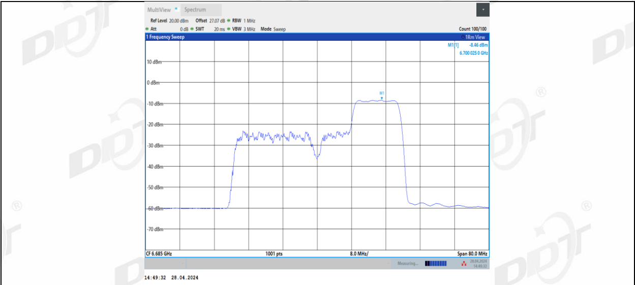
11BE40MIMO_Ant3_6685_106+26_3
