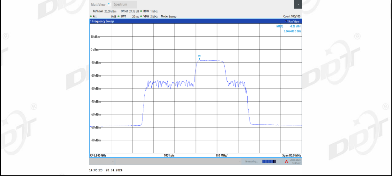
11BE40MIMO_Ant2_6845_106+26_4
