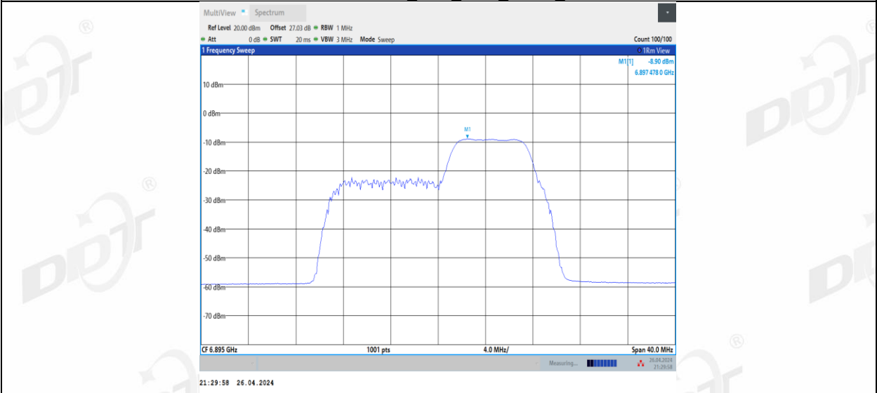
11BE20MIMO_Ant2_6895_106+26_1
