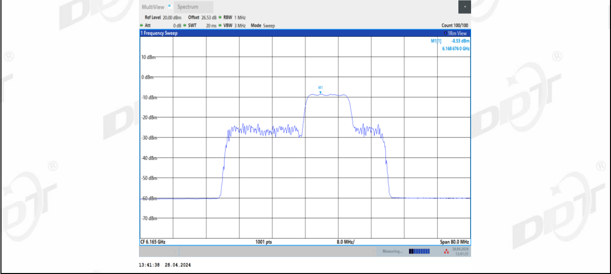
11BE40MIMO_Ant2_6165_106+26_4
