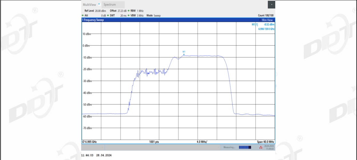
11BE20MIMO_Ant2_6995_52+26_1
