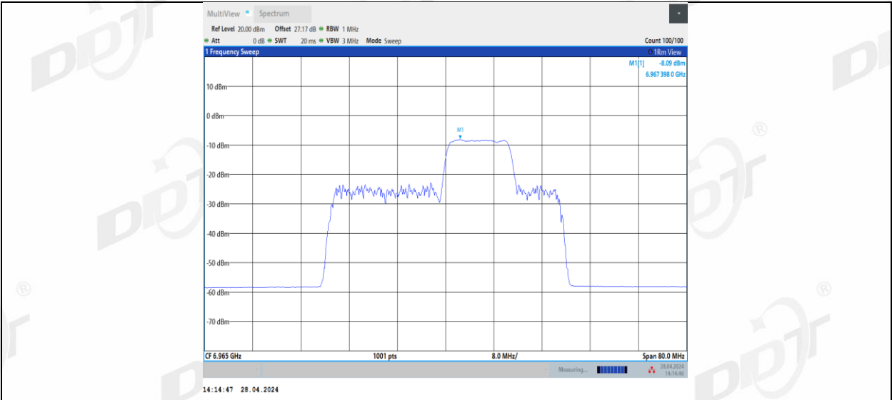
11BE40MIMO_Ant1_6965_106+26_4
