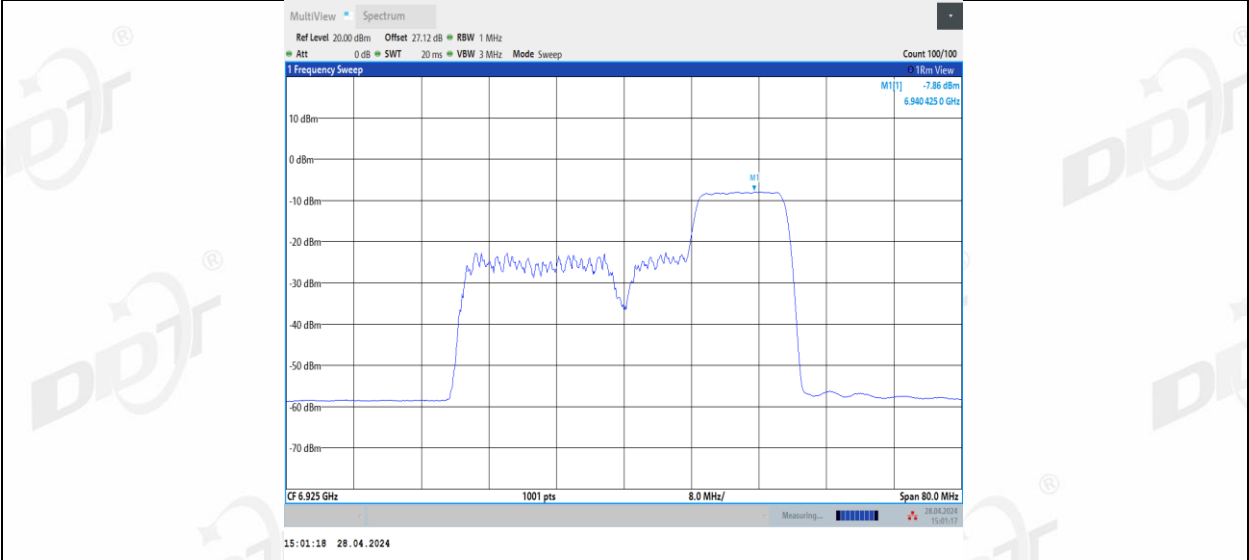
11BE40MIMO_Ant2_6925_106+26_3
