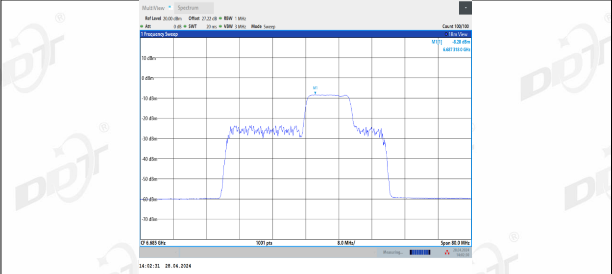
11BE40MIMO_Ant3_6685_106+26_4
