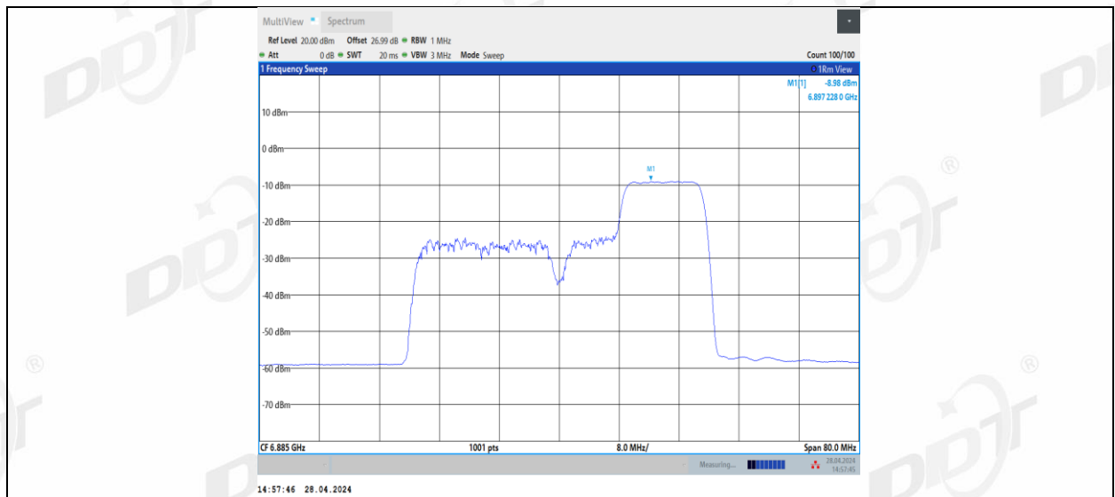
11BE40MIMO_Ant3_6885_106+26_3
