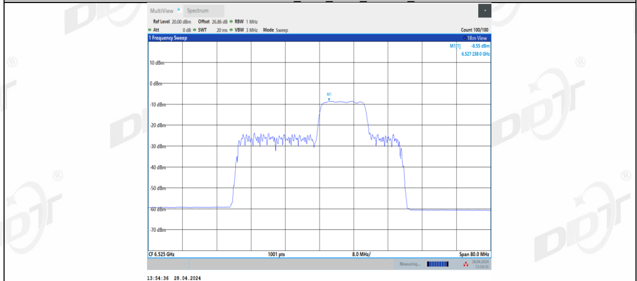
11BE40MIMO_Ant2_6525_106+26_4
