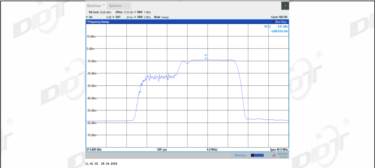
11BE20MIMO_Ant3_6895_52+26_1
