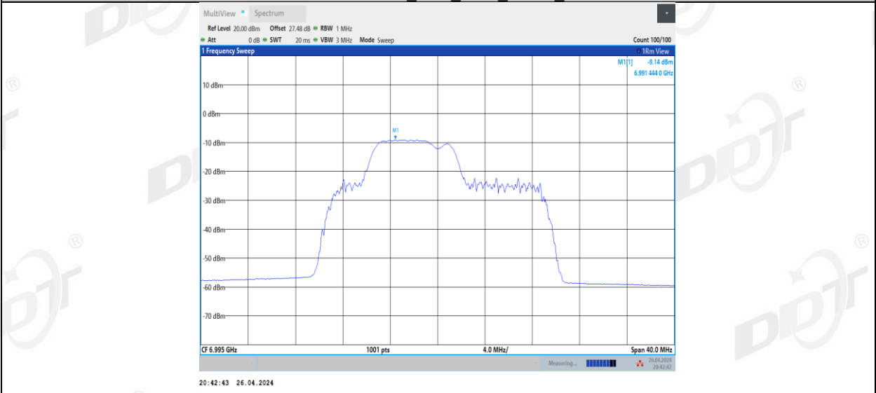
11BE20MIMO_Ant3_6995_52+26_3
