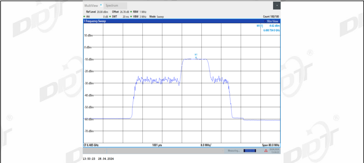
11BE40MIMO_Ant1_6485_106+26_4
