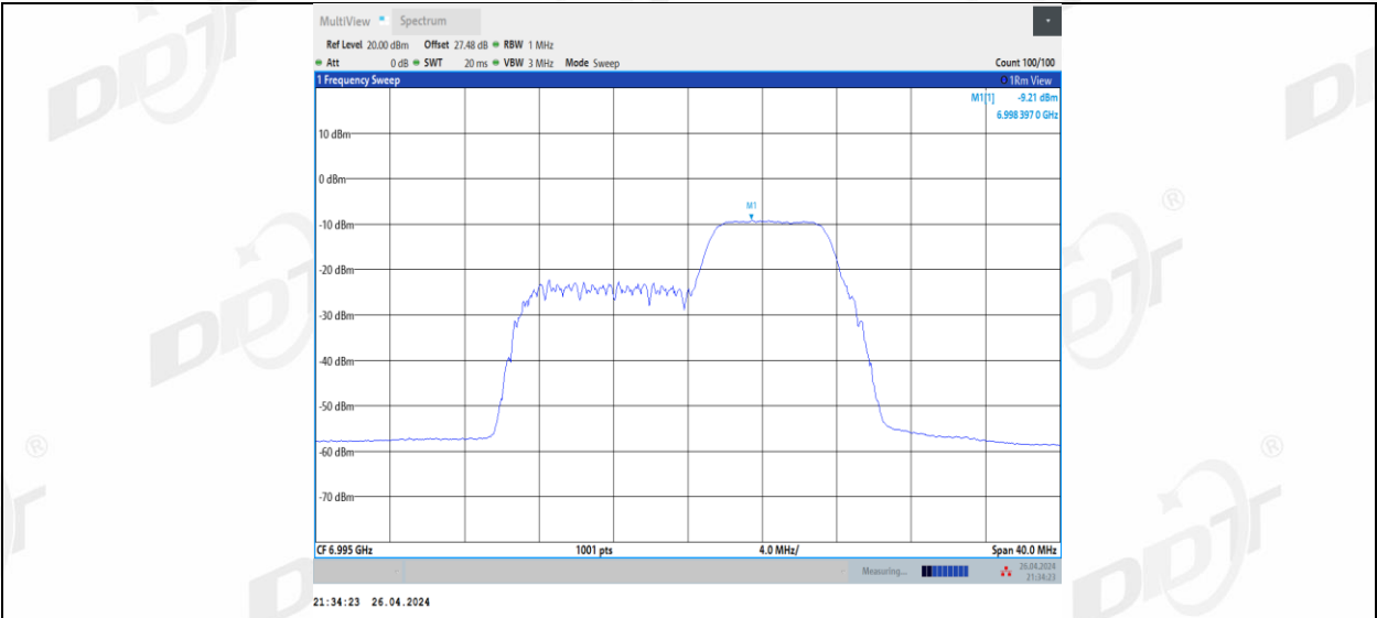
11BE20MIMO_Ant3_6995_106+26_1
