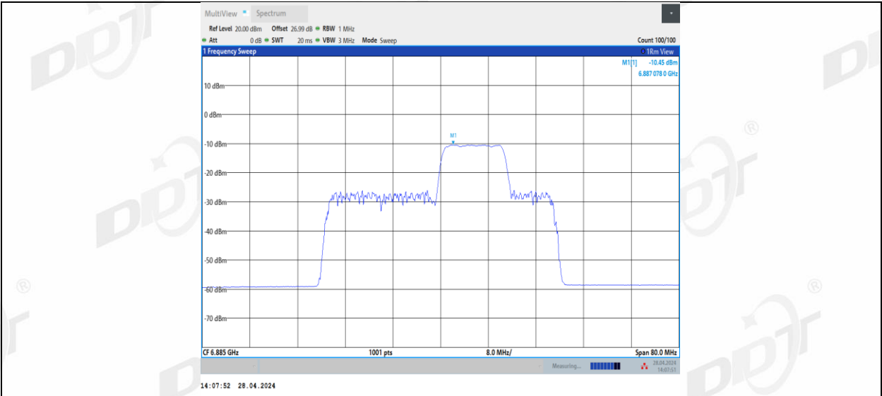
11BE40MIMO_Ant1_6885_106+26_4
