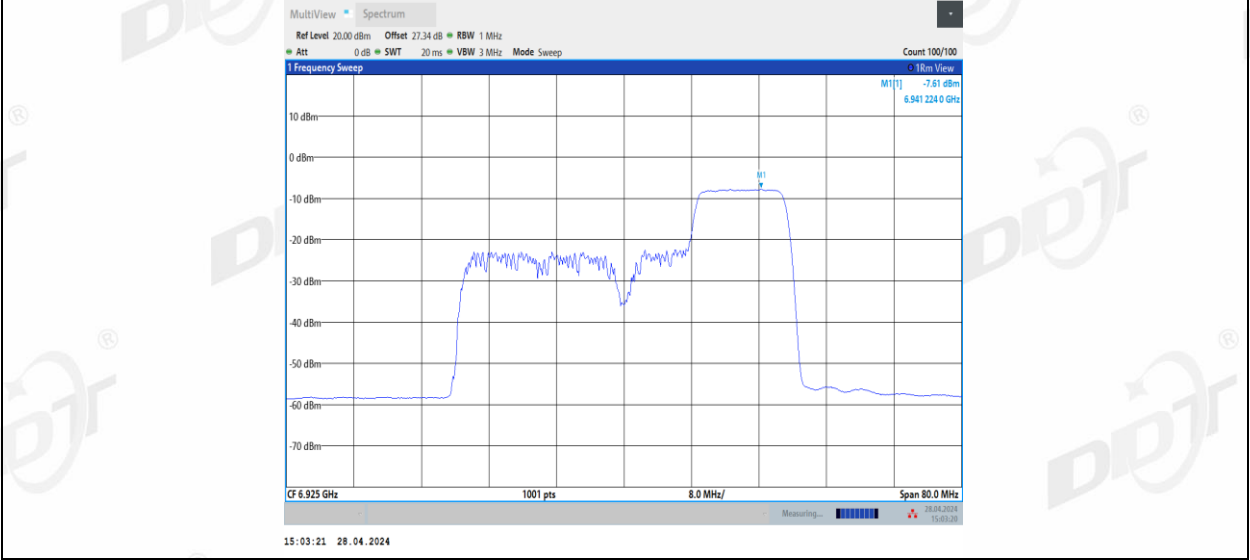
11BE40MIMO_Ant1_6965_106+26_3
