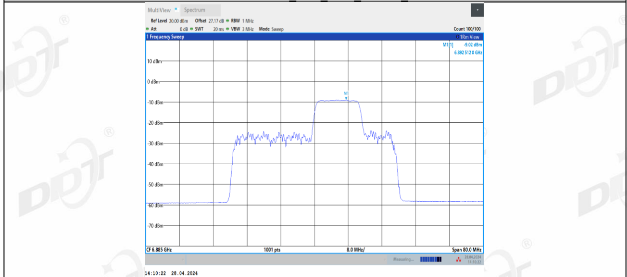
11BE40MIMO_Ant3_6885_106+26_4
