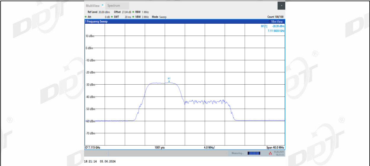
11BE20MIMO_Ant1_7115_52+26_2
