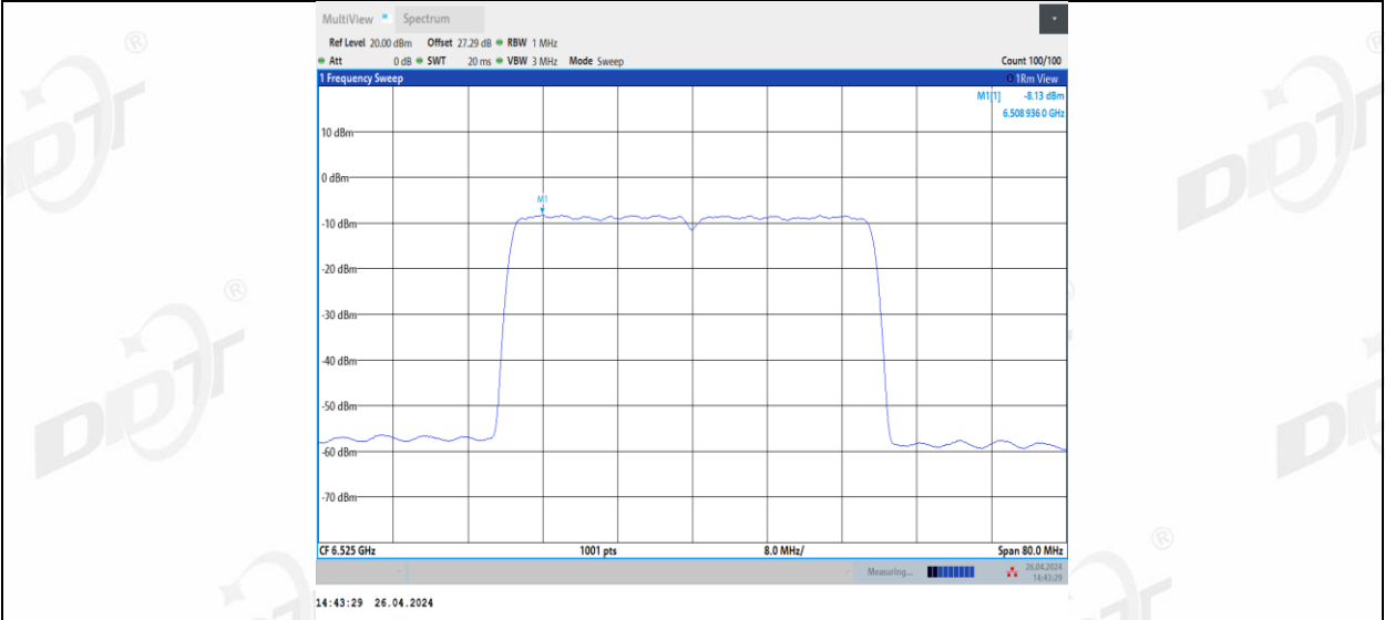
11BE40MIMO_Ant3_6525
