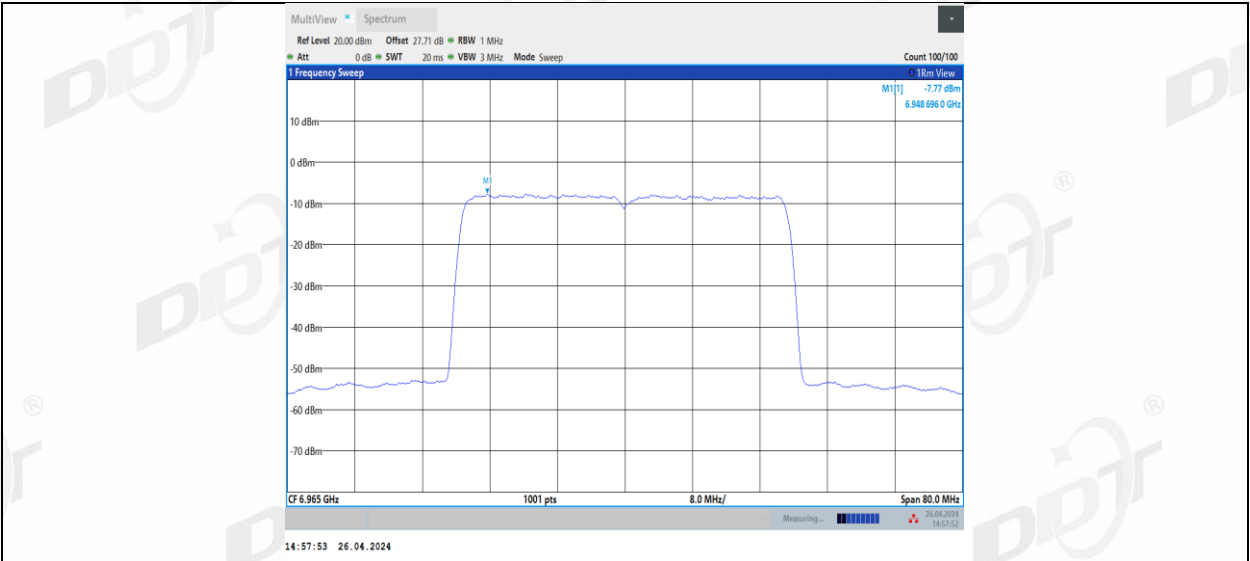
11BE40MIMO_Ant2_6965
