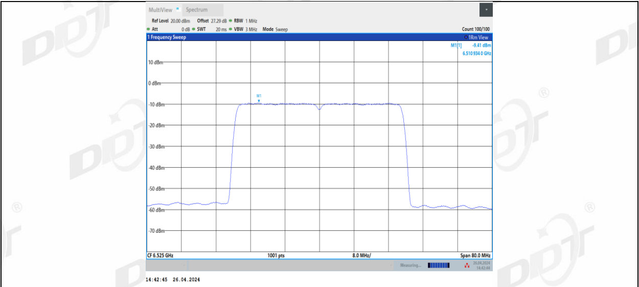
11BE40MIMO_Ant2_6525
