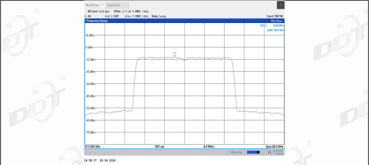
11BE40MIMO_Ant3_6965
