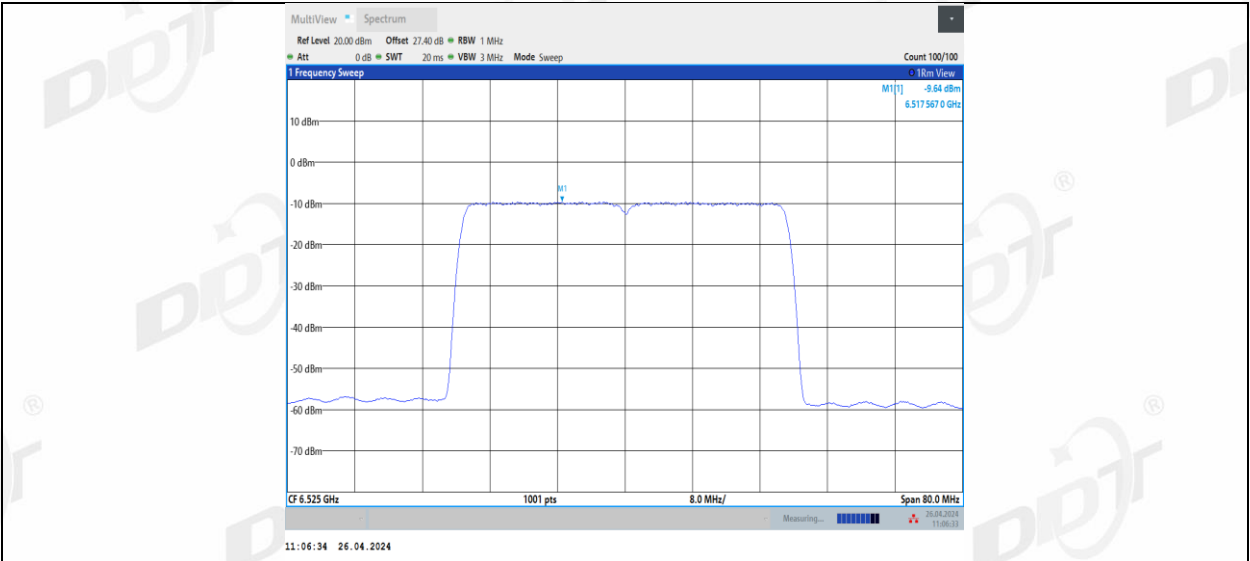
11AX40MIMO_Ant2_6525
