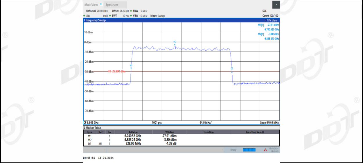
11BE320MIMO_Ant3_6905
