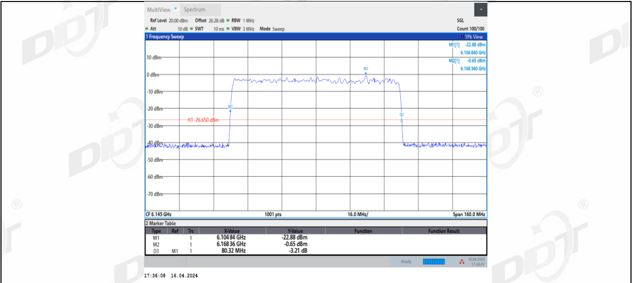
11BE80MIMO_Ant2_6145
