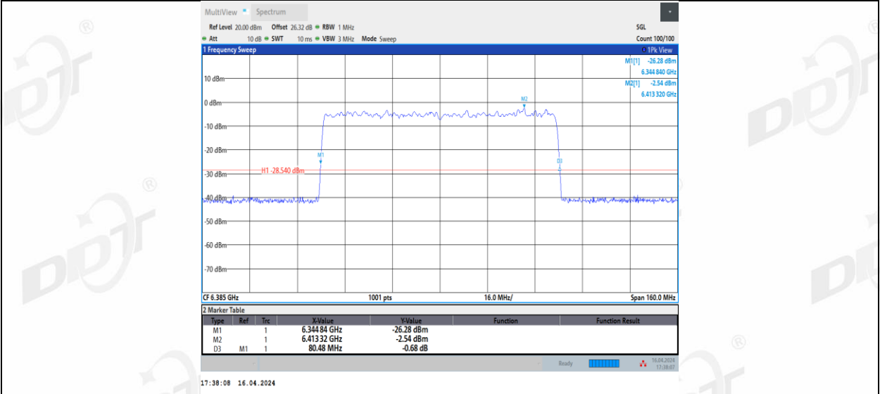
11BE80MIMO_Ant3_6385
