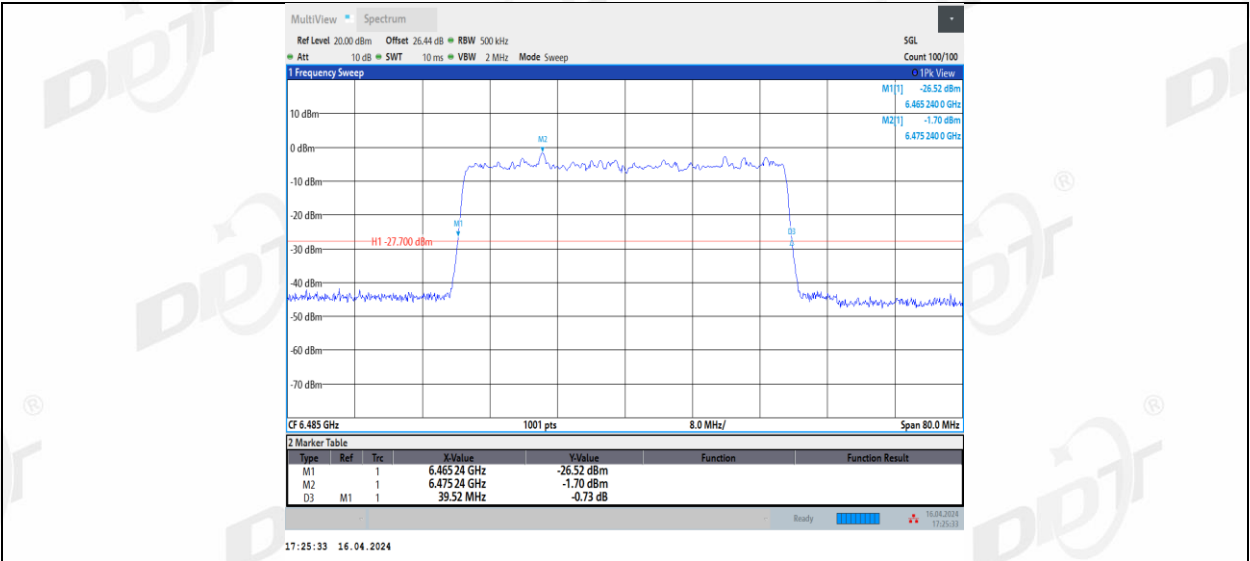
11BE40MIMO_Ant2_6485
