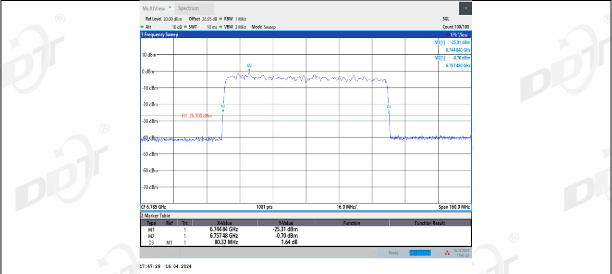
11BE80MIMO_Ant3_6785
