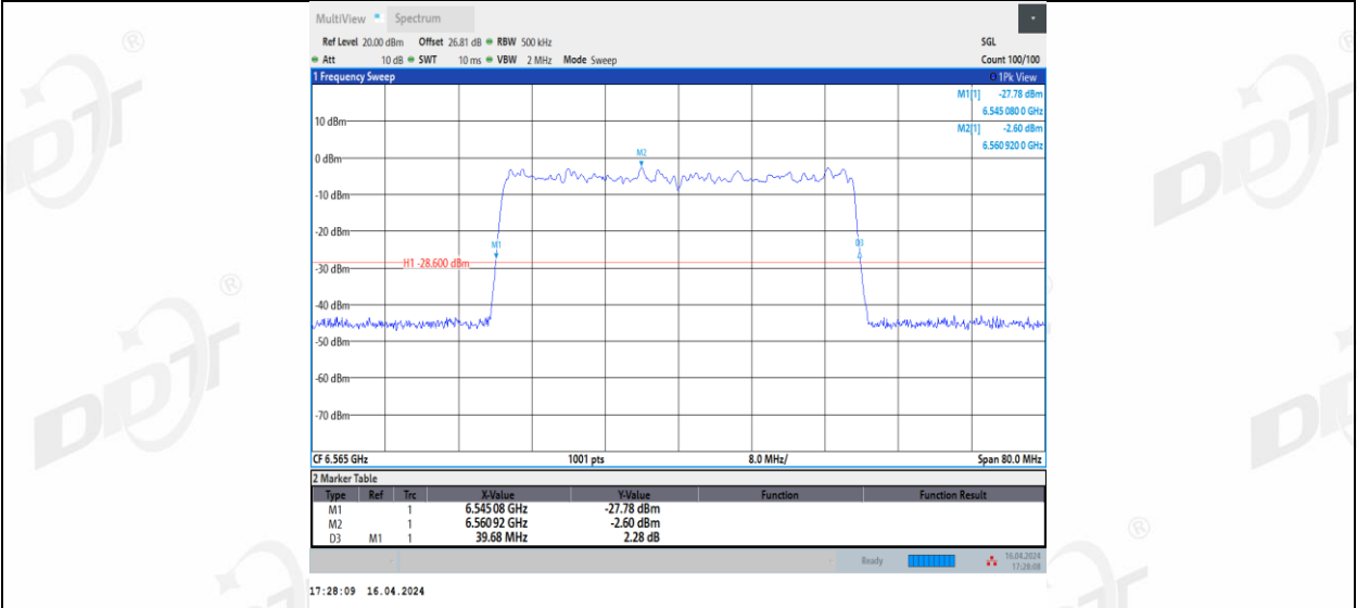
11BE40MIMO_Ant3_6565
