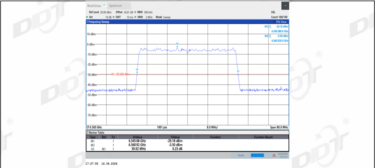
11BE40MIMO_Ant2_6565
