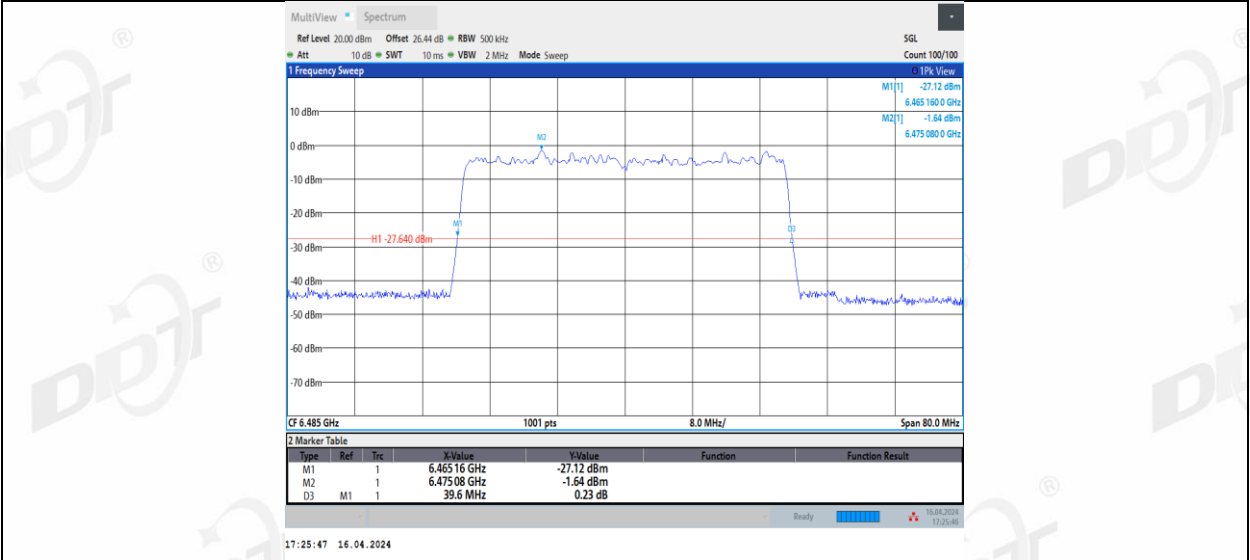
11BE40MIMO_Ant3_6485
