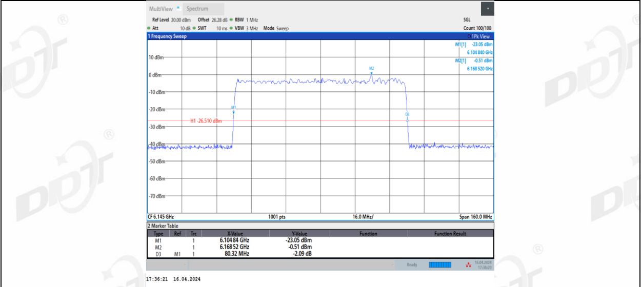
11BE80MIMO_Ant3_6145
