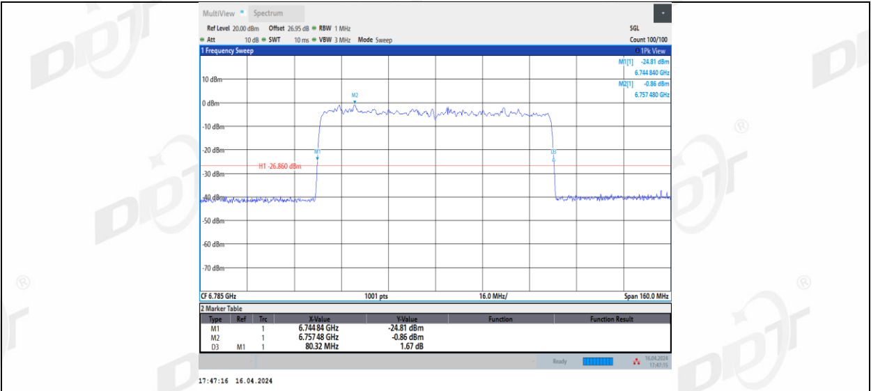
11BE80MIMO_Ant2_6785
