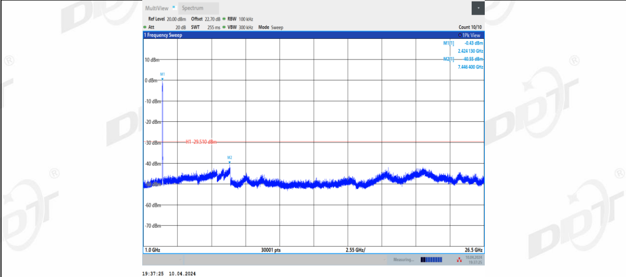
11AX40MIMO_Ant2_2422_0~Reference
