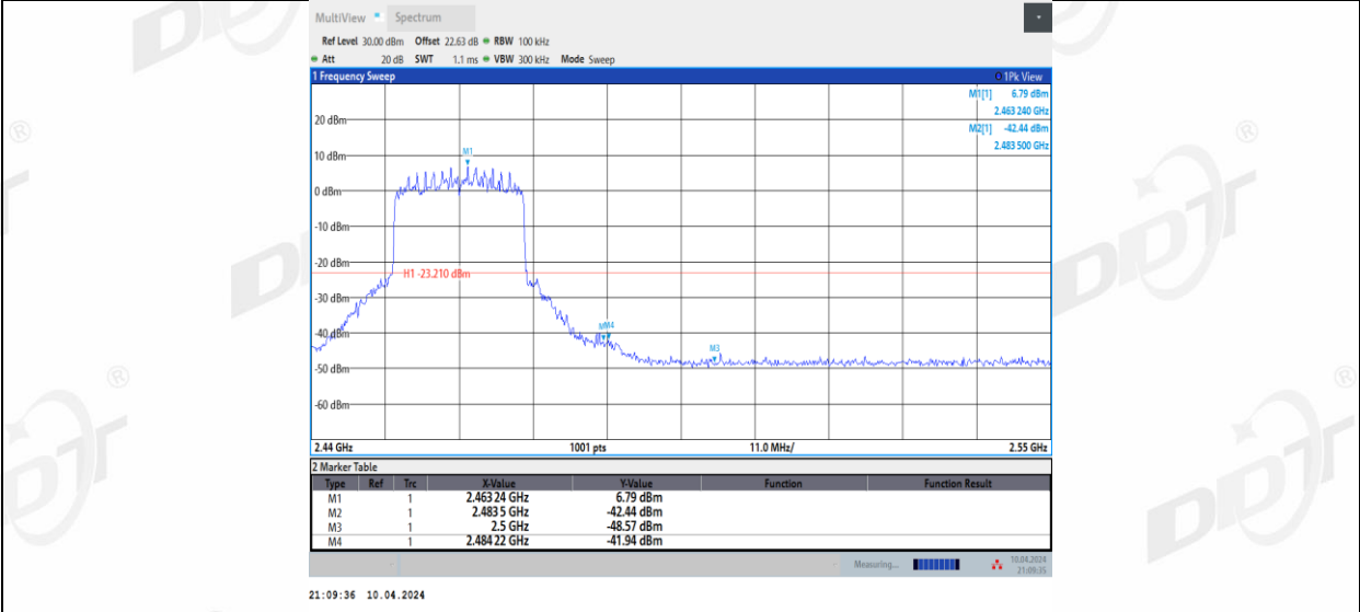
11BE20MIMO_Ant2_High_2462
