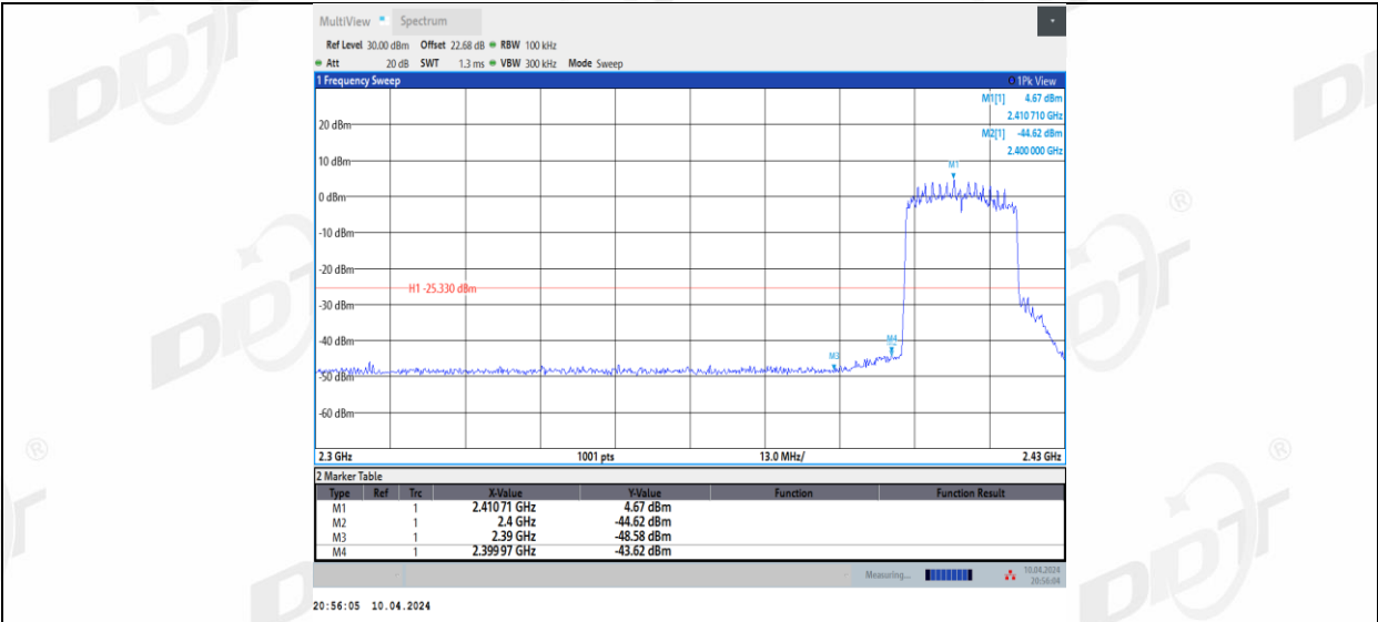
11BE20MIMO_Ant2_Low_2412
