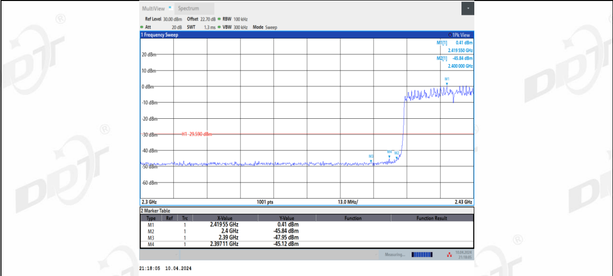
11BE40MIMO_Ant2_Low_2422
