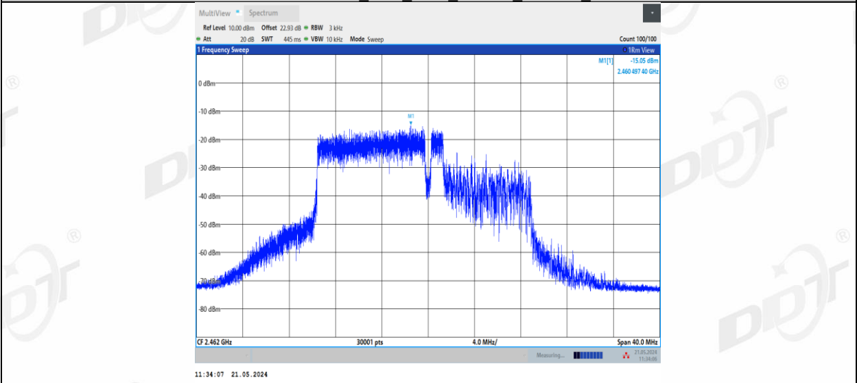
11BE20MIMO_Ant1_2462_106+26_OFDMA_2
