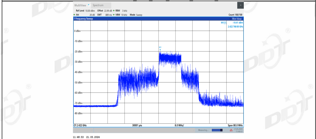
11BE40MIMO_Ant2_2422_106+26_OFDMA_4
