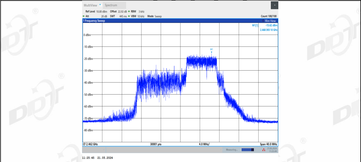
11BE20MIMO_Ant1_2462_106+26_OFDMA_1
