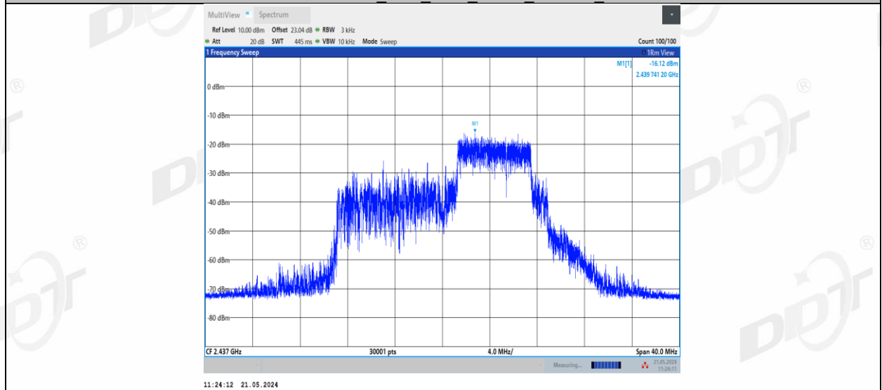
11BE20MIMO_Ant2_2437_106+26_OFDMA_1
