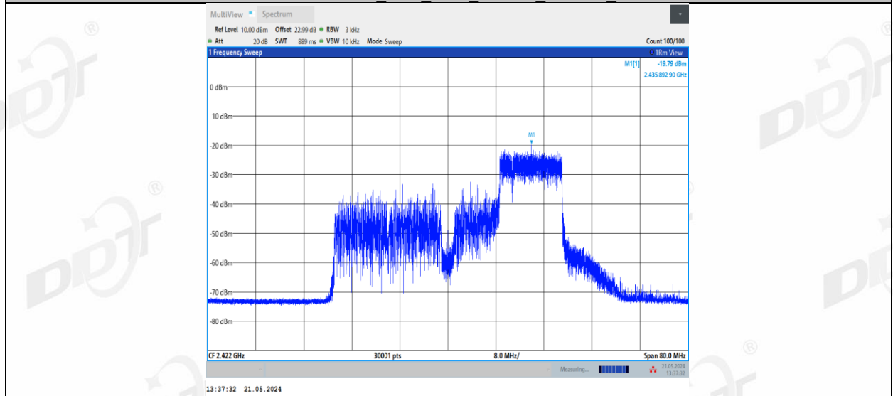
11BE40MIMO_Ant2_2422_106+26_OFDMA_3
