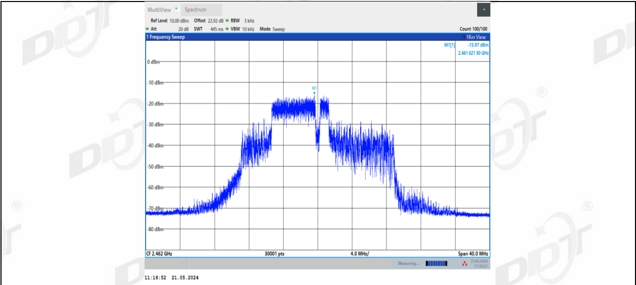
11BE20MIMO_Ant1_2462_52+26_OFDMA_3
