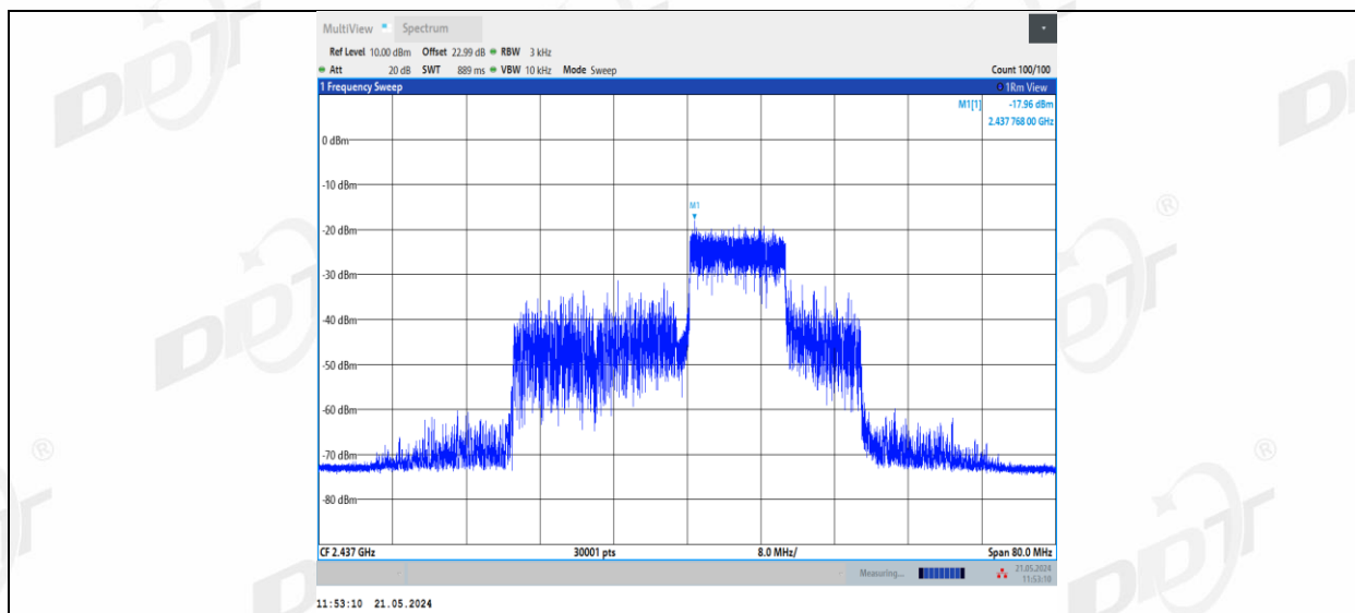
11BE40MIMO_Ant2_2437_106+26_OFDMA_4
