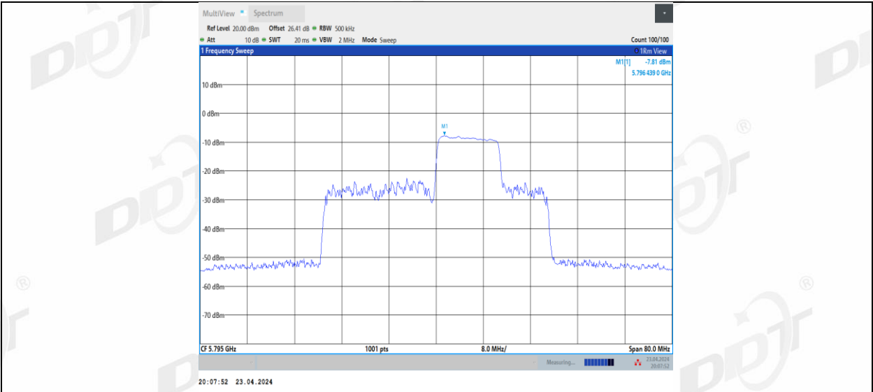
11BE40MIMO_Ant1_5795_106+26_4
