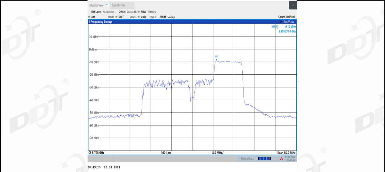
11BE40MIMO_Ant2_5795_106+26_3
