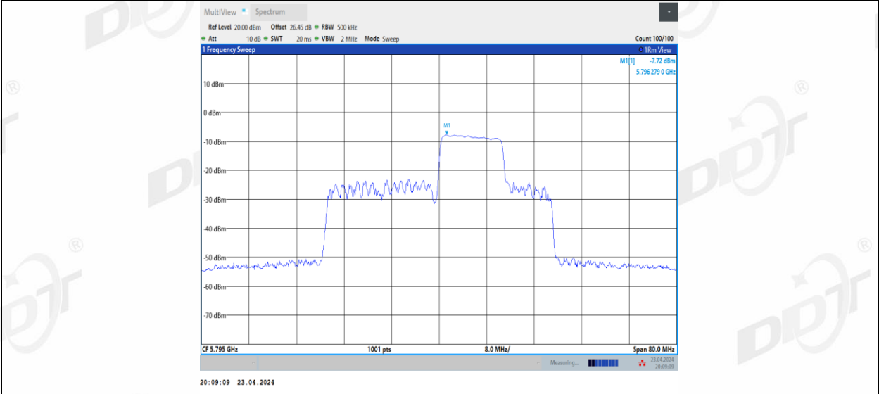
11BE40MIMO_Ant2_5795_106+26_4
