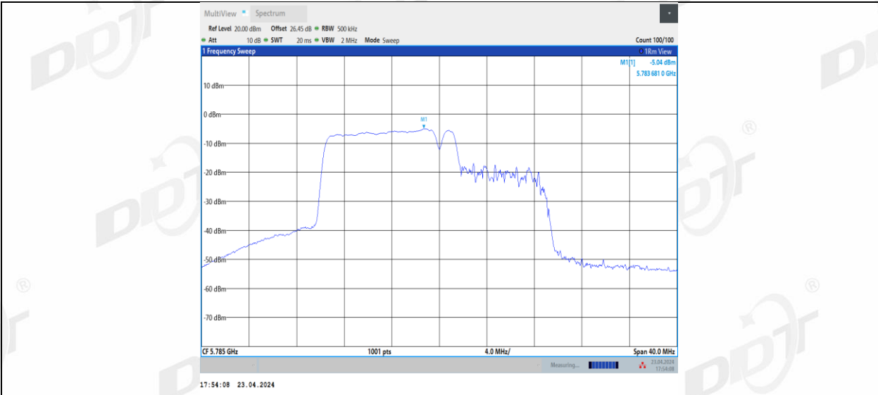
11BE20MIMO_Ant1_5785_106+26_2
