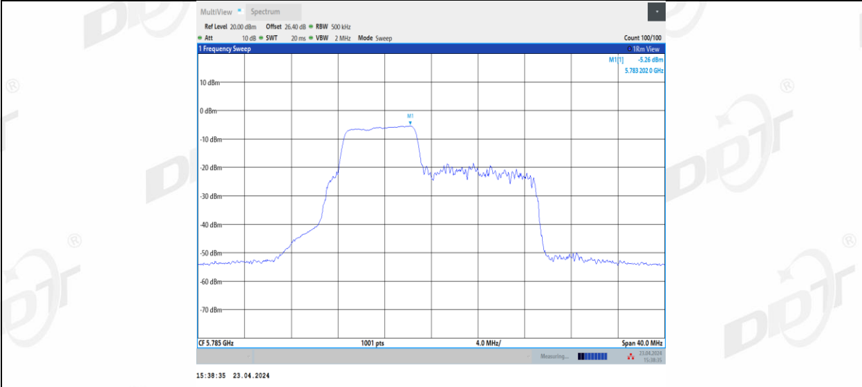
11BE20MIMO_Ant2_5785_52+26_2
