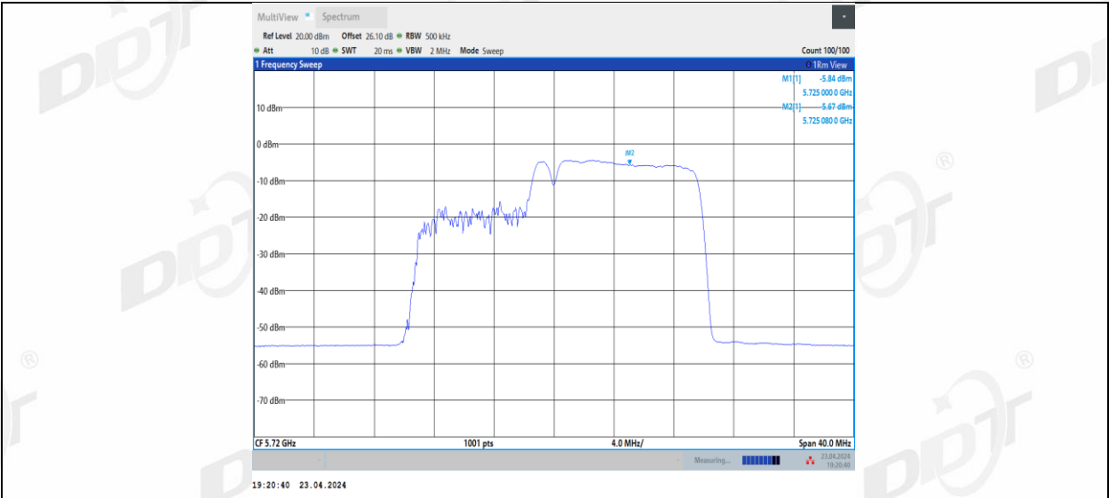
11BE20MIMO_Ant3_5720_UNII-3_52+26_1
