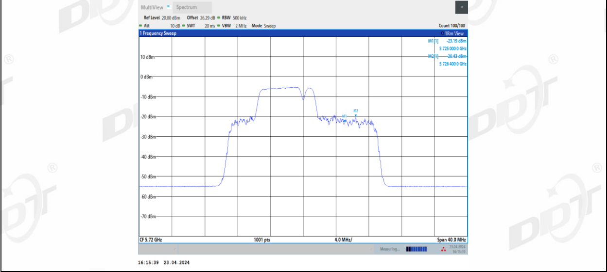
11BE20MIMO_Ant3_5720_UNII-3_52+26_3
