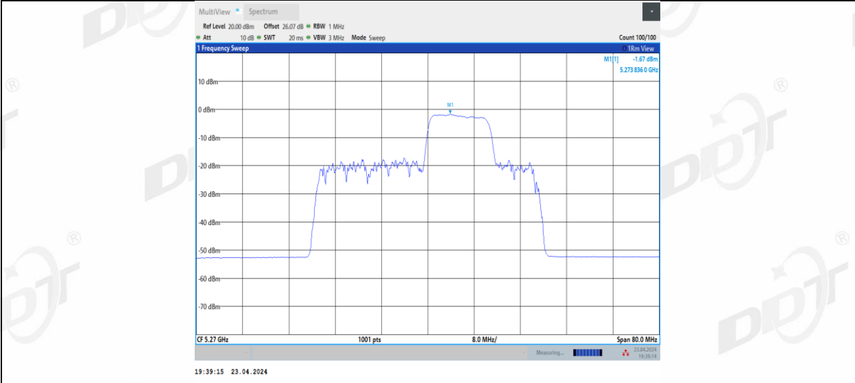
11BE40MIMO_Ant2_5270_106+26_4
