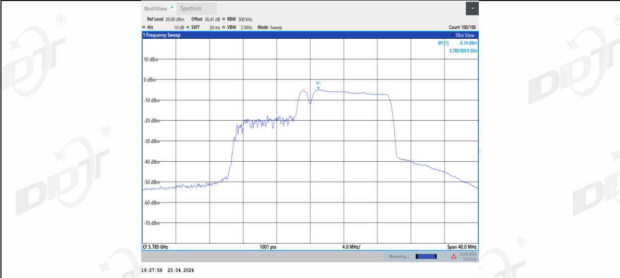
11BE20MIMO_Ant2_5785_52+26_1
