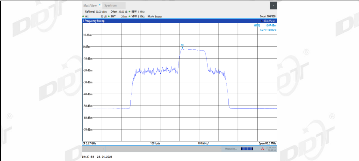
11BE40MIMO_Ant1_5270_106+26_4
