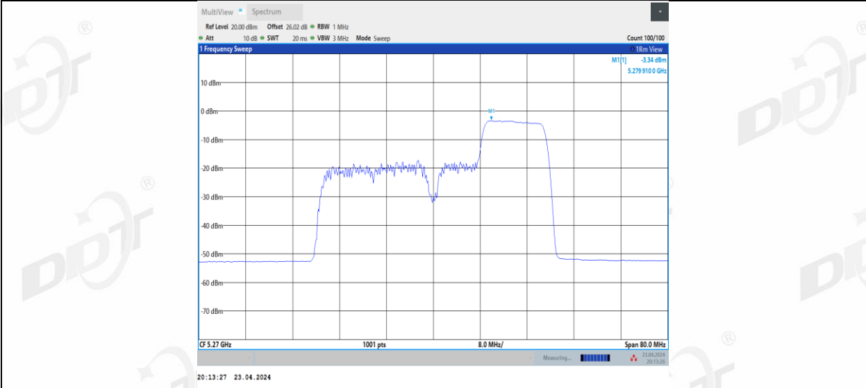
11BE40MIMO_Ant2_5270_106+26_3
