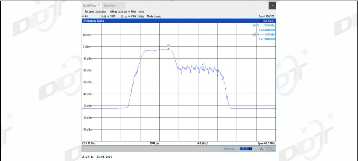
11BE20MIMO Ant1 5720 UNII-2C 52+26 2
