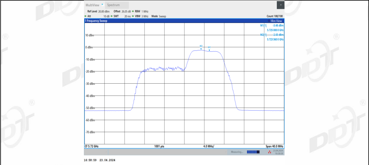
11BE20MIMO Ant1 5720 UNII-2C 106+26 1
