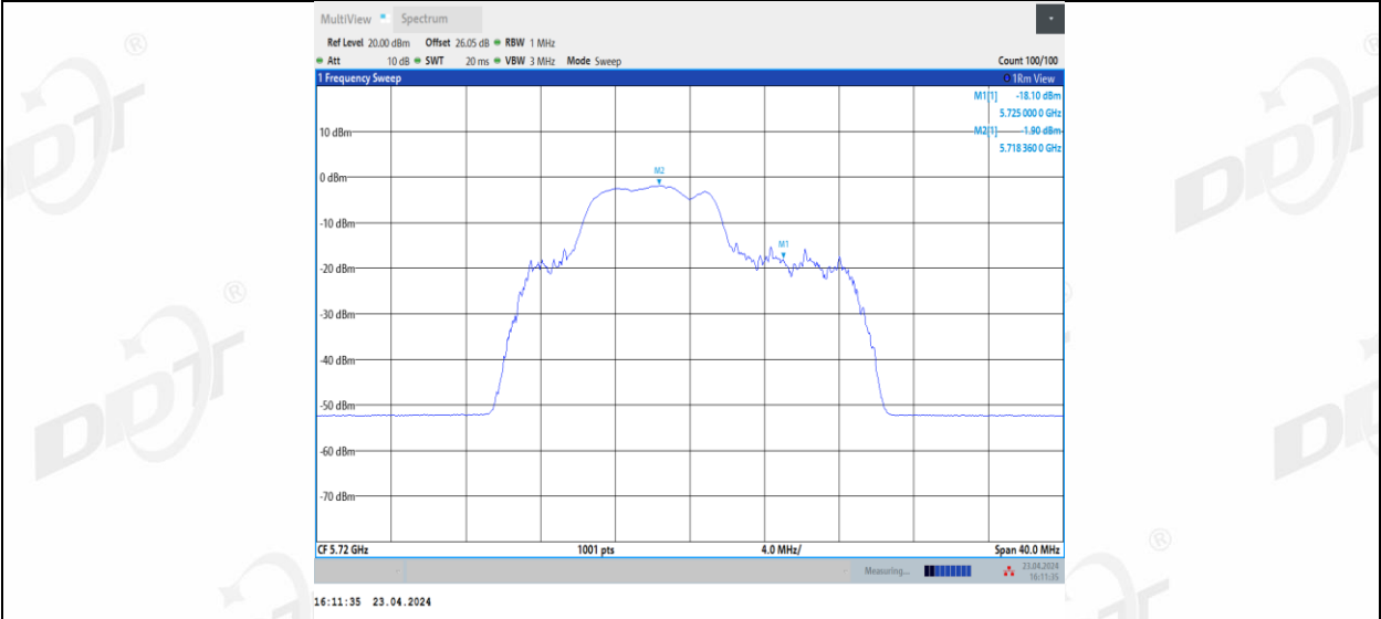
11BE20MIMO Ant1 5720 UNII-2C 52+26 3
